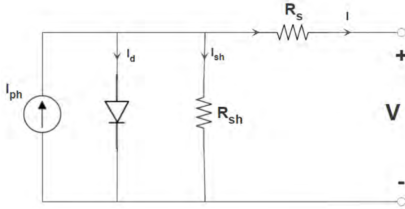
Figure 6 Modèle 1-diode équivalent.
