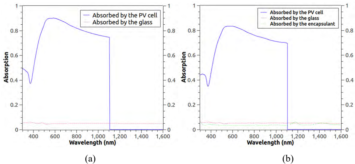
Figure 5 Pourcentage des photons absorbés par les couches du panneau photovoltaïque en fonction de la longueur d'onde pour les panneaux : BP 350 et BP 585(a) et VSMS275 (b).
