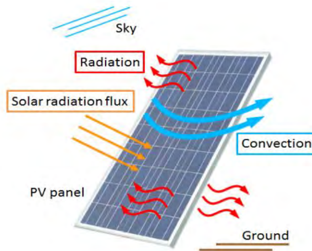
Figure 3 Représentation des échanges thermiques avec l'environnement du panneau.
