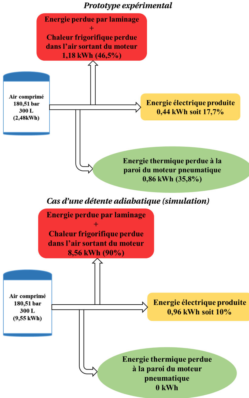
FIGURE 3.21 : Diagramme de répartition de l'énergie pendant la phase de décharge des bouteilles ; cas du prototype expérimental (à gauche) et cas d'un système où la détente de l'air dans le moteur pneumatique se ferait de façon adiabatique (à droite)
