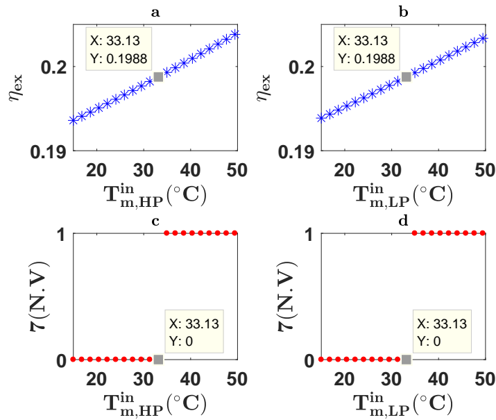
FIGURE 4.17 : Effet de la variation de la température de l'air à l'entrée de l'étage haute puissance (a&c) et basse puissance (b&d) du moteur pneumatique sur le rendement exergetique global et sur la violation des contraintes au point optimal.
