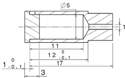
FIGURE E.5 – Schéma de la géométrie du creuset (dimension en millimètre).
