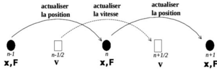
FIGURE 2.14 – Schéma de propagation en Leap Frog
