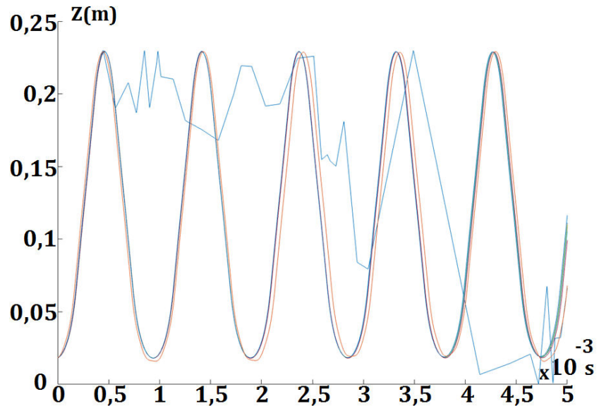
FIGURE C.4 – Évolution de la coordonnée z d'une particule de propagation dans une source d'ions avec différents pas de temps. Les pas de temps affichés vont de 2 \times 10^{-11} \text{s} à 5 \times 10^{-5} \text{s} .
