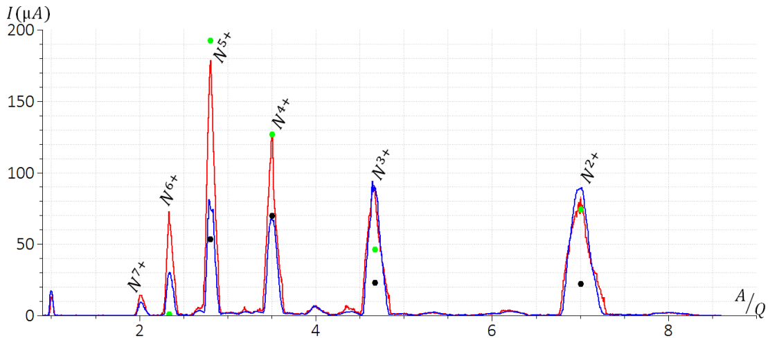
FIGURE D.7 – Spectre d'ions pour un plasma d'azote à 500 W avec GTS. Les spectres expérimentaux sont obtenus en présence d'un confinement magnétique tel que B_{inj} = 1,65 T , B_{med} = 0,29 T et B_{ext} = 0,85 T sur l'axe de la chambre. Dans les deux cas (avec et sans l'utilisation du disque polarisé), la pression à l'injection est de P_{inj} = 6,8 \times 10^{-7} mbar .
