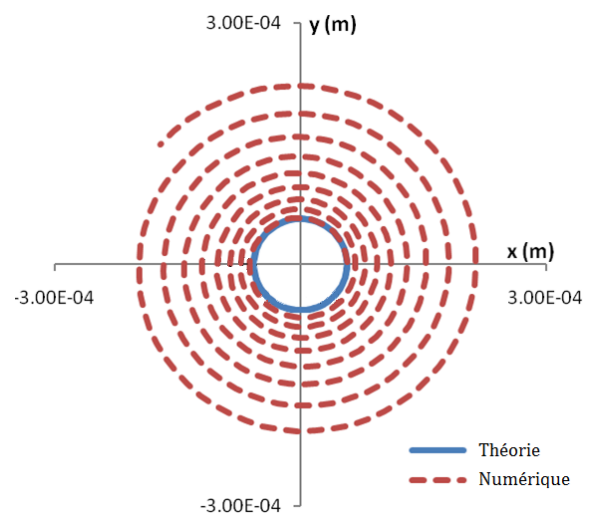
FIGURE 2.15 – Propagation d'une particule chargée dans une champ magnétique par la méthode du "Leap Frog" [89]
