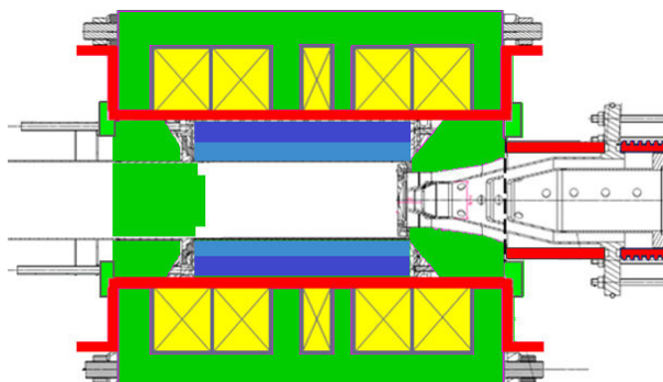
FIGURE 3.1 – La source d'ions PHOENIX V3 est une source d'ions RCE. Son confinement magnétique est produit par trois solénoïdes (représentés en jaune) et un hexapôle (en bleu).
