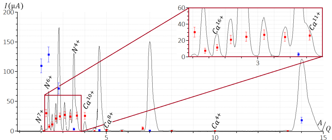
FIGURE 5.3 – Spectre d'ions Ca obtenu avec la simulation CHIMERE (en optimisant les courants d'ions Ca ) avec des énergies moyennes pour les électrons froids E_{out} = 10 eV , E_{in} = 350 eV pour les électrons tièdes et E_{hot} = 400 eV pour les électrons chauds. Les valeurs de puits de potentiels et de potentiel plasma sont respectivement Pot_{Dip} = 0,39 V et Pot_{plasma} = 0 V . Les points bleus représentent les courants des ions N et les points rouges les courants des ions Ca .
