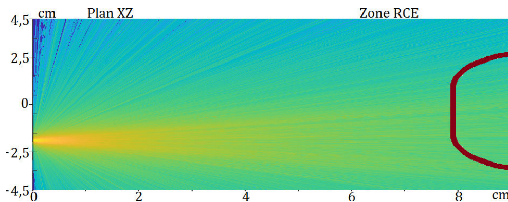
FIGURE 4.11 – Représentation de la densité de particules en échelle logarithmique entre le creuset ( z = 0 \text{ cm} ) et la zone RCE ( z = 8 \text{ cm} ) dans le plan XZ.
