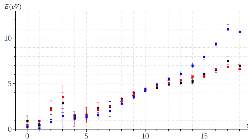
FIGURE 3.19 – Distribution en énergie moyenne des différents états de charge présents dans le plasma de la source d'ions RCE, en noir les valeurs de référence, en rouge les valeurs avec la distance maximale à 10 \mu\text{m} et en bleu à 10 \text{nm} . Les énergies moyennes des particules dans le plasma sont respectivement de 3,54 \pm 0,12 \text{eV} , 3,40 \pm 0,12 \text{eV} et 2,32 \pm 0,08 \text{eV} .
