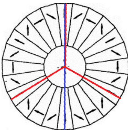
FIGURE 2.1 – Schéma en coupe d'un hexapôle. Chaque flèche indique la polarisation Nord-Sud de l'aimant permanent, l'ensemble produit un champ de type Halbach. La ligne bleue délimite une moitié d'hexapôle et la rouge un tiers d'hexapôle
