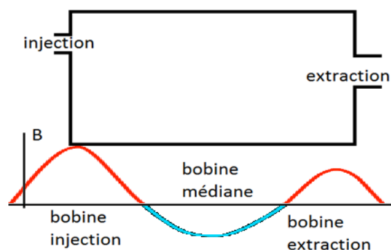
FIGURE 2.2 – Schéma de l'enceinte de la source, et des champs magnétique des solénoïdes
