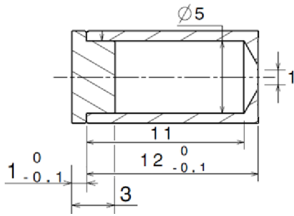
FIGURE E.3 – Schéma de la géométrie du creuset (dimension en millimètre).
