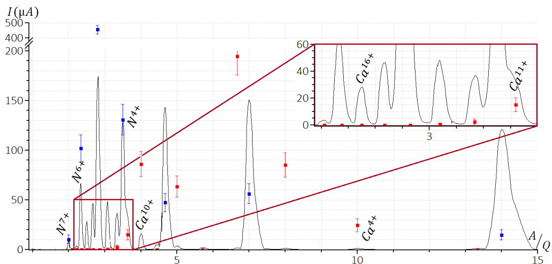
FIGURE 5.1 – Spectre d'ions calcium obtenu avec la simulation CHIMERE avec des énergies moyennes pour les électrons froids E_{out} = 90 \text{ eV} , E_{in} = 40 \text{ eV} pour les électrons tièdes et E_{hot} = 285 \text{ eV} pour les électrons chauds. Les valeurs de puits de potentiels et de potentiel plasma sont respectivement à Pot_{Dip} = 0,07 \text{ V} et Pot_{plasma} = 60 \text{ V} . Les points bleus représentent les courants des ions N et les points rouges les courants des ions Ca .
