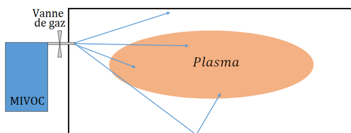
FIGURE 1.20 – Schéma d'utilisation de la méthode MIVOC pour la production d'ions métalliques.
