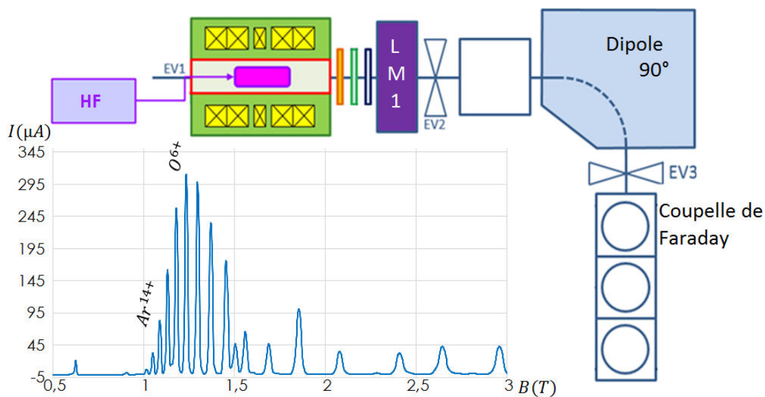
FIGURE 3.2 – La ligne d'analyse basse énergie associée à la source d'ions PHOENIX V3 est constituée d'une lentille magnétique, d'un dipôle magnétique et de diagnostics faisceaux. Un spectre d'ions \text{Ar} (avec oxygène comme gaz support) typique produit par la source et mesuré par cette ligne d'analyse est affiché sous le synoptique de la ligne.
