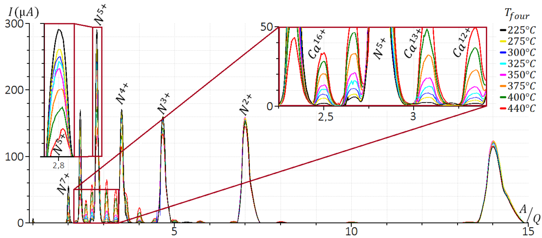
FIGURE 4.27 – Spectres d'ions Ca obtenus avec la source d'ions PHOENIX V3. Les différents spectres d'ions ont été obtenus pour une puissance micro-onde injectée dans la chambre à plasma de 1900\text{ W} , une différence de potentiel de 40\text{ kV} , et différentes températures de four. Le confinement magnétique est tel que B_{inj} = 1,50\text{ T} , B_{med} = 0,43\text{ T} et B_{ext} = 1,10\text{ T} sur l'axe de la chambre à plasma, et la pression à l'injection est de P_{inj} = 3,7 \pm 0,1 \times 10^{-8}\text{ mbar} , pour tous les spectres d'ions. Pour l'ensemble des spectres d'ions, la tension du disque de polarisation est flottante.
