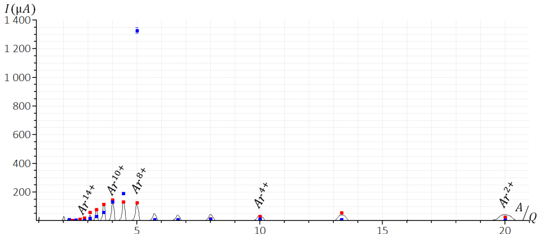
FIGURE 3.12 – Spectre d'ions présenté sur la figure 3.9 en rouge. Le spectre d'ions supplémentaire (en bleu) est issu de la simulation. Il est obtenu en initialisant la simulation avec les mêmes paramètres que précédemment à l'exception de l'énergie moyenne des électrons froids (fixée à 10^{-6}\text{ eV} au lieu de 5\text{ eV} ).
