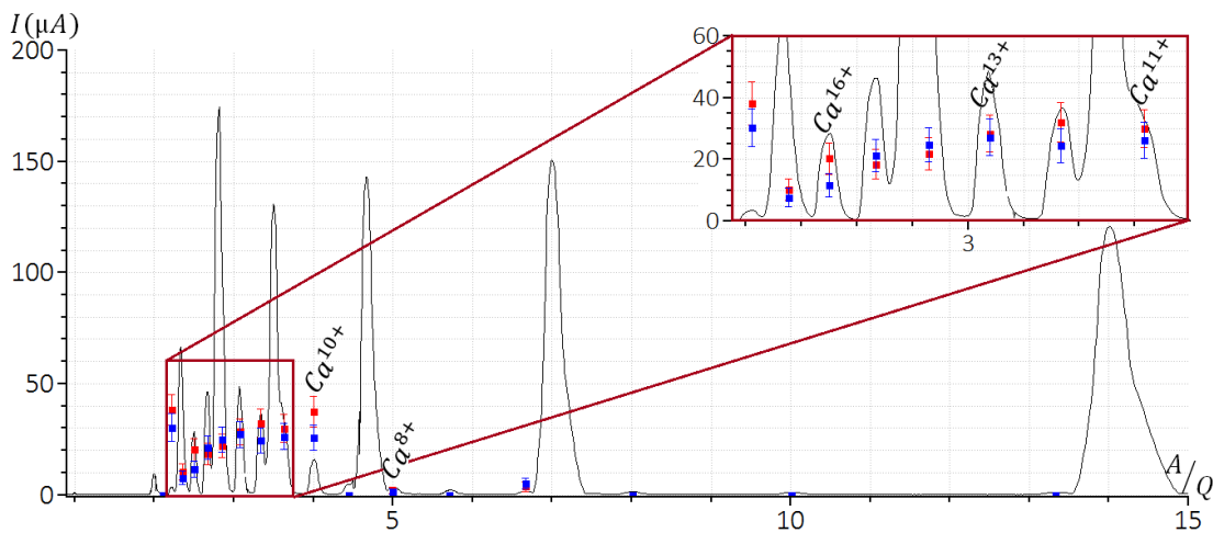
FIGURE 5.11 – Spectre d'ions Ca obtenu avec la simulation CHIMERE avec des énergies moyennes pour les électrons froids E_{out} = 5 \text{ eV} , E_{in} = 450 \text{ eV} pour les électrons tièdes et E_{hot} = 450 \text{ eV} pour les électrons chauds. Les valeurs du puits de potentiel et potentiel plasma sont respectivement à Pot_{Dip} = 0,41 \text{ V} et Pot_{plasma} = 0 \text{ V} . Les points bleus correspondent au spectre pour une chambre avec un diamètre interne de 89 mm; les points rouges pour une chambre avec un diamètre interne de 80 mm (seuls les points correspondants aux courants d'ions calcium sont représentés).
