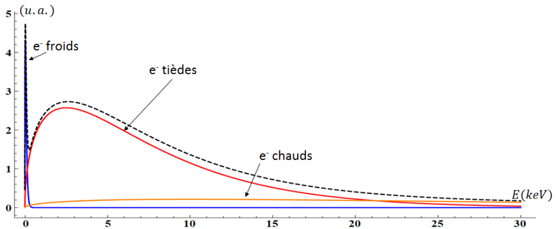
FIGURE 1.14 – Distribution qualitative des différentes populations d'électrons en fonction de l'énergie. Les fonctions de distributions maxwelliennes en énergie des électrons sont représentées: en bleu pour les électrons froids; en rouge, pour les électrons tièdes; et en orange pour les électrons chauds. La courbe en pointillés définit le contour de la distribution globale des électrons.
