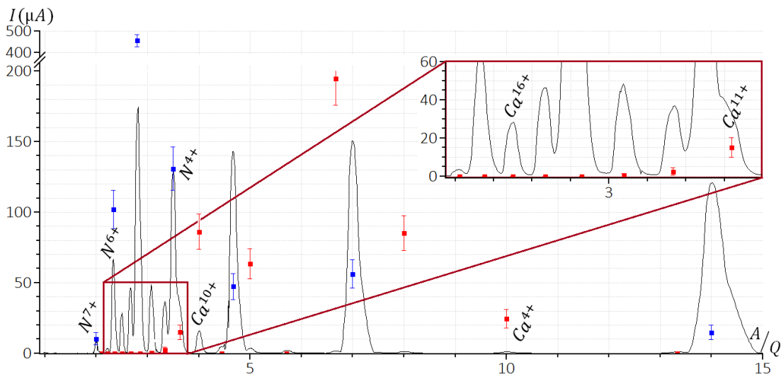
FIGURE 5.2 – Spectre d'ions calcium obtenu avec la simulation CHIMERE (en optimisant les courants d'ions N ) avec des énergies moyennes pour les électrons froids E_{\text{out}} = 40 \text{ eV} , E_{\text{in}} = 90 \text{ eV} pour les électrons tièdes et E_{\text{hot}} = 295 \text{ eV} pour les électrons chauds. Les valeurs de puits de potentiels et de potentiel plasma sont respectivement à Pot_{\text{Dip}} = 0,07 \text{ V} et Pot_{\text{plasma}} = 40 \text{ V} . Les points bleus représentent les courants des ions N et les points rouges les courants des ions Ca .
