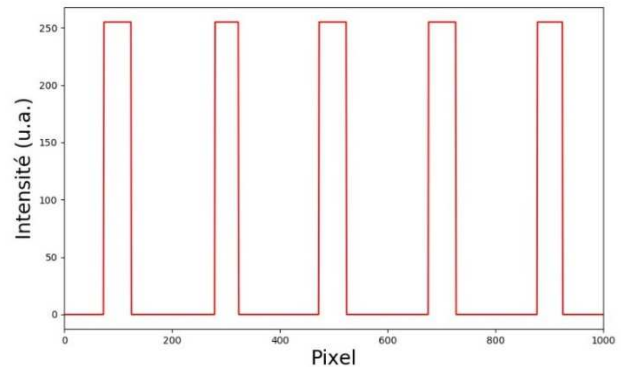
Figure IV.18 : Signal obtenu sur une coupe horizontale d'un échantillon virtuel (binaire).
