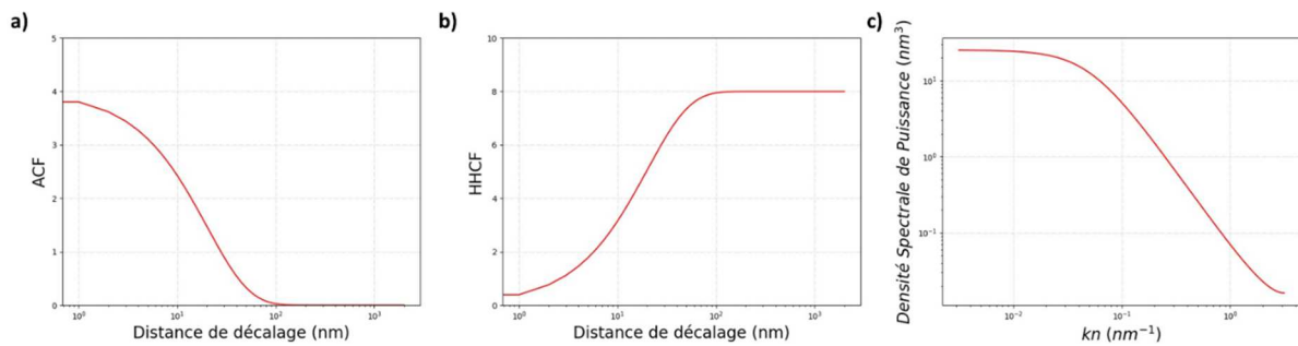
Figure II.8 : Représentation des différents modèles liés à la rugosité, d'un cas de paramétrage identique ( \sigma = 2 nm, \alpha = 0.5 , \xi = 20 nm), a) ACF (AutoCorrelation Function), b) HHCF (Heigh-Heigh Correlation Function), c) PSD (Power Spectral Density).
