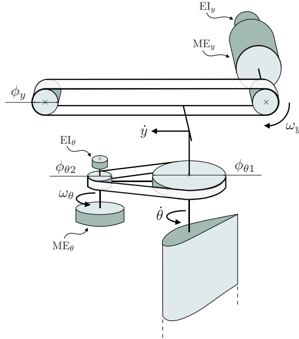
FIGURE 3.6 – Systèmes de conversion des mouvements de pilonnement et de tangage en mouvements de rotation.
