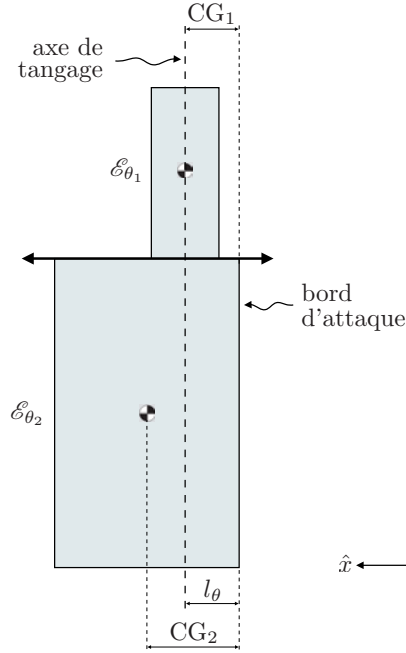
FIGURE 3.14 – Subdivision de l'ensemble \mathcal{E}_{\theta} d'éléments impliqués dans le mouvement de tangage en deux groupes : \mathcal{E}_{\theta_1} , dont le centre de gravité est supposé sur l'axe de tangage, et \mathcal{E}_{\theta_2} , dont la distance à l'axe de tangage est variable.
