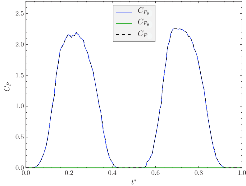
FIGURE 5.7 – Évolution des coefficients de puissance du système hydrolien sur une période d’oscillation de l’aile dans le cas optimal de la configuration C_2 .
