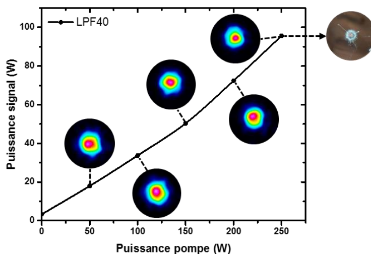
Figure IV-2 – Évolution de la puissance extraite en fonction de la puissance de pompe pour une LPF40 en régime d'amplification nanoseconde pour une puissance en entrée de fibre de 4,9 W environ. En insert sont reportées les distributions d'intensité du faisceau en champ lointain prises à plusieurs niveaux de puissances extraites ainsi qu'une photo de la face endommagée à puissance maximale.
