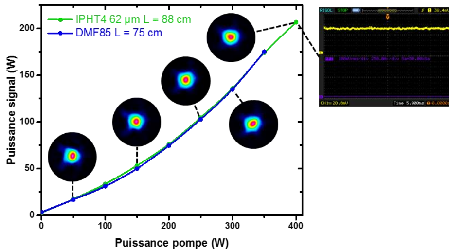
Figure IV-5 – Évolution de la puissance extraite en fonction de la puissance de pompe pour l'échantillon 1 IPHT 4 62 (FA-LPF de diamètre de champ de mode proche de 62\ \mu\text{m} et de \Delta n \approx 4.10^{-5} ) en régime d'amplification nanoseconde pour une puissance en entrée de FA-LPF de 4,9 W environ (courbe verte). La courbe en bleu donne la puissance extraite en fonction de la puissance de pompe en régime d'amplification nanoseconde pour une puissance en entrée de fibre de 4,9 W environ pour la DMF85 présentée en Figure IV-3. En insert sont reportées les distributions d'intensité du faisceau en champ lointain prises à plusieurs niveaux de puissances extraites ainsi qu'une trace temporelle acquise à la photodiode témoignant de l'absence du phénomène des instabilités modales transverses.
