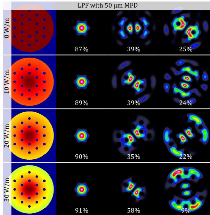
Figure II-6 – Représentation schématique de la structure LPF et modes calculés pour une LPF de 50 \mu\text{m} de diamètre de champ modal à 1030 \text{ nm} lorsque la charge thermique (exprimée en \text{W.m}^{-1} ) augmente. Le mode fondamental et les deux modes d'ordre supérieur les plus confinés sont étudiés. Pour chaque mode, un pourcentage est calculé correspondant au facteur de recouvrement du mode avec la zone de gain [STUTZKI 14].
