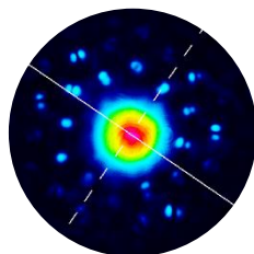
Figure IV-9 – Distribution d'intensité du faisceau en champ proche en sortie de DMF prise à la caméra WinCamD UCD12 à 50 mW de signal à 1030 nm injecté dans le cœur sans pomper la fibre.
