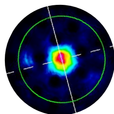
Figure IV-11 – Distribution d'intensité du faisceau en champ proche en sortie de FA-LPF prise à la caméra WinCamD UCD12 à 50 mW de signal à 1030 nm injecté dans le cœur sans pompage.
