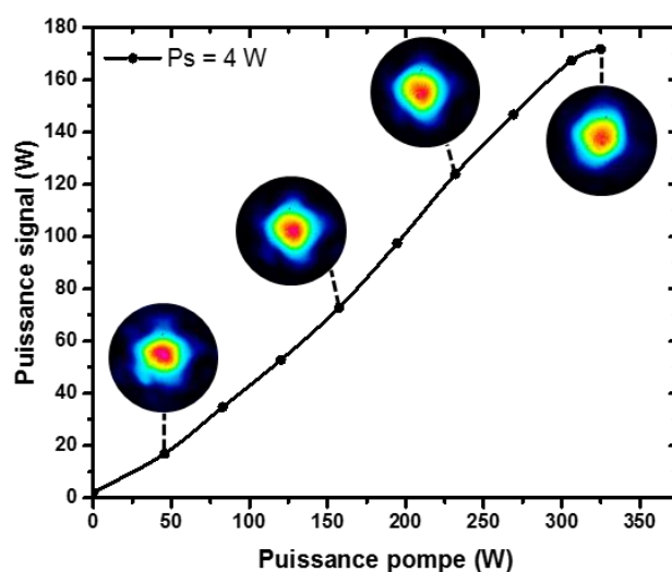
Figure IV-7 – Évolution de la puissance extraite en fonction de la puissance de pompe pour l'échantillon 2 Heraeus 1 68 (FA-LPF de diamètre de champ de mode proche de 68\ \mu\text{m} et de \Delta n \approx 8.10^{-5} ) en régime d'amplification picoseconde pour une puissance en entrée de FA-LPF de 4 W environ. En insert sont reportées les distributions d'intensité du faisceau en champ lointain prises à plusieurs niveaux de puissances extraites.
