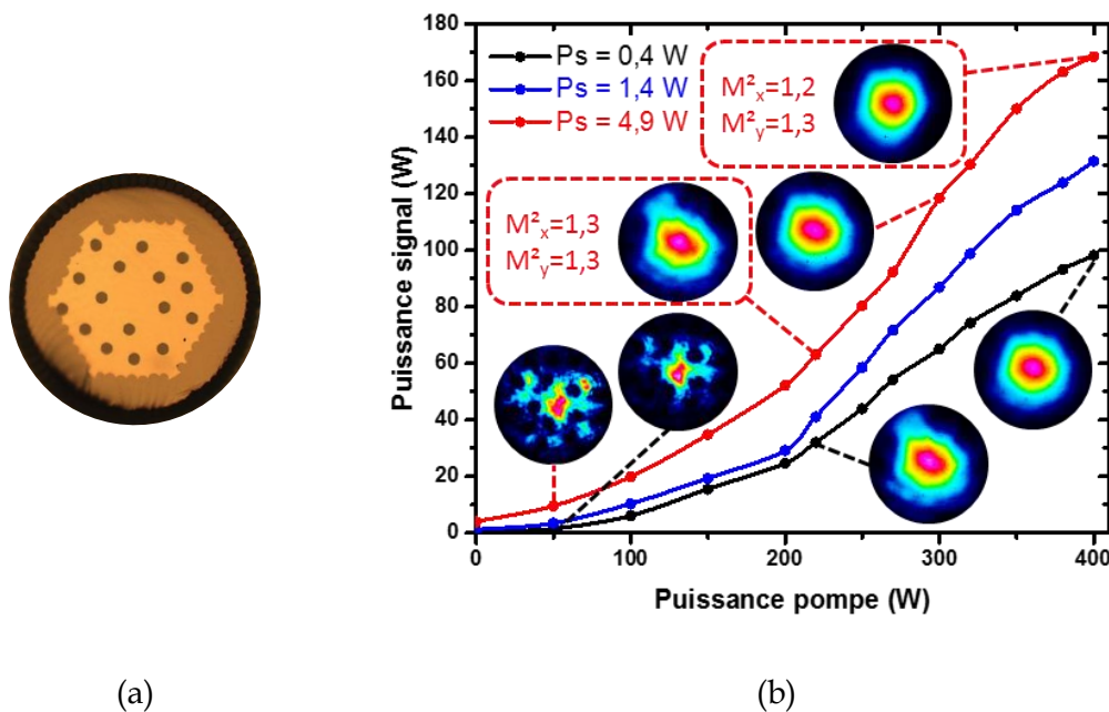
Figure V-8 – (a) Image de la face de la FA-LPF de diamètre de champ de mode environ égal à 92\ \mu\text{m} et de \Delta n \approx -3.10^{-5} prise au microscope ; (b) évolution de la puissance extraite en fonction de la puissance de pompe pour la FA-LPF sous test en régime d'amplification nanoseconde. En insert sont reportées les distributions d'intensité du faisceau correspondant au champ proche pour 50\ \text{W} de pompe et au champ lointain pour les valeurs supérieures.
