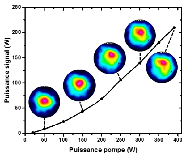
Figure III-10 – Évolution de la puissance extraite en fonction de la puissance de pompe pour la FA-LPF de \Delta n \approx +13.10^{-5} et un diamètre de cœur de 65\ \mu\text{m} . En insert sont reportées les distributions d'intensité du faisceau émis mesurées en champ lointain et prises à plusieurs niveaux de puissances extraites.
