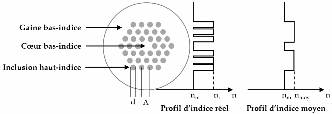
Figure II-7 – Section transverse et profils d'indice réel et moyen d'une fibre PCF à bande interdite photonique, avec n_m l'indice de réfraction du milieu, n_i l'indice de réfraction des inclusions et n_{moy} l'indice moyen de la gaine.
