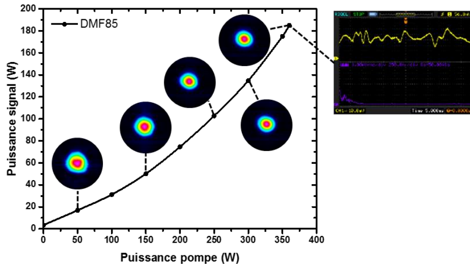
Figure IV-3 – Évolution de la puissance extraite en fonction de la puissance de pompe pour une DMF85 en régime d'amplification nanoseconde pour une puissance en entrée de fibre de 4,9 W environ. En insert sont reportées les distributions d'intensité du faisceau en champ lointain prises à plusieurs niveaux de puissances extraites ainsi qu'une trace temporelle acquise à la photodiode témoignant d'une instabilité temporelle dans la distribution d'intensité du faisceau.
