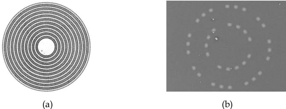
Figure II-9 – (a) Image de la première fibre de Bragg [YEH 78] ; (b) image d'une fibre de Bragg pixélisée de 60 \mu\text{m} de diamètre de champ de mode [YEHOUESSI 16].
