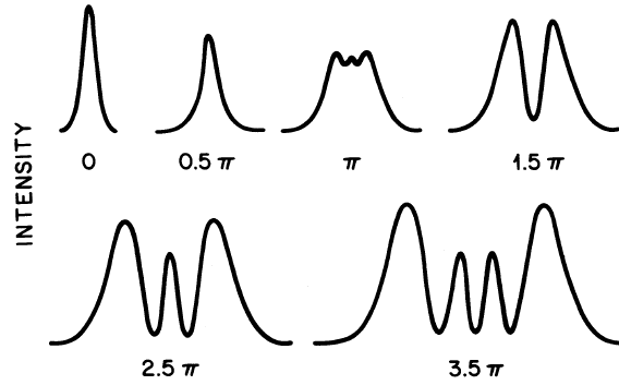
Figure I-11 – Élargissement spectral dû à l'auto-modulation de phase d'une impulsion gaussienne non-chirpée pour différentes valeurs de \phi_{SPM} [AGRAWAL 07].
