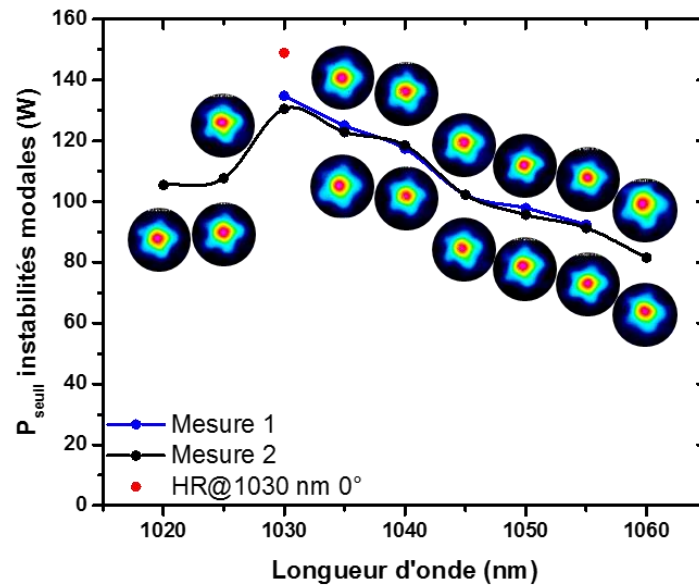
Figure III-14 – Étude de l'influence de la longueur d'onde d'émission sur le seuil des instabilités modales transverses avec en insert les distributions d'intensité du faisceau mesurées en champ lointain avant (sous la courbe) et après (au-dessus de la courbe) l'apparition des instabilités modales transverses. Le point rouge correspond au seuil des instabilités modales avant l'insertion du VBG dans la cavité laser. Deux séries de mesure ont été réalisées pour confirmer la tendance et prouver que la décroissance du seuil n'était pas liée à la décroissance du seuil au cours du temps.
