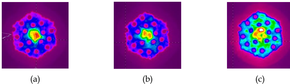
Figure V-2 – Distributions d'intensité du faisceau en champ proche à 1100 nm en sortie de la FA-LPF fortement dopée aux ions ytterbium de 68 \mu\text{m} de diamètre de champ de mode et de \Delta n \approx 8.10^{-5} avec une excitation préférentielle du \text{LP}_{01} (a) ; du \text{LP}_{11} (b) et du \text{LP}_{21} (c).
