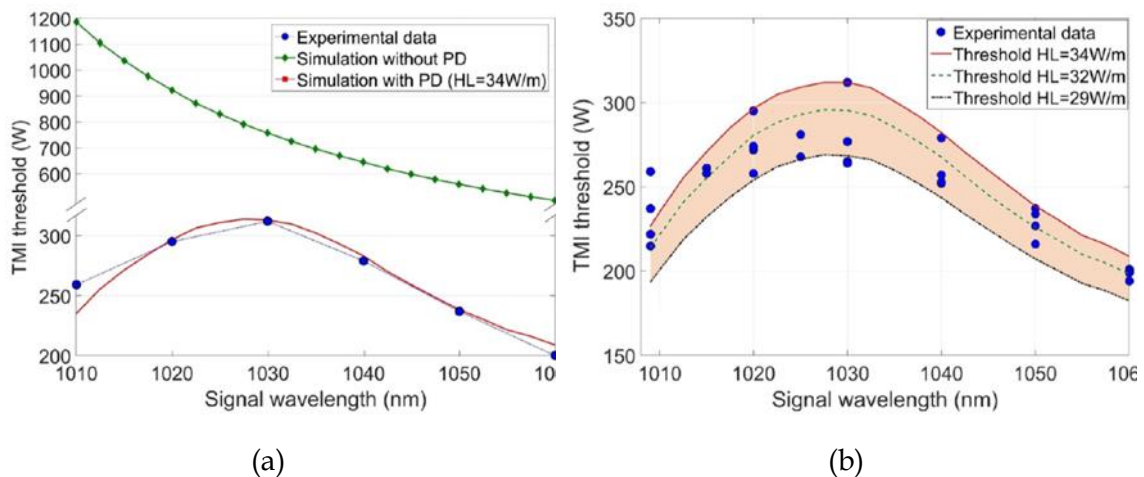
Figure II-17 – (a) Comparaison des valeurs du seuil des instabilités modales transverses les plus élevées mesurées expérimentalement (points bleus) et des résultats de simulation avec (ligne rouge) et sans (ligne verte) prise en compte du photo-noircissement. (b) Comparaison de l'évolution des seuils d'instabilités modales transverses mesurés expérimentalement et simulés selon la longueur d'onde signal pour une LPF de 63 \mu\text{m} de diamètre de cœur ( L = 1,2 m, diamètre de gaine d'air \approx 200 \mu\text{m} , P_{\text{seed}} \approx 30 W). La simulation a été réalisée en considérant différentes valeurs de charge thermique (34 \text{W.m}^{-1} pour la ligne rouge, 32 \text{W.m}^{-1} pour la ligne en pointillés verte et 29 \text{W.m}^{-1} pour la ligne en pointillés noire) [JAUREGUI 15].
