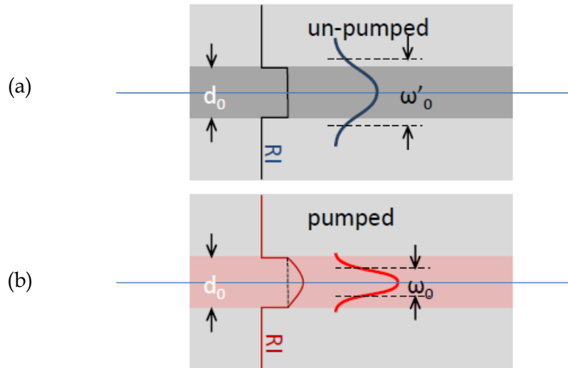
Figure II-11 – (a) Représentation schématisée d'une fibre à saut d'indice « à froid » (non impactée par la charge thermique) ; (b) profil d'indice quasi-parabolique d'une fibre à saut d'indice « à chaud » (en présence de charge thermique) et réduction du diamètre de champ modal [ZERVAS 18].
