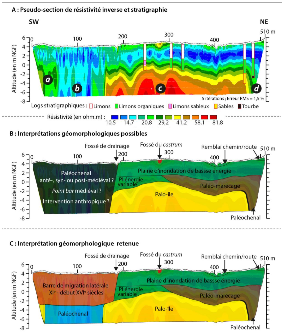
Fig. 83 – Profil ERT P1 de Langoiran : palette de résistivité de référence et difficultés d'interprétation. Espacement inter-électrode de 1 m ; pseudo-section réalisée par Clément Virmoux. Le couplage avec la stratigraphie permet de préciser la résistivité des strates les plus épaisses tels que les limons : 10-20 ohm/m ; les limons sableux ou organiques : 14-35 ohm/m ; les sables : 35-60 ohm/m ; les graviers/galets : > 60 ohm/m. L'île atlantique est nettement identifiable entre les mètres 280 et 510 grâce à sa résistivité accrue. Elle correspond à l'emplacement supposé par la topographie. Le paléochenal qui lui est contemporain au NE est très partiellement recoupé par la prospection ce qui empêche de préciser sa géométrie. Entre les mètres 60 et 130, la chute de résistivité est complexe à interpréter. Toutes les données acquises jusqu'à présent dans ce secteur démontraient qu'il avait été recoupé par le chenal médiéval à partir du fossé de drainage (mètre 190). Or, l'augmentation de la résistivité vers le SW remet cette hypothèse en doute. Il pourrait s'agir d'un profond chenal atlantique ou, au contraire, d'un chenal médiéval peu profond et/ou ayant connu un changement hydrologique majeur. Il est même envisageable que ce soit un paléochenal d'un autre temps, sans oublier la possibilité d'une intervention anthropique. Finalement, l'hypothèse retenue est celle d'un chenal médiéval peu profond en migration ( point bar ).
