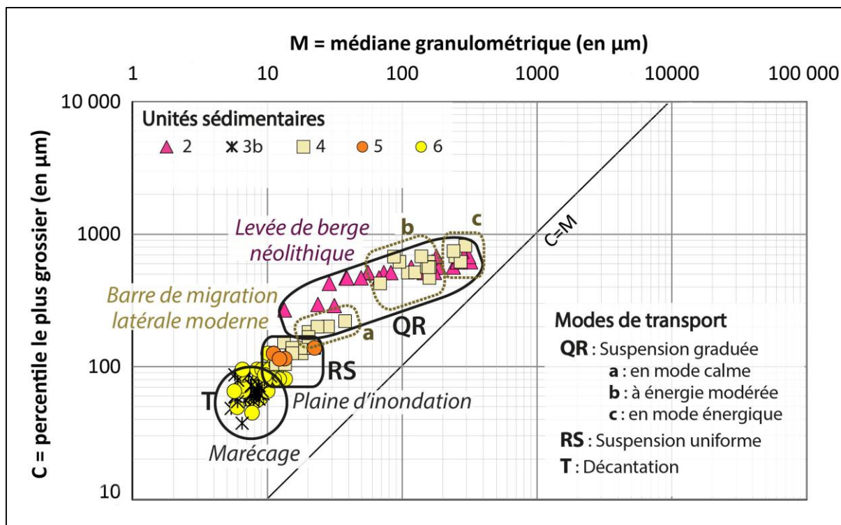
Fig. 72 – Image CM du transect stratigraphique 4 de Langoiran. L'unité interprétée comme un banc de migration latérale s'étire de la suspension uniforme ( C > 106 \mu\text{m} ) à la suspension graduée ( C < 824 \mu\text{m} ). Trois types de suspension graduée peuvent être distingués pour la barre de migration latérale : la suspension graduée en mode calme ( a ; 105 < C < 223 \mu\text{m} ; M < 40 \mu\text{m} ), celle à énergie modérée ( b ; 429 < C < 685 \mu\text{m} ; 60 < M < 160 \mu\text{m} ) et celle en mode énergétique ( c ; 623 < C < 824 \mu\text{m} ; M > 200 \mu\text{m} ). Le marécage (unité 3) et la plaine d'inondation (5-6) occupent les mêmes positions sur cette image CM que sur les images précédentes.
