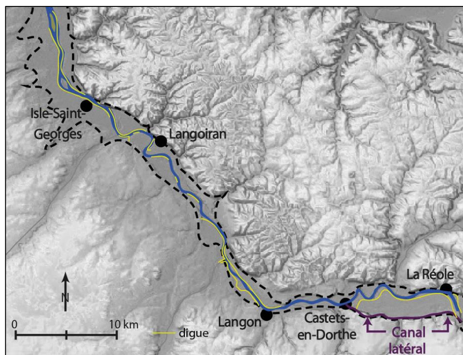
Fig. 32 – Les digues de la Garonne maritime en amont de Bordeaux.
