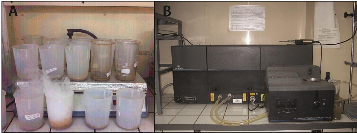
Fig. 52 – Analyse granulométrique des sédiments. A : Élimination de la matière organique au peroxyde d'hydrogène, avec un premier passage à froid puis à chaud ; B : Passage des sédiments au granulo-mètre laser Beckman Coulter LS 230.
