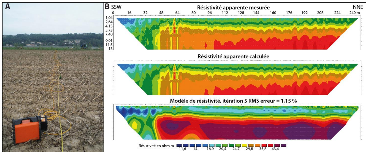
Fig. 56 – Acquisition (A) et interprétation (B) des données de résistivité électrique (P4 de Langoiran). Le facteur d'erreur RMS ( Root Mean Squared ) quantifie la différence entre les valeurs de résistivités apparentes mesurées et celle calculées par le programme de traitement. La pseudo-section P4 de Langoiran a été réalisée avec un espacement inter-électrode de 2 m et démontre la présence d'un chenal au SSW via une chute de la résistivité.
