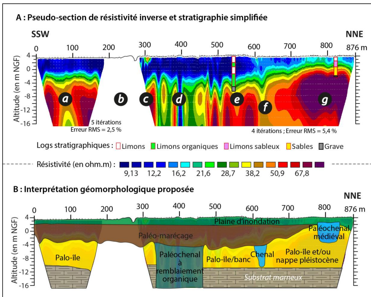
Fig. 105 – Profils ERT P2 et P3 d'Isle-Saint-Georges. Espacement inter-électrode de 3 m ; pseudo-section construite par Clément Virmoux ; rapport profondeur/distance : 1/10. En réalité, le profil P2 atteint 32 m de profondeur. Ici, il a été coupé à 20 m pour s'aligner sur le second profil, ce qui fut permis par l'absence d'alluvions holocène au-delà de cette profondeur.
