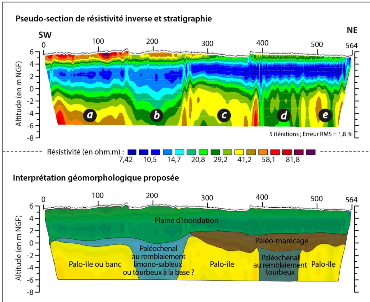
Fig. 87 – Profil ERT P3 de Langoiran : confirmation du système anastomosé atlantique ? Espacement inter-électrode de 1 m ; pseudo-section réalisée par Clément Virmoux. Le profil électrique traverse également trois entités relativement résistantes (80-130 m de large) séparés par deux chutes verticales de la résistivité (80-115 m de large). Cette succession latérale appuie la thèse d'un système anastomosé à l'Atlantique ancien.
