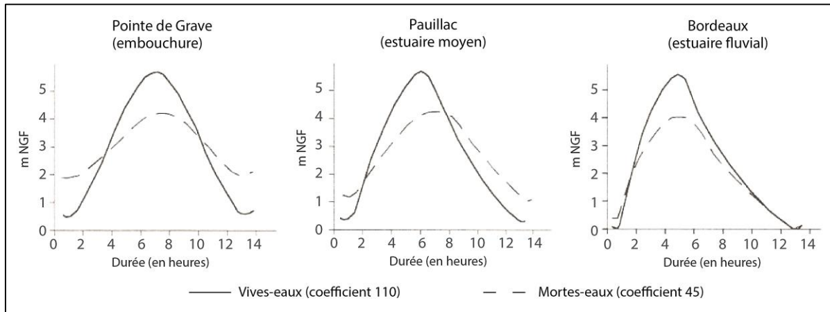
Fig. 17 – Évolution de l'onde de marée dans l'estuaire Garonne-Dordogne-Gironde. Courbes marégraphiques reprises d'Allen, 1972.
