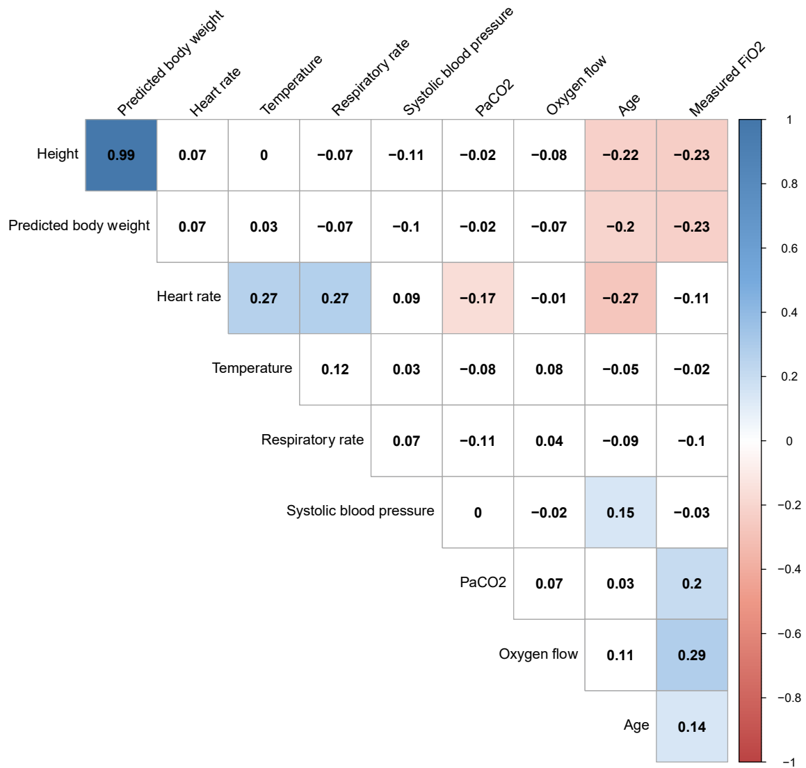
Figure 7. Corrélogramme montrant les coefficients de rang de Spearman parmi les variables analysées. Les corrélations positives significatives sont colorées en bleu et les corrélations négatives significatives sont colorées en rouge. Plus les couleurs sont foncées, plus la corrélation est forte.
