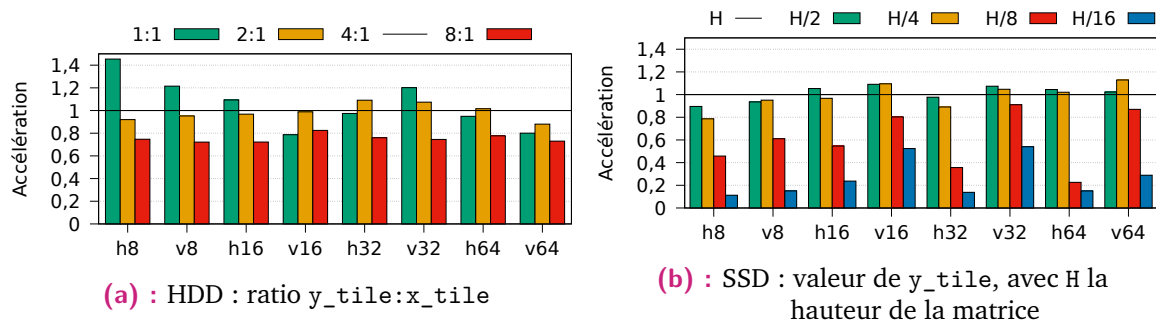
Figure 4.2 : Accélération moyenne obtenue en fonction de la dimension des tuiles de lecture ( y\_tile \times x\_tile ) et d'écriture ( x\_tile \times y\_tile ) par rapport à la valeur choisie dans notre solution avec une mémoire temporaire src de 1 Go sur des matrices d'orientations et de tailles différentes (de 8 Go à 64 Go)
