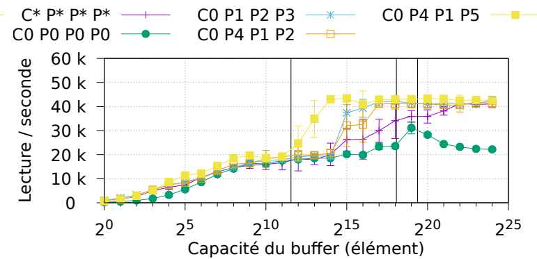
(b) : Attente yield
