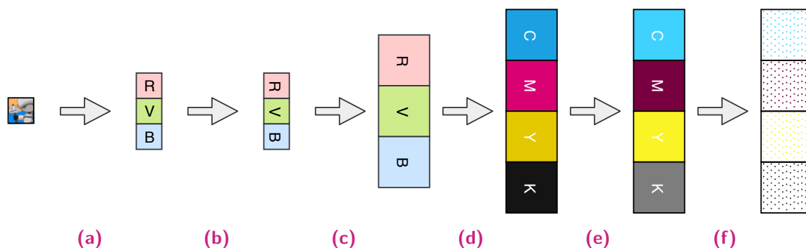
Figure 2.1 : Schématisation des différents traitements graphiques successifs réalisés par un RIP sur l'image d'entrée lors de la génération des données pour une imprimante, avec RVB pour Rouge-Vert-Bleu et CMYK pour Cyan-Magenta-Yellow-Black, (a) décodage, (b) prétraitement, (c) mise à l'échelle, (d) colorimétrie, (e) limitation et linéarisation, et (f) tramage
