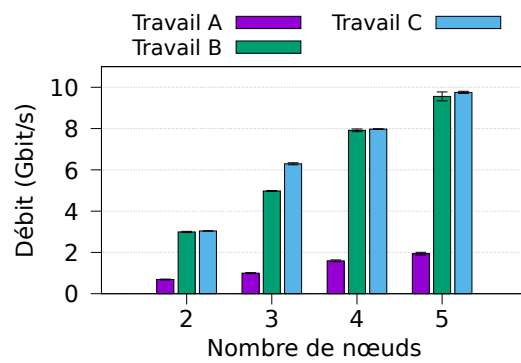
(d) : many-to-many
