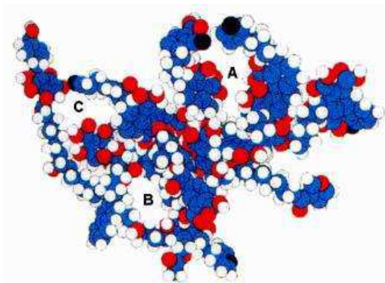
Figura 4: Modelo estrutural propostos pela teoria macromolecular Schulten & Schnitzer (1997), em que as esferas azuis, vermelhas, brancas e pretas representam os átomos de carbono, oxigênio, hidrogênio e nitrogênio, respectivamente. As letras A, B e C indicam os espaços “vazios” presentes na molécula das SH capazes de interagir com outros compostos
