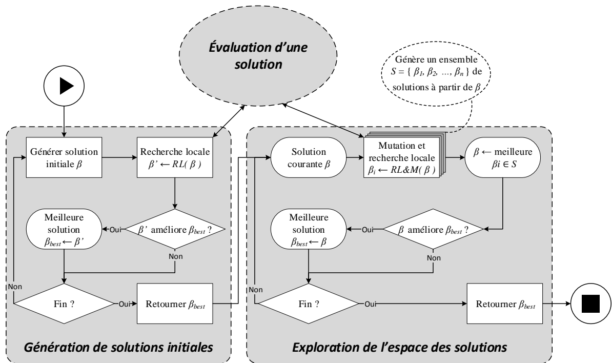
Figure 2.4 : Schéma global de l'algorithme ELS
