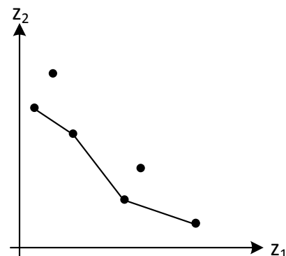
(3) – Les nouvelles solutions sont insérées dans la population à la fin de la génération i formant ainsi un nouveau front
