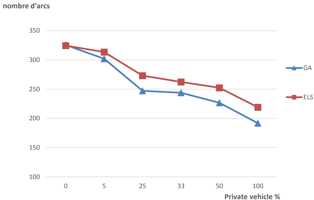
Figure 3.30 : Comparaison de la moyenne du nombre d'arcs utilisés
