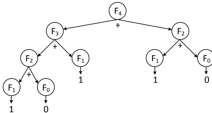
Figure 1.8 : Arbre d'appels de fonctions pour calculer le 4 ème terme de Fibonacci. F_0, F_1 et F_2 sont calculées plusieurs fois
