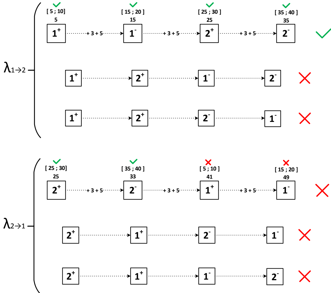
Figure 3.17 : Test de précedence entre les clients 1 et 2 : une contrainte existe forçant le sommet de pickup du client 1 à être servi avant le sommet de pickup du client 2
