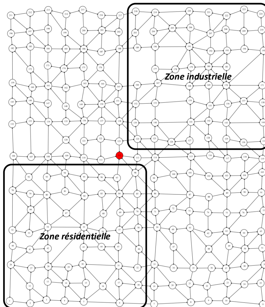
Figure 2.17 : Détermination d'une zone résidentielle et d'une zone de travail dans le graphe
