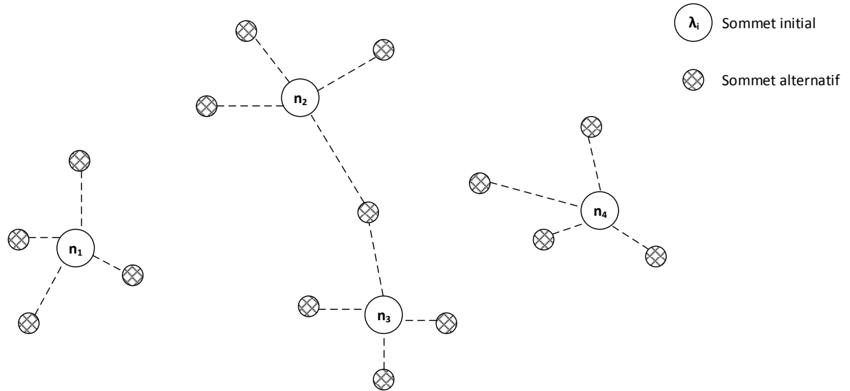
Figure 2.3 : Sommets initiaux avec sommets alternatifs associés, n_2 et n_3 ayant un sommet alternatif commun
