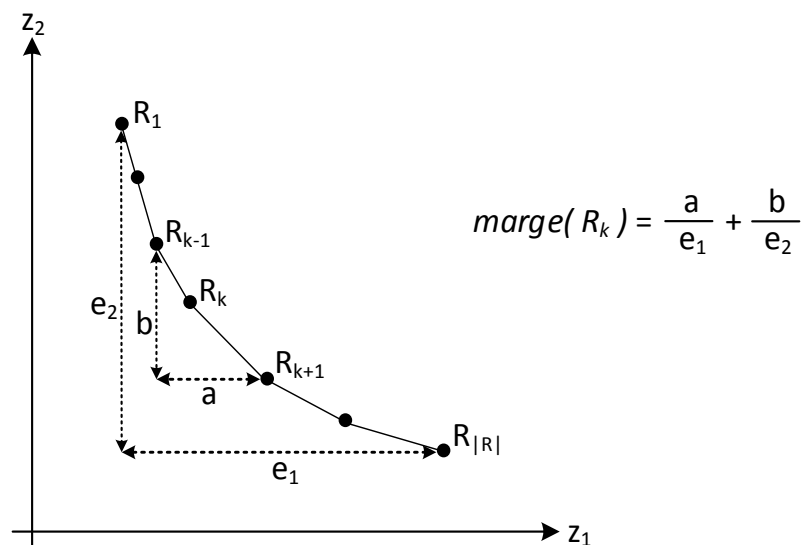
Figure 4.11 : Calcul de la marge associée à un individu représentant une solution (Deb et al., 2002)
