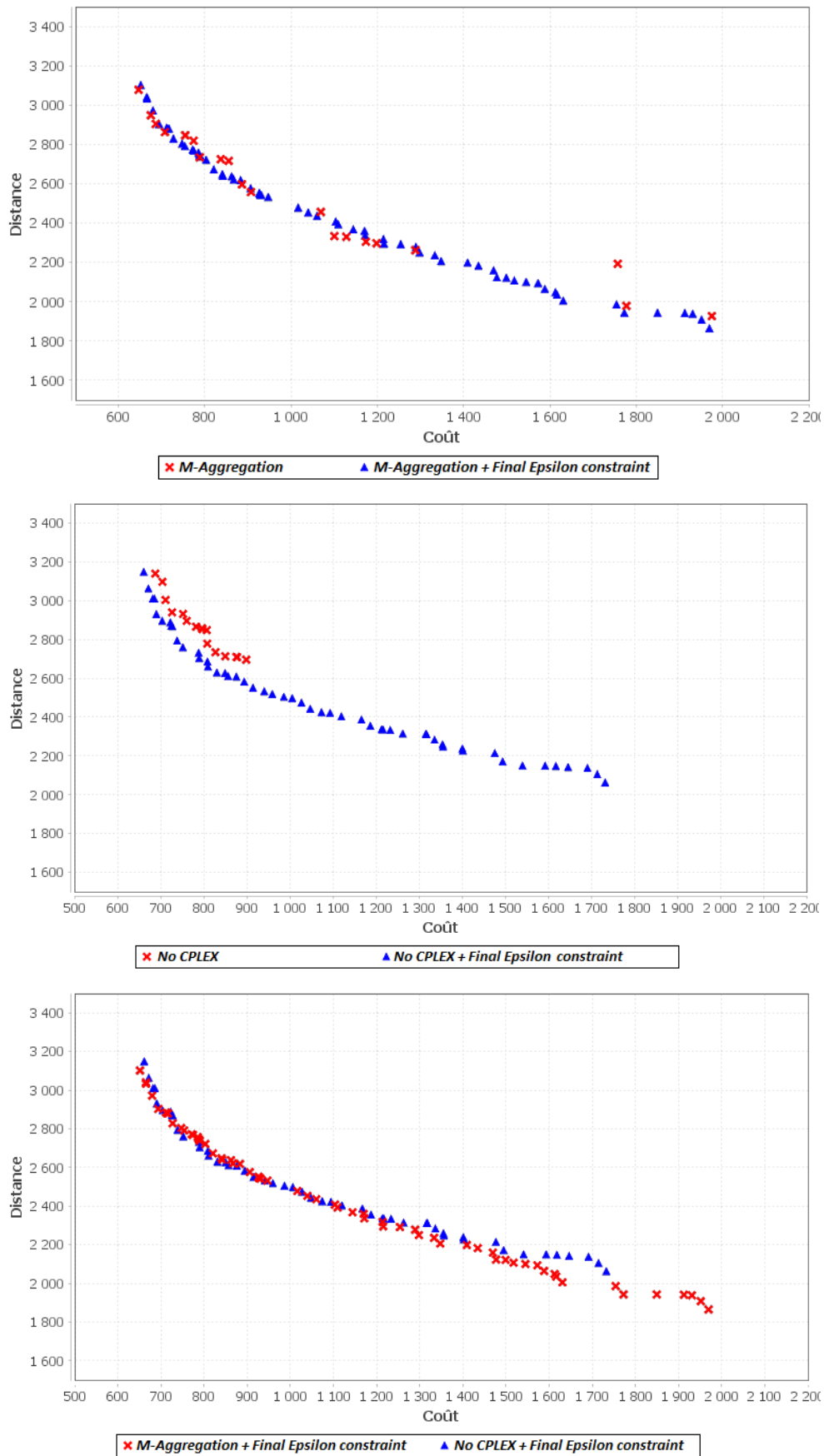
Figure 4.23 : Comparaison des fronts de Pareto sans et avec la méthode \epsilon -contrainte en fin d'algorithme sur l'instance PCD_120_60VP avec le scénario 5
