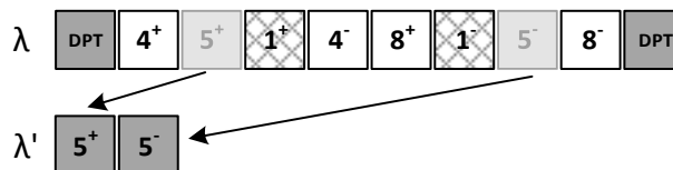
Figure 2.14 : Création de la tournée privée
