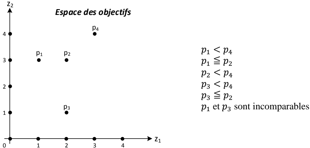
Figure 4.3 : Comparaison des relations de dominance entre différents points
