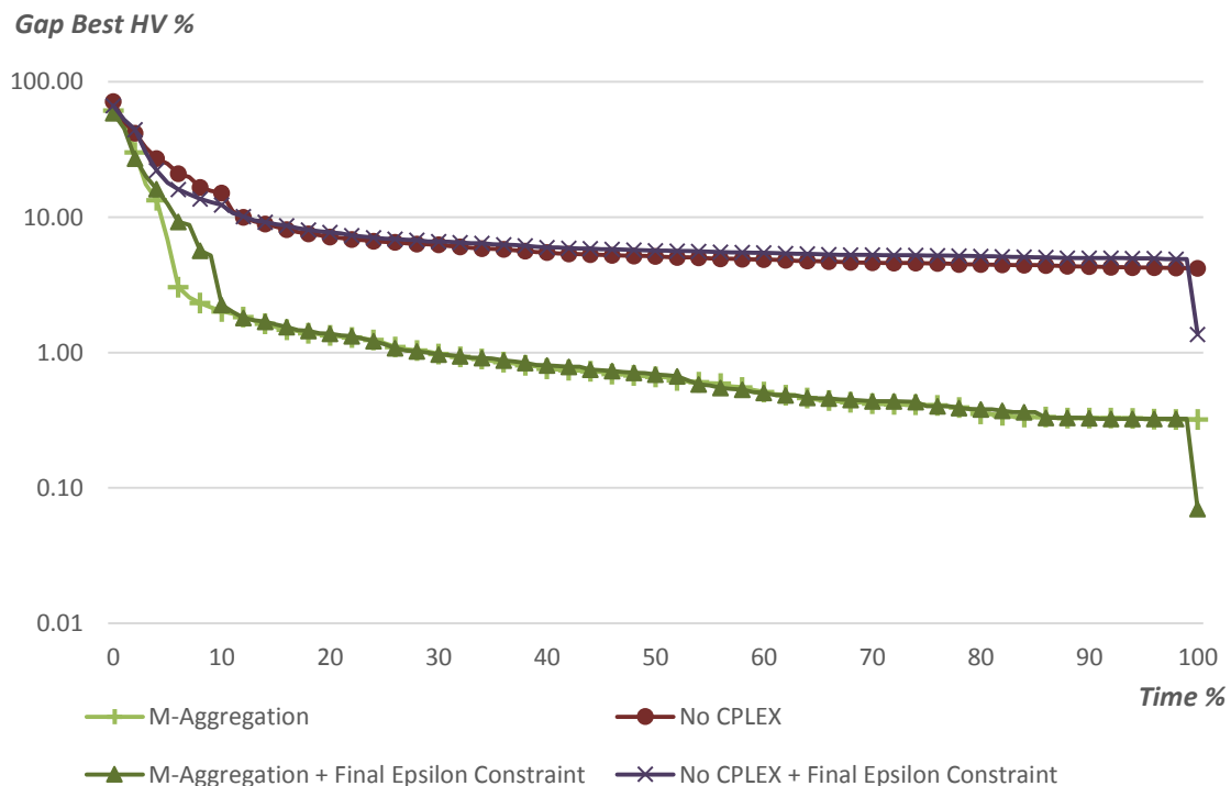
Figure 4.22 : Convergence de l'hypervolume des approches utilisant la méthode \epsilon -contrainte en fin d'algorithme
