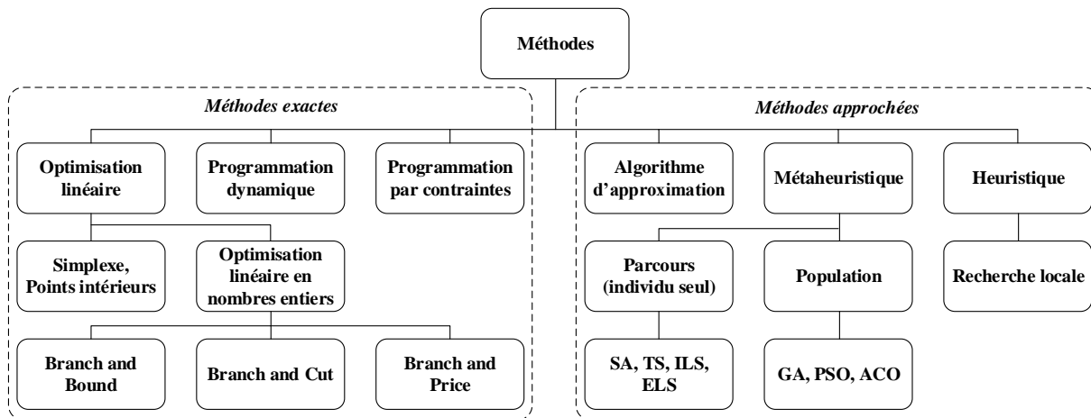
Figure 1.7 : Les différentes méthodes de résolutions pour les problèmes de transport
