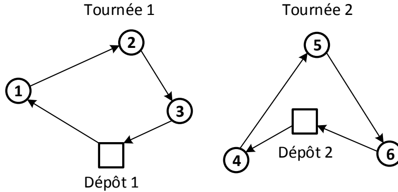
Figure 1.4 : Exemple de solution sur un problème de tournées de véhicules comportant deux dépôts
