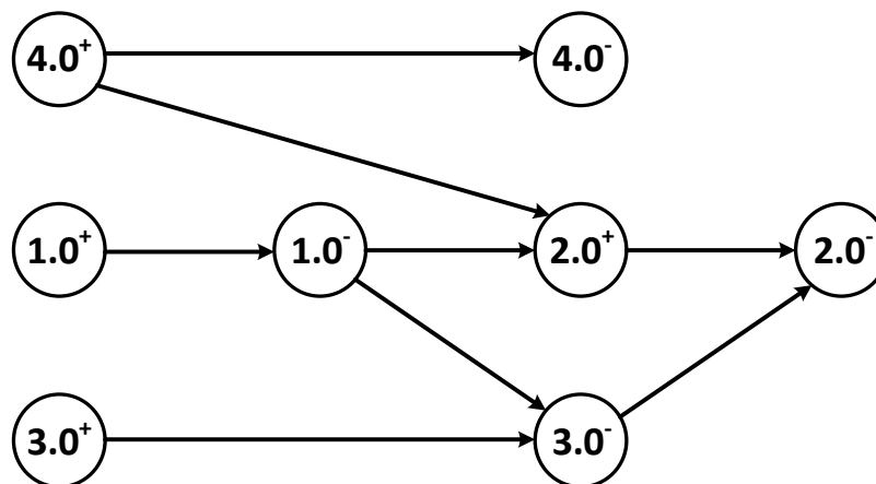
Figure 3.15 : Graphe de précédence entre les différents sommets de pickup et delivery des clients
