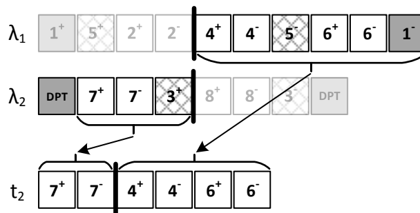
Figure 2.9 : Création de la tournée t_2
