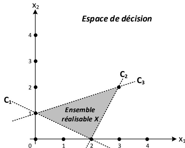
Figure 4.1 : Espace de décision à deux variables et ensemble réalisable respectant les contraintes C_1 , C_2 et C_3
