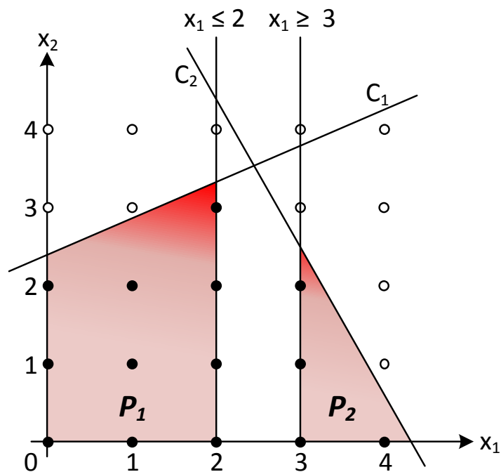
Figure 1.10 : Phase de séparation en deux sous-problèmes P_1 et P_2
