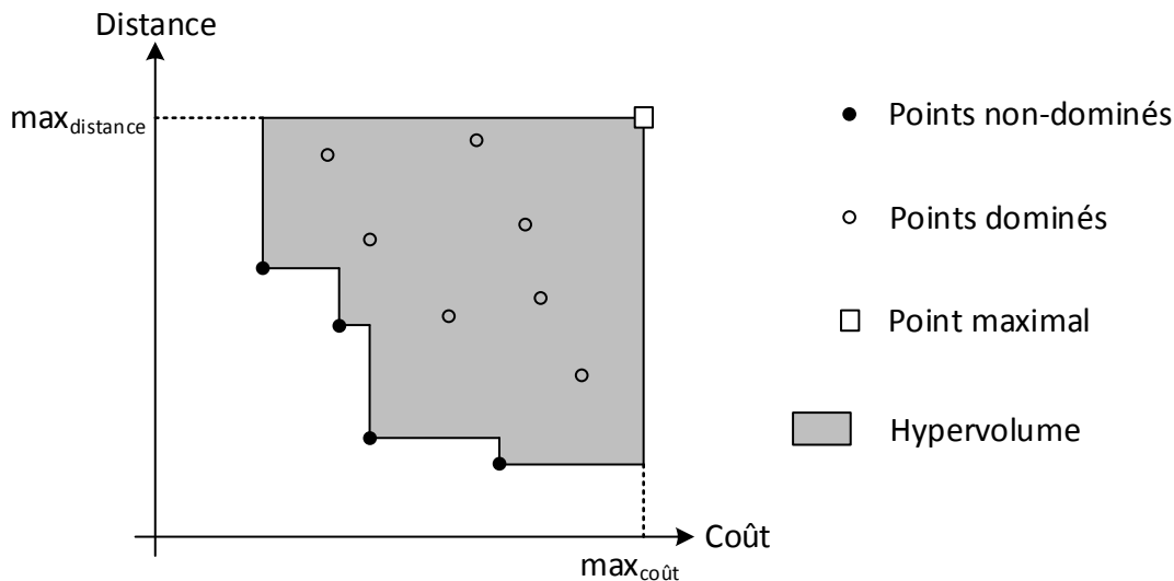
Figure 4.17 : Exemple de front de Pareto avec sa mesure d'hypervolume
