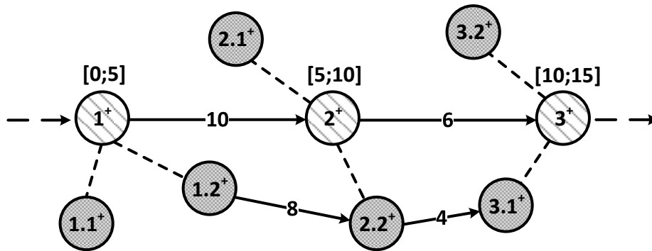
Figure 3.1 : Fausse estimation si les sommets alternatifs sont trop éloignés des sommets initiaux
