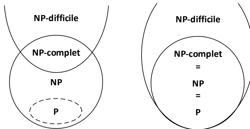
Figure 1.6 : Inclusion des classes si P \neq NP (gauche) et si P = NP (droite)
