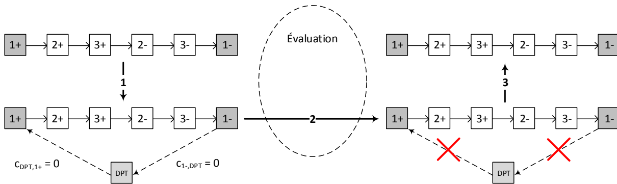
Figure 2.5 : Évaluation d'une tournée effectuée par un véhicule privé en utilisant des arcs à coût nul
