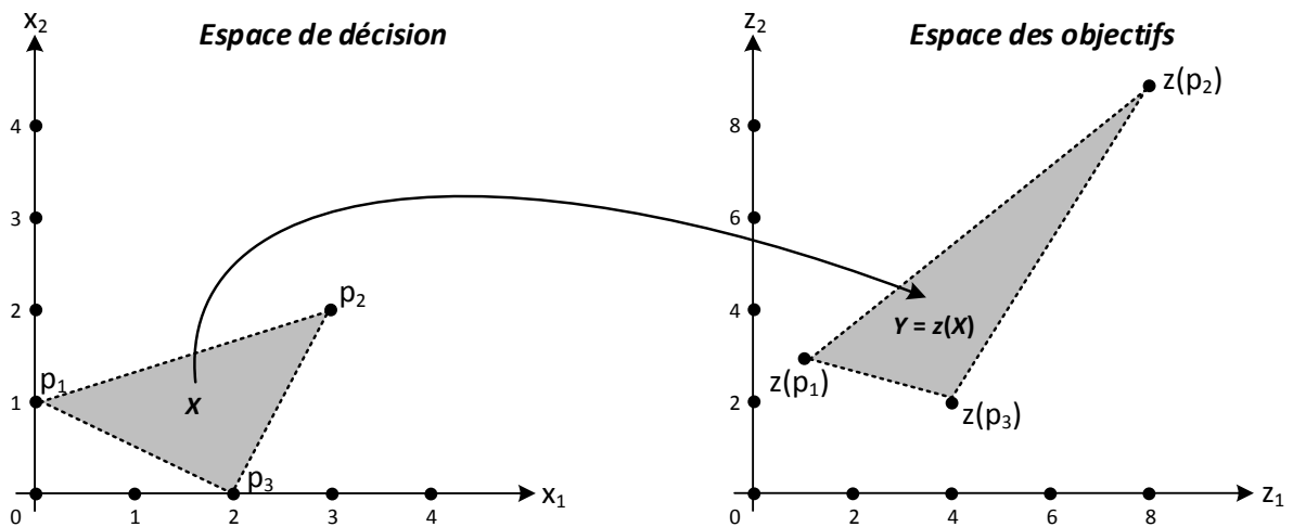
Figure 4.2 : Espace des objectifs avec deux critères pour l'espace de décision de la Figure 4.1
