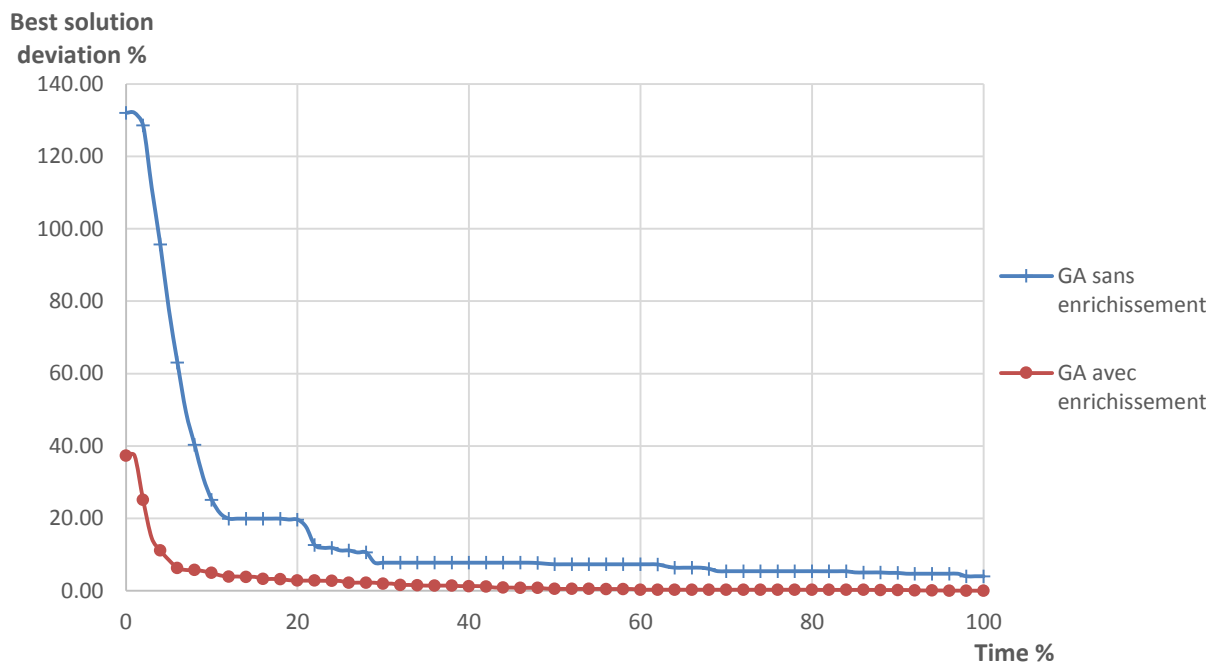
Figure 3.33 : Comparaison des vitesses de convergence de l'algorithme génétique avec et sans enrichissement de la population
