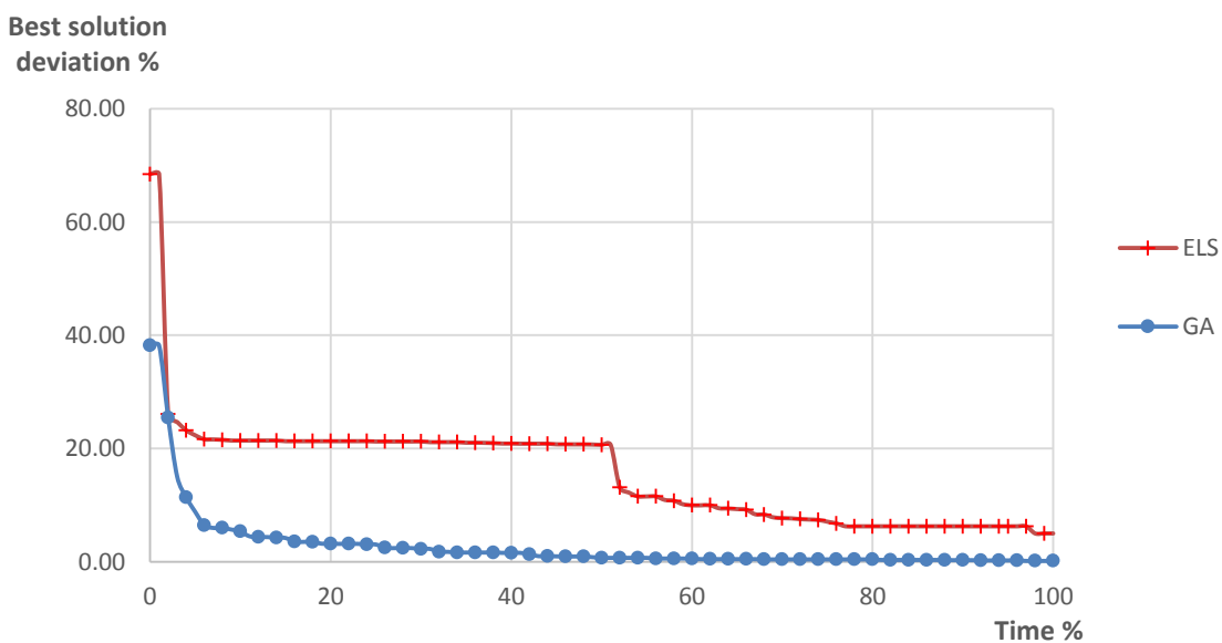
Figure 3.32 : Comparaison des vitesses de convergence des deux méthodes de résolution
