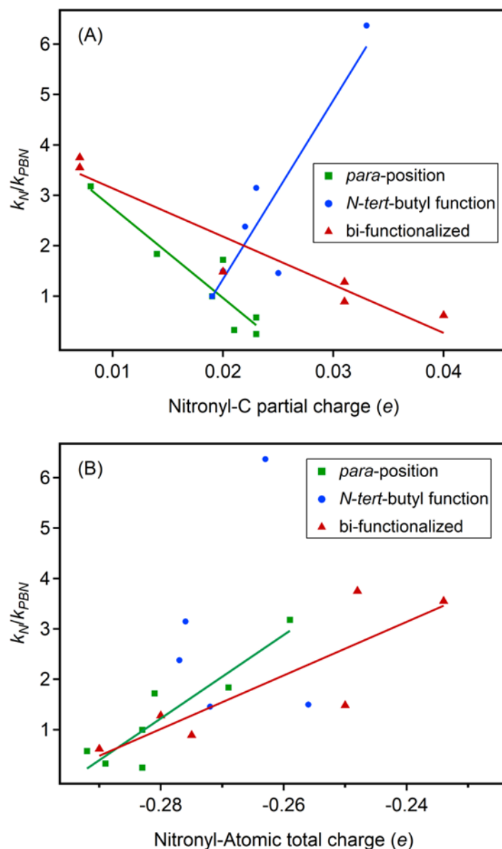
Figure 3. Tracé des constantes de vitesse relatives de piégeage du radical \cdot\text{CH}_2\text{OH} en fonction de (A) : la charge partielle du carbone et (B) : la charge totale atomique de la fonction nitronyle pour les dérivés modifiés en para (■) ((A) : R^2 = 0,87 et (B) : R^2 = 0,83 , en excluant les valeurs aberrantes de 4-Ph-PBN et 4-MeO-PBN), ceux modifiés sur la partie N - tert -butyle (●) ((A) : R^2 = 0,82 ), et les dérivés bi-fonctionnalisés (▲) ((A) : R^2 = 0,91 et (B) : R^2 = 0,65 en excluant la valeur aberrante de 4-MeO-PPN).
