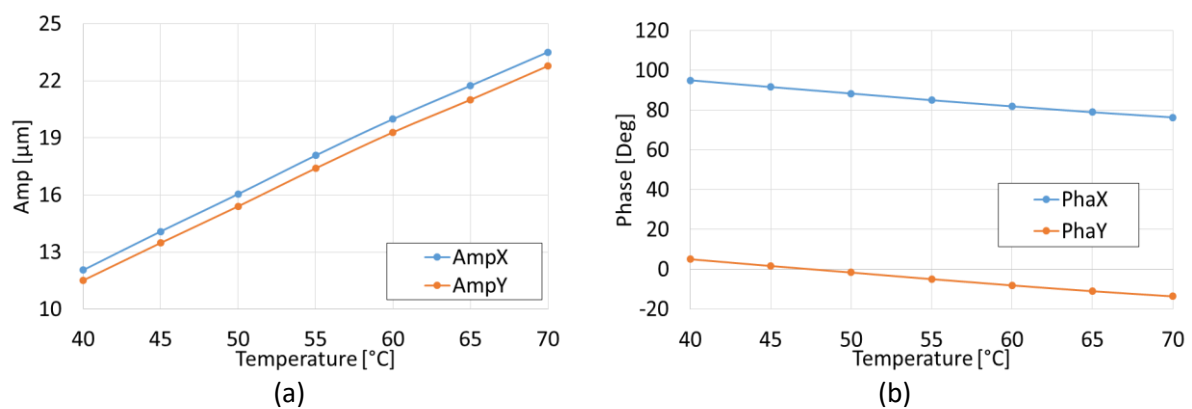
Figure 4.3-4 : Evolution des amplitudes (a) et des phases (b) avec la température pour un balourd constant
