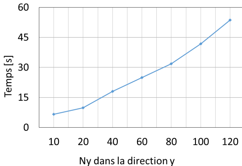
Figure 2.4-5 : Temps de calcul de la NDM pour différents nombres de cellules
