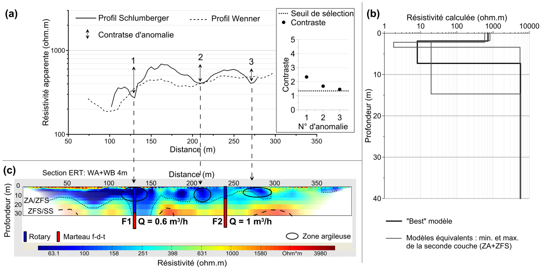
Figure 6.8 – Profil électrique (PE), sondage électrique (SE) et tomographie de résistivité électrique (ERT) sur le site Saré. a) PE avec les dispositifs Schlumberger et Wenner ; b) SE réalisé sur l'anomalie N°1 du PE Schlumberger ; c) ERT utilisant les dispositifs combinés Wenner alpha (WA) et Wenner beta (WB).
