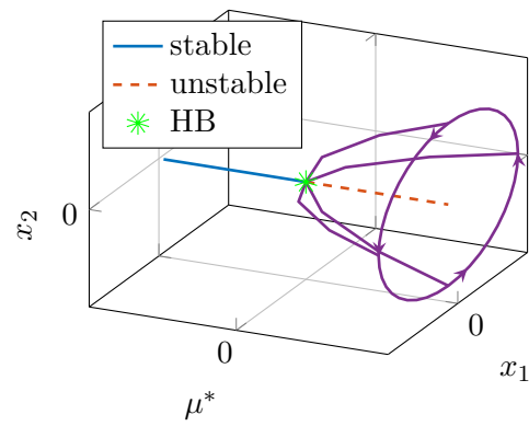
(d) Andronov-Hopf-bifurcation.
