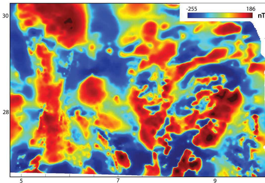
Figure II-12 : Carte magnétique de la grille de donnée du bassin d'Illizi ( IL32 )
