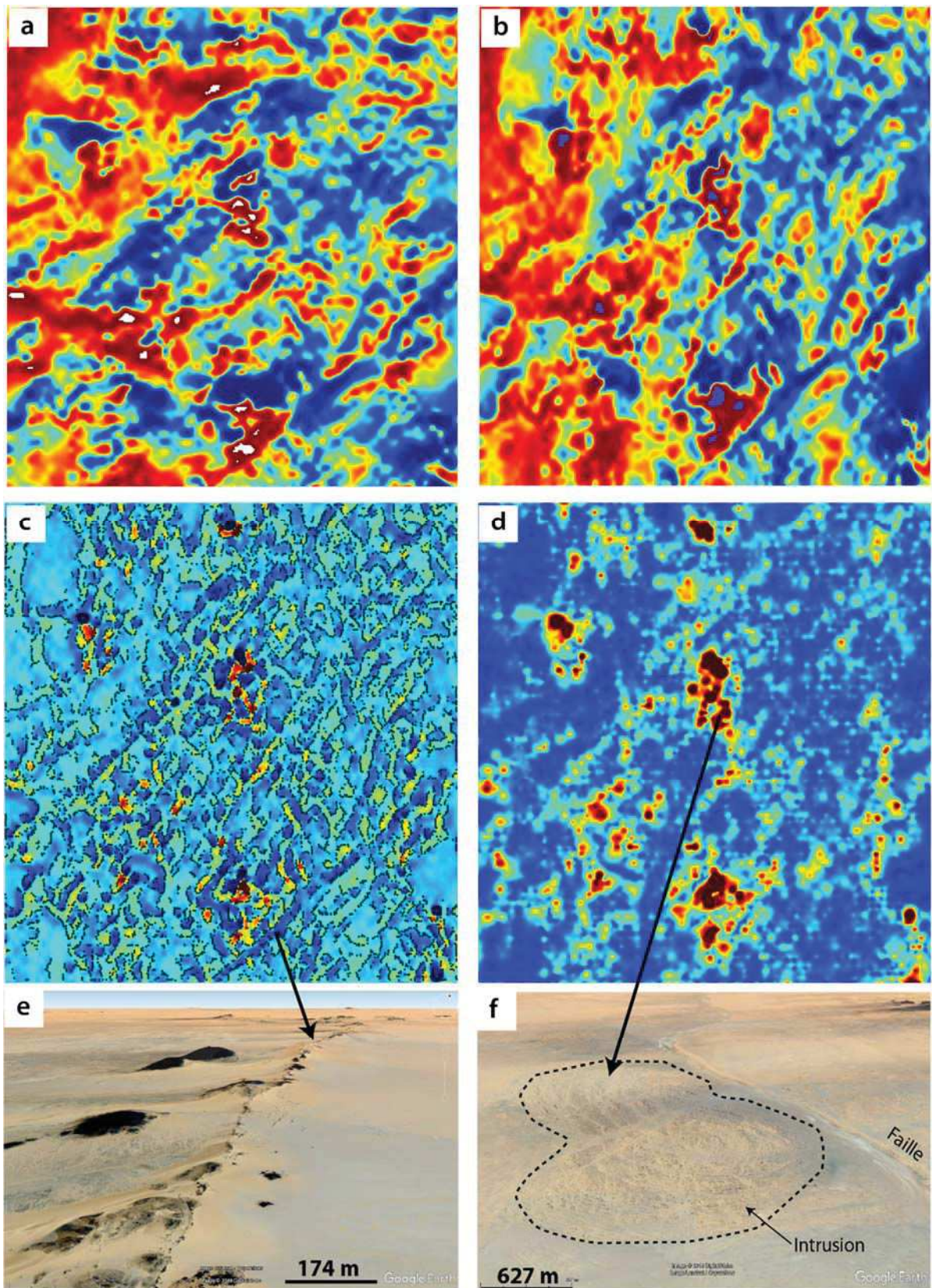
Cartes magnétiques transformées (a. Anomalies magnétiques ; b. Anomalies magnétiques réduite au pôle ; c. Dérivée verticale ; d. Signal analytique) ; mettant en évidence linéations magnétiques et (f) failles et (f) intrusions magmatiques (images de Google-Earth) dans le socle du Hoggar sur. (Echelle de cartes magnétiques : 1x1 degré décimal)
