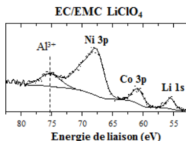
Figure 5-5 : (a) Pics de cœur XPS Al 3p, Ni 3p, Co 3p et Li 1s acquis à la surface d'une électrode de NMC cyclées vs LTO à 40°C à C/2 D/2 dans EC/EMC et \text{LiClO}_4 à la fin du centième cycle
