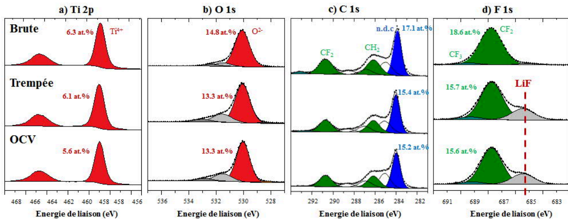
Figure 4-4 : Pics de cœur Ti 2p a), O 1s b), C 1s c) et F 1s d) de l'électrode LTO de référence brute (1 ère ligne), trempée (2 ème ligne) et après OCV face au NMC dans un électrolyte composé de EC/EMC (3:7) LiPF_6 (1M), à 60°C pendant 15h
