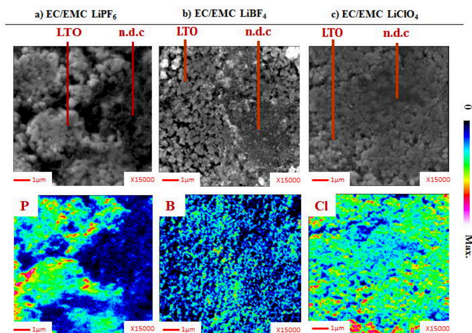
Figure 5-6 : Clichés SEM (1 ère ligne) de la surface des électrodes de LTO en fin de 100 ième lithiation cyclées versus NMC avec les sels \text{LiPF}_6 a), \text{LiBF}_4 b) et \text{LiClO}_4 c) ; et cartographies chimiques (2 ème ligne) réalisées par spectroscopie des électrons Auger, représentant la répartition chimique du phosphore (P), du bore (B) et du chlore (Cl)
