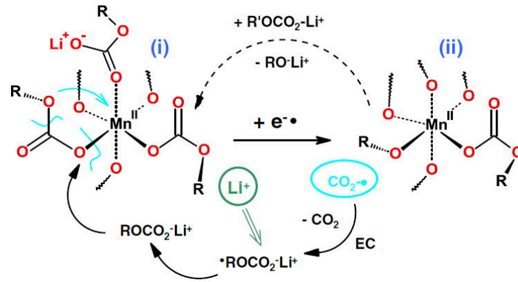
Figure 1-29 : Représentation schématique du mécanisme électro-catalytique de Leung pour les ions Mn II dans le SEI. La complexation des anions par Mn II dans la matrice SEI donne un centre actif (complexe i).
