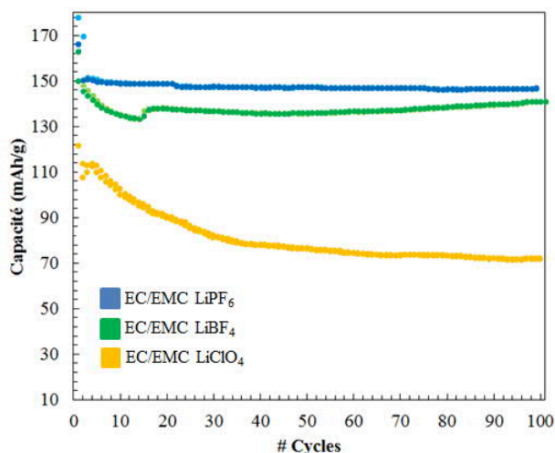
Figure 5-1 : Evolution de la capacité au cours du cyclage des cellules LTO//NMC avec le sel LiPF 6 (bleu), LiBF 4 (vert) et LiClO 4 (jaune)
