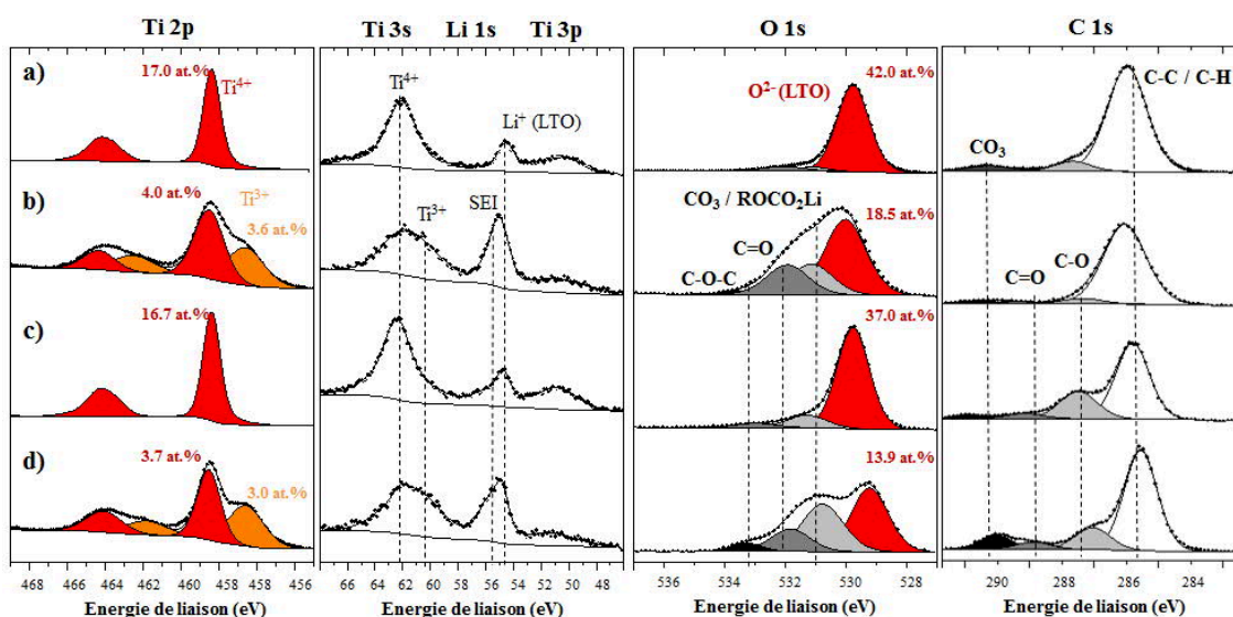
Figure 5-27 : Pics de cœur Ti 2p, Ti 3s, Li 1s, Ti 3p, O 1s et C 1s de l'électrode LTO de référence brute trempée dans l'hexane (1 ère ligne, a), lithiée chimiquement (2 ème ligne, b), brute trempée dans l'électrolyte (3 ème ligne, c) et lithiée chimiquement puis trempée dans l'électrolyte (4 ème ligne, d)
