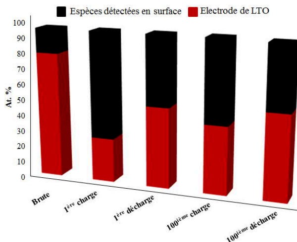
Figure 3-11 : Analyse quantitative sous forme d'histogramme via addition des différents pourcentages atomiques (at.%) associés aux environnements chimiques identifiés par XPS en surface des électrodes LTO brutes et cyclées en piles complètes face au LFP jusqu'en fin de première et centième lithiation, de première et centième délithiation, avec un électrolyte EC/EMC-1M LiPF6
