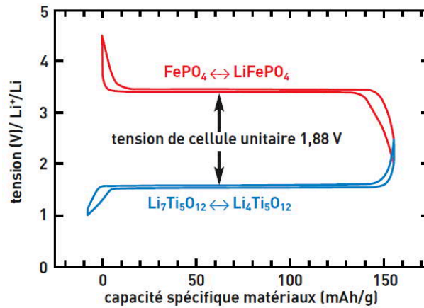
Figure 1-14 : Courbe d'une charge galvanostatique de LFP face au LTO entre 2,5 et 4,2 V vs \text{Li}^+/\text{Li}^0
