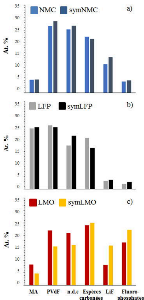
Figure 3-29 : Analyse XPS quantitative sous forme d'histogrammes des électrodes de (a) NMC, (b) LFP et (c) LMO cyclées en symétriques
