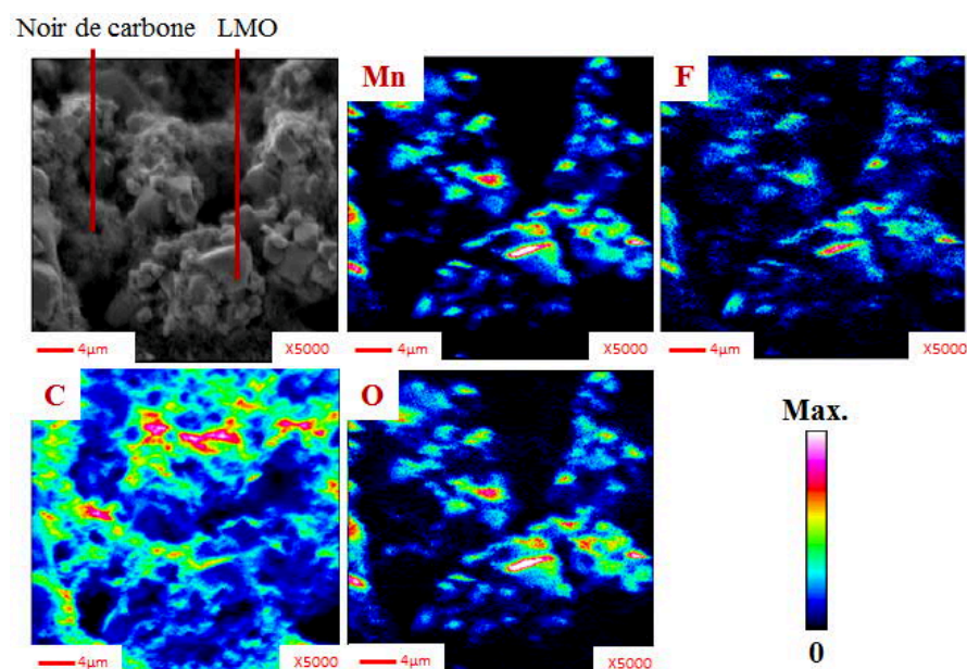
Figure 2-30 : (De gauche à droite et de haut en bas) Cliché SEM de la surface de l'électrode LMO brute non cyclée ; Cartographies chimiques réalisées par spectroscopie des électrons Auger, représentant la répartition chimique du manganèse (Mn), du fluor (F) du carbone (C), et de l'oxygène (O)
