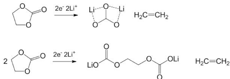
Figure 4-18 : Réduction de EC à bas potentiel [11]
