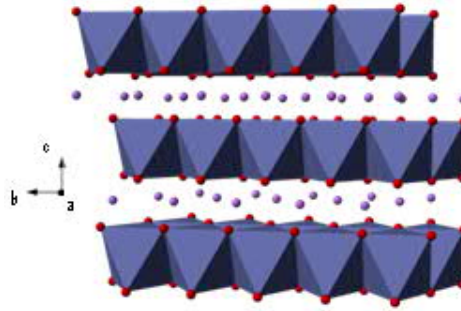
Figure 1-9 : Structure cristalline de \text{LiMO}_2 ( ● Li ● Oxygène )
