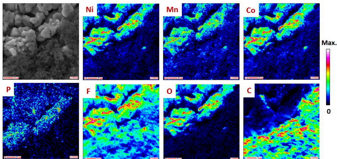
Figure 3-4 : (De gauche à droite et de haut en bas) Cliché SEM de la surface de l'électrode NMC en fin de 100 ième lithiation ; Cartographies chimiques réalisées par spectroscopie des électrons Auger, représentant la répartition chimique du nickel (Ni), du manganèse (Mn), du cobalt (Co), du phosphore (P), du fluor (F), de l'oxygène (O) et du carbone (C)
