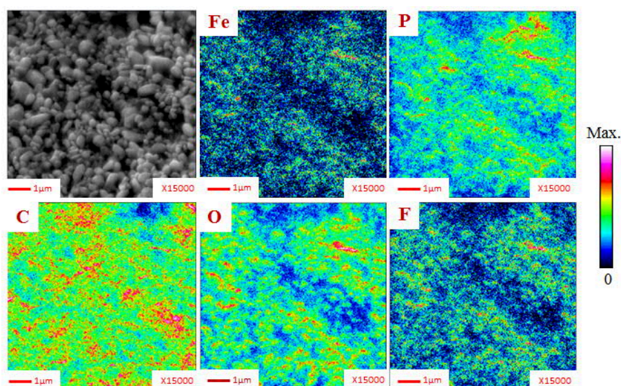
Figure 2-32 : (De gauche à droite et de haut en bas) Cliché SEM de la surface de l'électrode LFP brute non cyclée ; Cartographies chimiques réalisées par spectroscopie des électrons Auger, représentant la répartition chimique du fer (Fe), du phosphore (P), du carbone (C), de l'oxygène (O) et du fluor (F)
