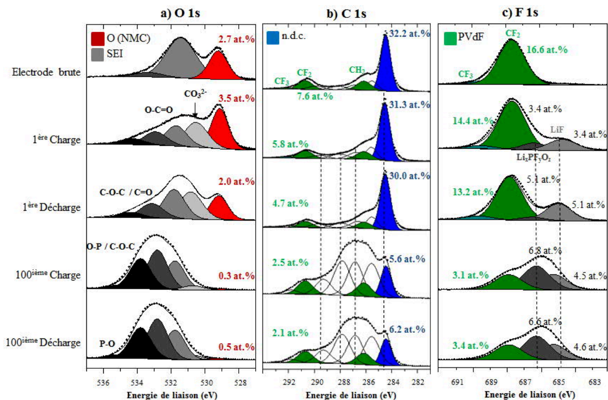
Figure 3-20 : Analyse XPS pics de cœur C 1s de (a) l'électrode NMC de référence non cyclée ; des électrodes NMC cyclées en bi-boutons en (b) fin de 1 ère délithiation, (c) fin de 1 ère lithiation, (d) fin de 100 ième délithiation et (e) fin de 100 ième lithiation ; pic de cœur O 1s de (f) l'électrode NMC de référence non cyclée ; des électrodes NMC cyclées en (f) fin de 1 ère délithiation, (h) fin de 1 ère lithiation, (i) fin de 100 ième délithiation et (j) fin de 100 ième lithiation ; pics de cœur F 1s de (k) l'électrode NMC de référence non cyclée ; des électrodes NMC cyclées en (l) fin de 1 ère délithiation, (m) fin de 1 ère lithiation, (n) fin de 100 ième délithiation et (o) fin de 100 ième lithiation
