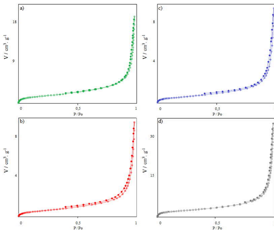
Figure 2-3 : Isothermes d'adsorption/désorption de l'azote pour les électrodes de LTO (a), LFP (b), NMC (c) et LMO (d)
