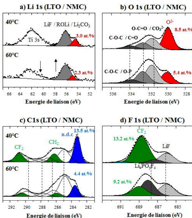
Figure 4-2 : Pics de cœur Li 1s (a), O 1s (b), C 1s (b) et F 1s (c) des électrodes LTO cyclées en boutons complets face au NMC en fin de 100ième lithiation à 40°C (première ligne) et à 60°C (deuxième ligne)
