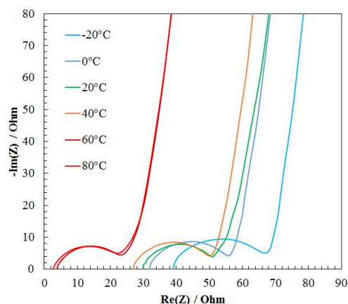
Figure A3-1 : Mesures par spectrométrie d'impédance électrochimique à différentes températures réalisées à l'OCV sur une cellule symétrique LTO vs LTO utilisant l'électrolyte EC/EMC 1M LiPF 6
