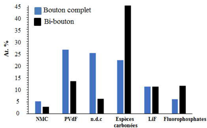
Figure 3-21 : Analyse quantitative sous forme d'histogramme via addition des différents pourcentages atomiques (at.%) associés aux environnements chimiques identifiés par XPS en surface des électrodes NMC cyclées piles complètes (bleues) et en bi-boutons (noirs) en fin de centième cycle, avec un électrolyte EC/EMC-1M LiPF 6
