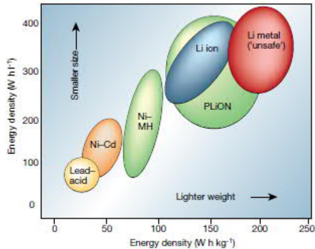
Figure 1-2 : Comparaison des différentes technologies de batteries en termes de densité d'énergie volumétrique et gravimétrique [13]
