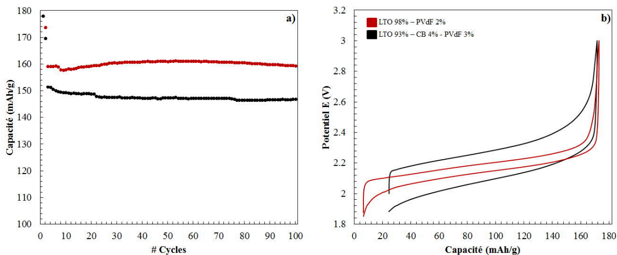
Figure 5-23 : Evolution de la capacité en fonction du nombre de cycle a) et 100ième cycle galvanostatique b) pour le système complet LTO vs NMC effectué dans EC/EMC (3:7) \text{LiPF}_6 (1M) intégrant une électrode de LTO composée de noir de carbone (en noir) et sans noir de carbone (en rouge)
