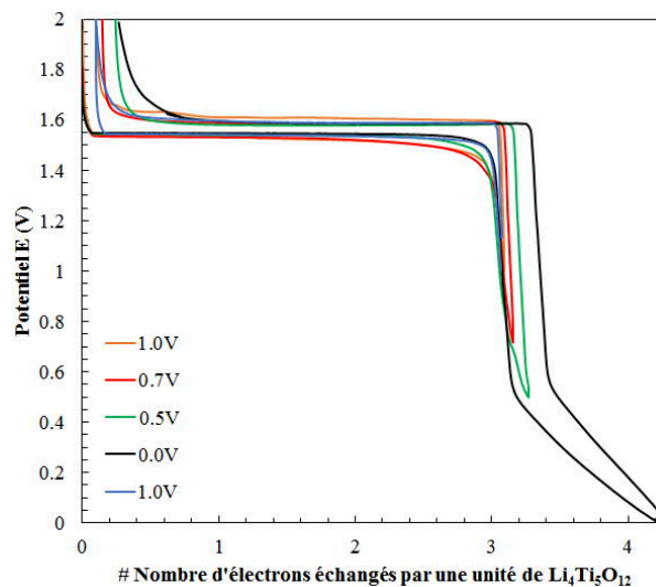
Figure 4-12 : Les 5 premiers cycles galvanostatiques de charge/décharge C/10-D/10 entre 2.0 et 1.0V (orange), entre 2.0 et 0.7V (rouge), entre 2.0 et 0.5V (vert), entre 2.0 et 0.0V (noir) et entre 2.0 et 1.0V (bleu)
