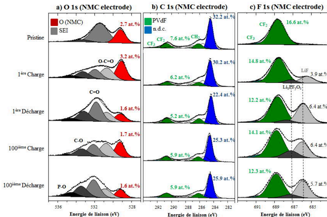
Figure 3-3 : Pics de cœur O 1s (a), C 1s de (b) et F 1s de (c) de l'électrode NMC de référence non cyclée ; des électrodes NMC cyclées en boutons complets en fin de 1ère délithiation, fin de 1ère lithiation, fin de 100ième délithiation et fin de 100ième lithiation
