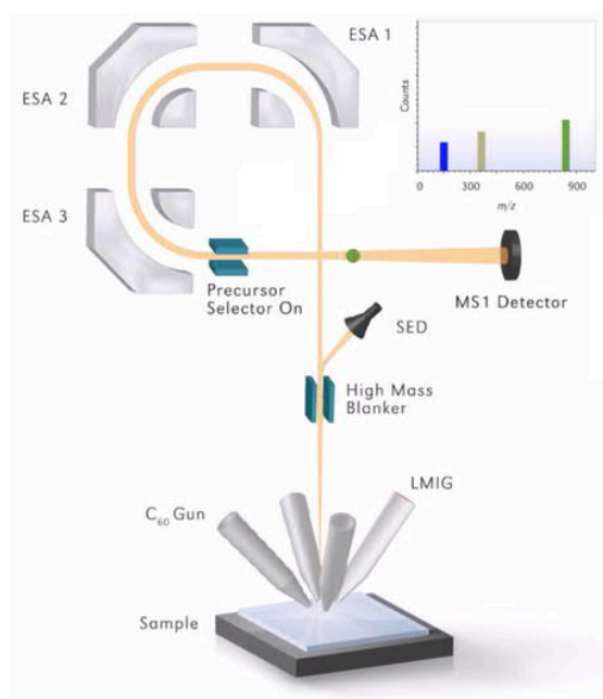
Figure 2-16 : Représentation des principaux éléments d'un spectromètre ToF-SIMS NanoToF TRIVT V de chez Physical Electronics et principe de fonctionnement d'une acquisition de spectre de masse [18]
