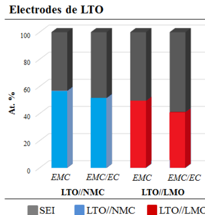
Figure 5-16 : Analyse quantitative sous forme d'historgramme via l'addition des différents pourcentages atomiques (at.%) associés aux environnements chimiques identifiés par XPS en fin de centième délithiation, à la surface des électrodes de LTO avec un électrolyte constitué d'un solvant binaire EC/EMC ou d'un mono-solvant EMC
