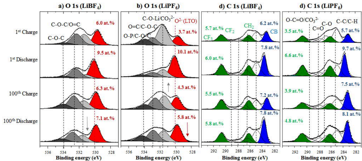
Figure 5-13 : Pics de cœur XPS O 1s et C 1s des électrodes de LTO brutes et cyclées dans un électrolyte composé du sel \text{LiBF}_4 (a et c) et \text{LiPF}_6 (b et d) en fin de 1 ère charge, fin de 1 ère décharge, fin de 100 ème charge et fin de 100 ème décharge
