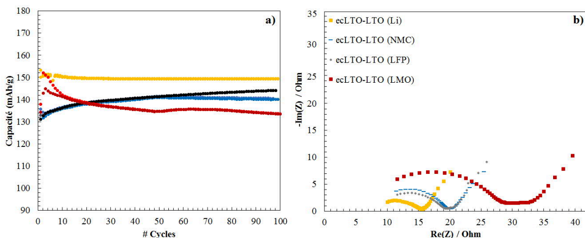
Figure 3-23 : Evolution de la capacité en fonction du nombre de cycle pour les systèmes complets LTO vs LTO avec un premier cycle effectué versus Li (jaunes), NMC (bleu et vert), LFP (gris), LMO (rouge) a). Spectroscopie d'impédance électrochimique réalisée à 25 °C au potentiel à l'abandon (OCV) à la fin du 100ème cycle de charge/décharge b)
