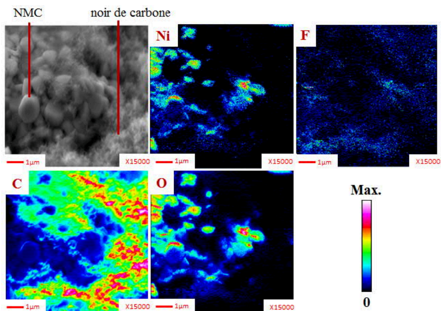
Figure 2-28 : (De gauche à droite et de haut en bas) Cliché SEM de la surface de l'électrode NMC brute non cyclée ; Cartographies chimiques réalisées par spectroscopie des électrons Auger, représentant la répartition chimique du nickel (Ni), du fluor (F), du carbone (C), et de l'oxygène (O)
