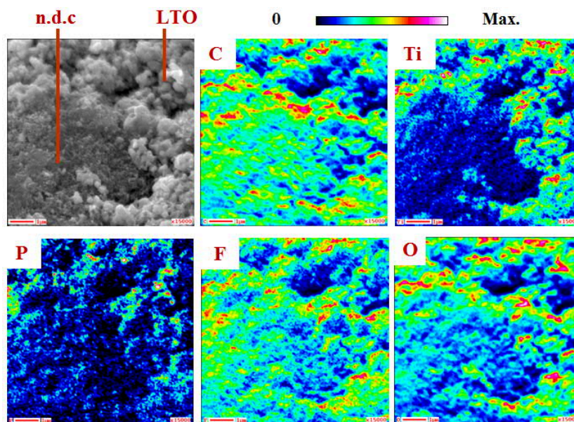
Figure 3-27 : (De gauche à droite et de haut en bas) Cliché SEM de la surface de l'électrode LTO en fin de 100 ième lithiation en symétrique avec un 1 er cycle face au lithium ; Cartographies chimiques réalisées par spectroscopie des électrons Auger, représentant la répartition chimique du carbone (C), du titane (Ti), du phosphore (P), du fluor (F) et de l'oxygène (O)
