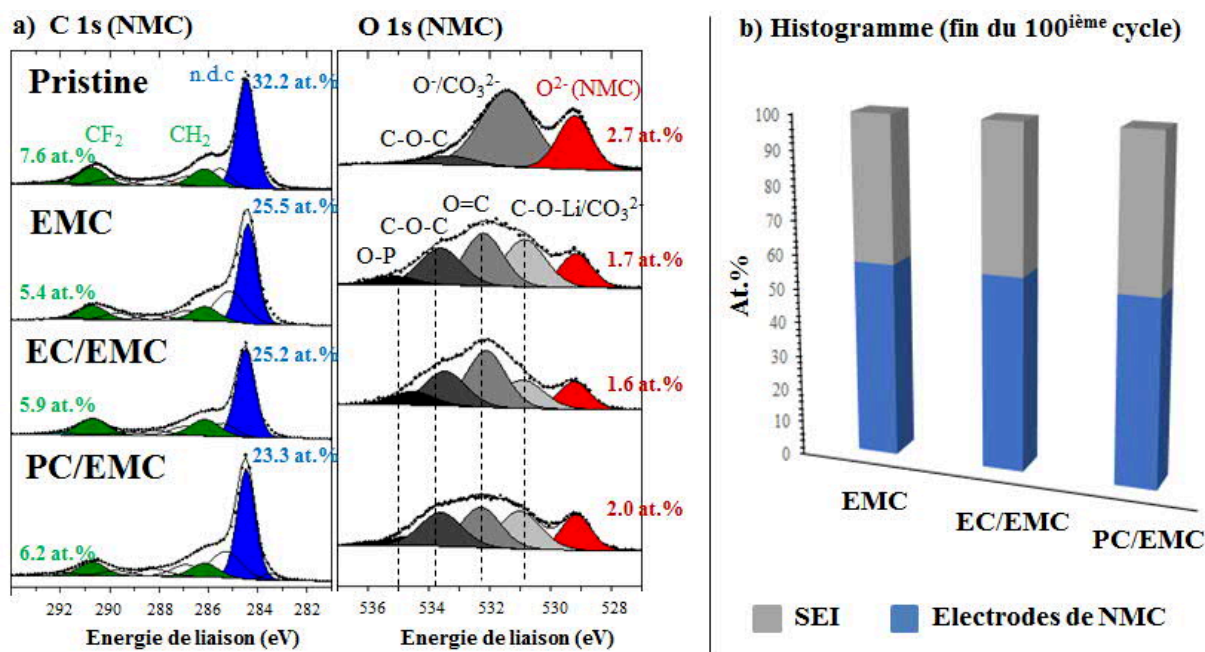
Figure 5-22 : Pics de cœur XPS C 1s et O 1s (a) et Analyse quantitative sous forme d'histogramme via l'addition des différents pourcentages atomiques (at.%) associés aux environnements chimiques identifiés par XPS à la surface des électrodes NMC, après le 100 ème lithiation, cyclées face au LTO dans un électrolyte composé de EMC (100%), EC/EMC (3:7) et PC/EMC (3:7) (b)
