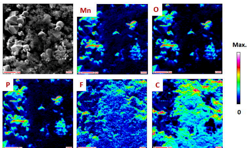
Figure 3-7 : (De gauche à droite et de haut en bas) Cliché SEM de la surface de l'électrode LMO en fin de 100 ième lithiation ; Cartographies chimiques réalisées par spectroscopie des électrons Auger, représentant la répartition chimique du manganèse (Mn), de l'oxygène (O), du phosphore (P), du fluor (F) et du carbone (C)
