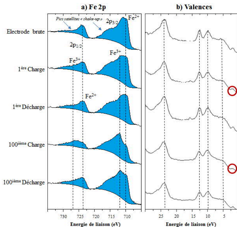
Figure 3-13 : Pics de cœur Fe 2p de (a) et de valences (b) de l'électrode LFP de référence non cyclée ; des électrodes LFP cyclées en piles complètes en fin de 1 ère délithiation, fin de 1 ère lithiation, fin de 100 ième délithiation et fin de 100 ième lithiation
