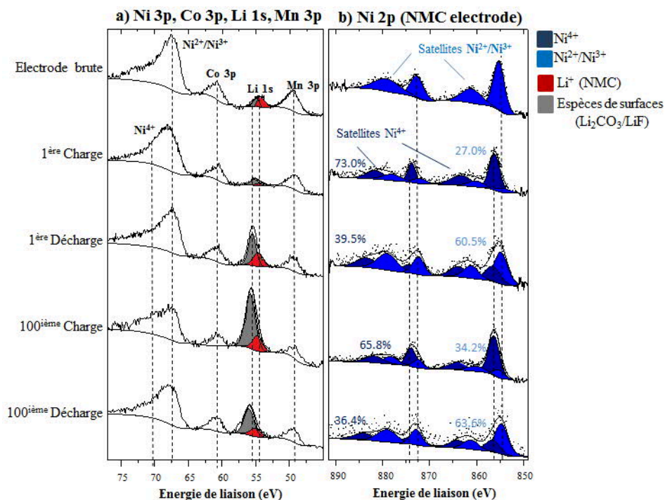
Figure 3-2 : Pics de cœur Ni 3p, Co 3p, Li 1s et Mn 3p obtenus avec une source Al (1486,6 eV) (a) et pics de cœur Ni 2p obtenus avec une source Ag (2984,3 eV) (b) de l'électrode NMC de référence non cyclée ; des électrodes NMC cyclées en piles complètes en fin de 1 ère délithiation, fin de 1 ère lithiation, fin de 100 ième délithiation et fin de 100 ième lithiation.
