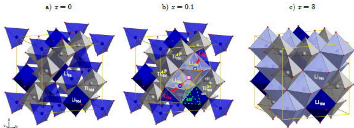
Figure 1-17 : Structure cristalline du composé \text{Li}_{4+x}\text{Ti}_5\text{O}_{12} avec x le nombre de lithium inséré ; a) avant lithiation, x = 0 ; b) en cours de lithiation, ici x = 0.1 ; c) à la fin de la lithiation, x = 3 [86]
