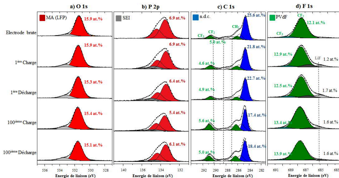
Figure 3-14 : Pics de cœur O 1s (a), pics de cœur P 2p (b), pics de cœur C 1s (c) et pics de cœur F 1s (d) de l'électrode LFP de référence non cyclée et des électrodes LFP cyclées en piles complètes en fin de 1 ère délithiation, fin de 1 ère lithiation, fin de 100 ième délithiation et fin de 100 ième lithiation
