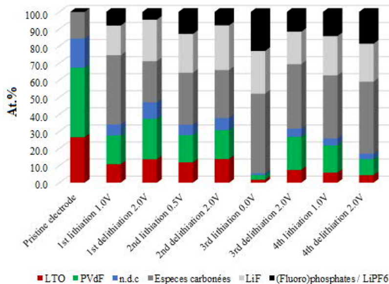
Figure 4-15 : Histogramme comparant la quantité d'espèces détectées en surface de l'électrode de LTO en fins de lithiation et délithiation au cours des 4 cycles de à formation
