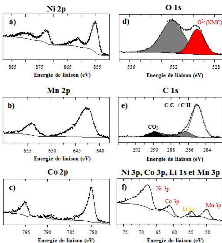
Figure 2-22 : Spectres XPS Ni 2p (a), Mn 2p (b), Co 2p (c), O 1s (d), C 1s (e) et Ni 3p, Co 3p, Li 1s et Mn 3p (f) du matériau de NMC 6/2/2
