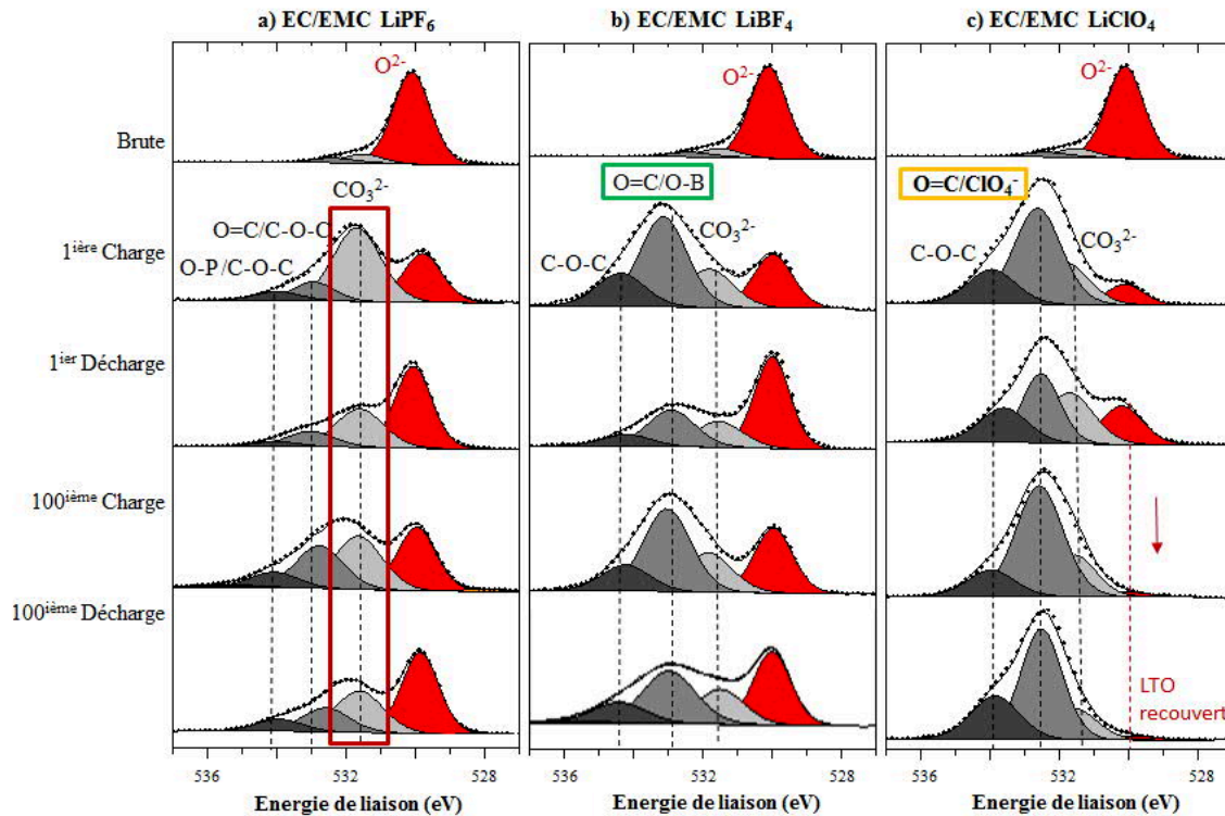
Figure 5-2 : Pics de cœur XPS O 1s de l'électrode LTO de référence non cyclée et des électrodes LTO cyclées dans un électrolyte composé du sel LiPF 6 (a), LiBF 4 (b) et LiClO 4 (c) en fin de 1ère charge, fin de 1ère décharge, fin de 100ième charge et fin de 100ième décharge
