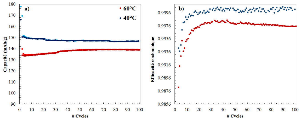
Figure 4-1 : Evolution de la capacité a) et de l'efficacité coulombique b) en fonction du nombre de cycle pour les cellules complètes LTO vs NMC cyclées à 40°C (bleu) et 60°C (rouge)
