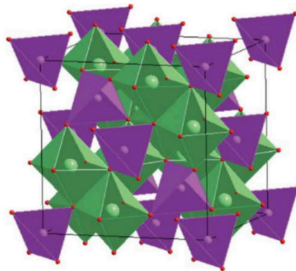
Figure 1-11 : Maille d'une structure spinelle stœchiométrique \text{LiMn}_2\text{O}_4 [51]
