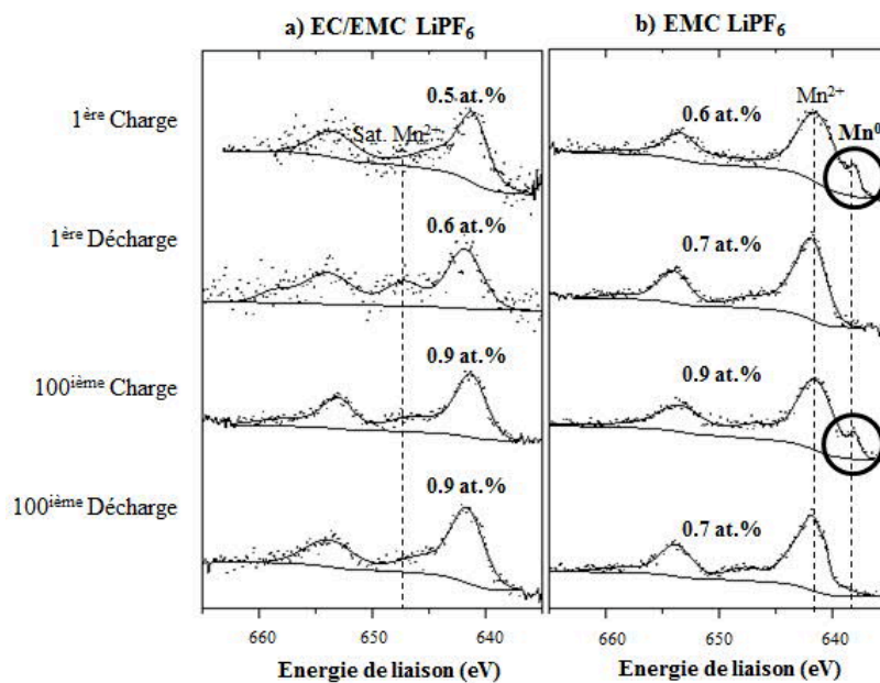
Figure 5-17 : Pics de cœur XPS Mn 2p acquis à la surface d'électrodes LTO cyclées face au LMO dans un électrolyte composé d'un solvant binaire EC/EMC (a), et d'un mono-solvant EMC (b) en fin de 1ère charge, fin de 1ère décharge, fin de 100ième charge et fin de 100ième décharge
