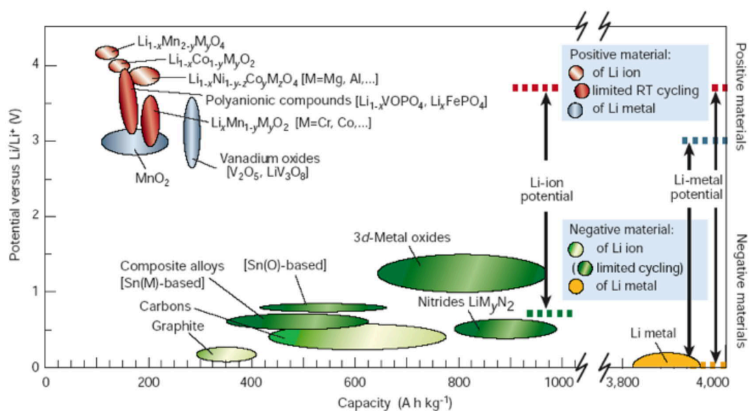
Figure 1-7 : Potentiel en fonction de la capacité pour des matériaux d'électrode [13]
