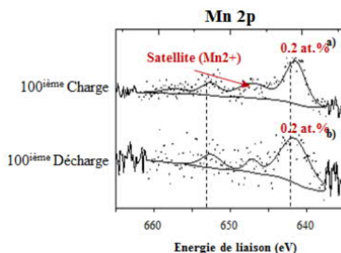
Figure 3-26 : Pics de cœur Mn 2p acquis à la surface des électrodes de LTO cyclées à 40°C à C/2 D/2 en cellules symétriques avec un premier cycle versus LMO
