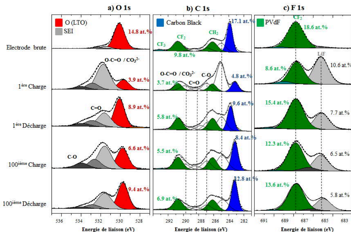
Figure 3-10 : Pics de cœur C 1s de (a) l'électrode LTO de référence non cyclée ; des électrodes LTO cyclées face au LFP en piles complètes en (b) fin de 1ère lithiation, (c) fin de 1ère délithiation, (d) fin de 100ième lithiation et (e) fin de 100ième délithiation ; pic de cœur O 1s de (f) l'électrode LTO de référence non cyclée ; des électrodes LTO cyclées en (g) fin de 1ère lithiation, (h) fin de 1ère délithiation, (i) fin de 100ième lithiation et (j) fin de 100ième délithiation ; pics de cœur F 1s de (k) l'électrode LTO de référence non cyclée ; des électrodes LTO cyclées en (l) fin de 1ère lithiation, (m) fin de 1ère délithiation, (n) fin de 100ième lithiation et (o) fin de 100ième délithiation
