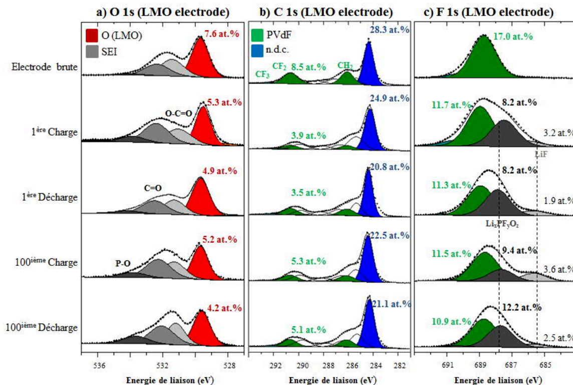
Figure 3-6 : Pics de cœur O 1s (a), pic de cœur C 1s de (b) et pics de cœur F 1s de (c) de l'électrode LMO de référence non cyclée ; des électrodes LMO cyclées en boutons complets en fin de 1 ère délithiation, fin de 1 ère lithiation, fin de 100 ième délithiation et fin de 100 ième lithiation
