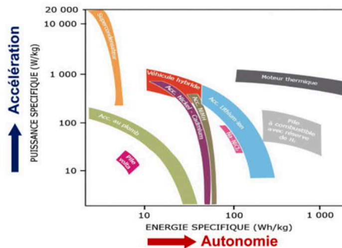
Figure 1-4 : Diagramme de Ragone de différents dispositifs de stockage
