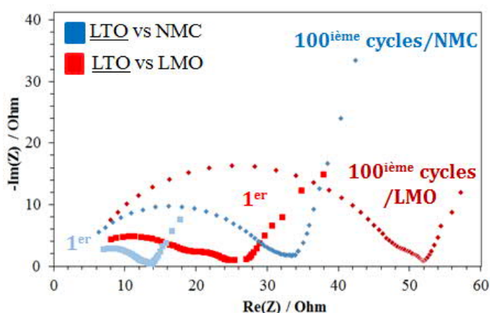
Figure 3-1 : Spectroscopie d'impédance électrochimique réalisée à 25 °C au potentiel à l'abandon (OCV) à la fin du 1 er et du 100 ième cycles de charge/décharge sur les systèmes LTO vs NMC (bleus) et LTO vs LMO (rouges)
