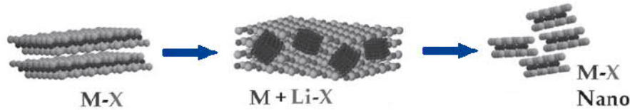
Figure 1-20 : Schéma d'une réaction de conversion inspiré de la référence [100]
