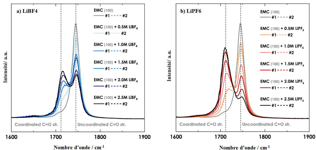
Figure 5-9 : Spectres FT-IR (1600–1900 cm -1 ) de LiBF 4 :EMC (a) et LiPF 6 :EMC (b) dans différente molarité
