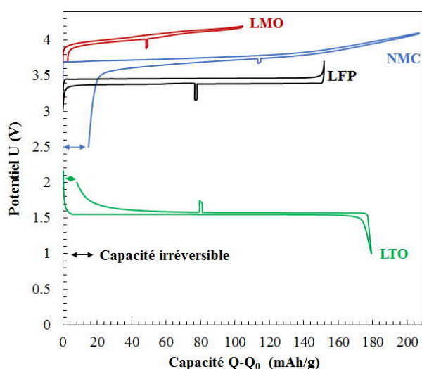
Figure 2-5 : Profils de charge et de décharge d'accumulateurs LTO/Li, LFP/Li, NMC/Li et LMO/Li utilisant un électrolyte à solvant binaire EC/EMC (3:7) et \text{LiPF}_6 (1M) au 1 er cycle aux régimes C/10 :D/10 à 60,0 \pm 0,5^\circ\text{C}
