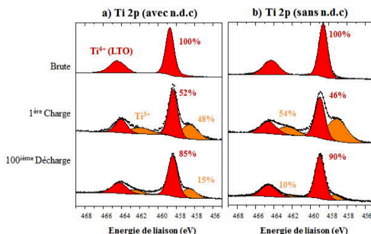
Figure 5-24 : Pics de cœur XPS Ti 2p des électrodes brutes de LTO non cyclées (1 ère ligne) et des électrodes de LTO cyclées à 40°C à C/2 D/2 en cellules complètes LTO//NMC à la fin de la 1 ère charge (2 ème ligne) et de la 100 ème décharge (3 ème ligne), avec a) et sans noir de carbone b)
