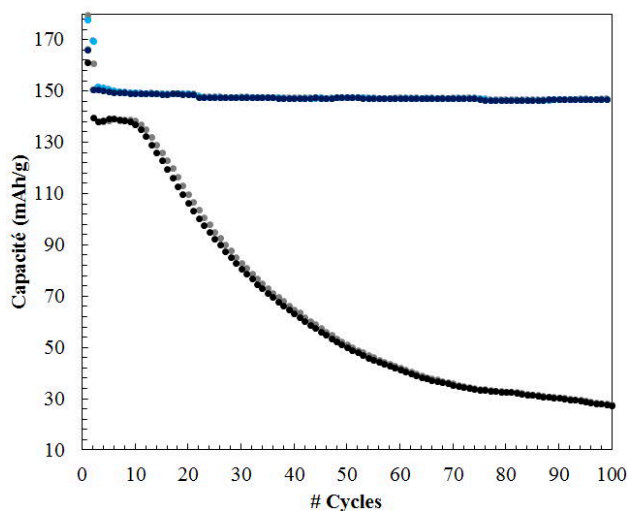
Figure 3-17 : Evolution des capacités en fonction du nombre de cycles pour les boutons complets en charge (bleu clair) et décharge (bleu foncé) ; et pour les bi-boutons en charge (gris) et décharge (noir)
