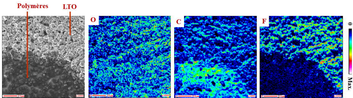
Figure 4-21 : (De gauche à droite) Cliché SEM de la surface de l'électrode LTO en fin de 30 ième délithiation en demi-pile ; Cartographies chimiques réalisées par spectroscopie d'électrons Auger, représentant la répartition chimique de l'oxygène (O), du carbone (C) et du fluor (F)
