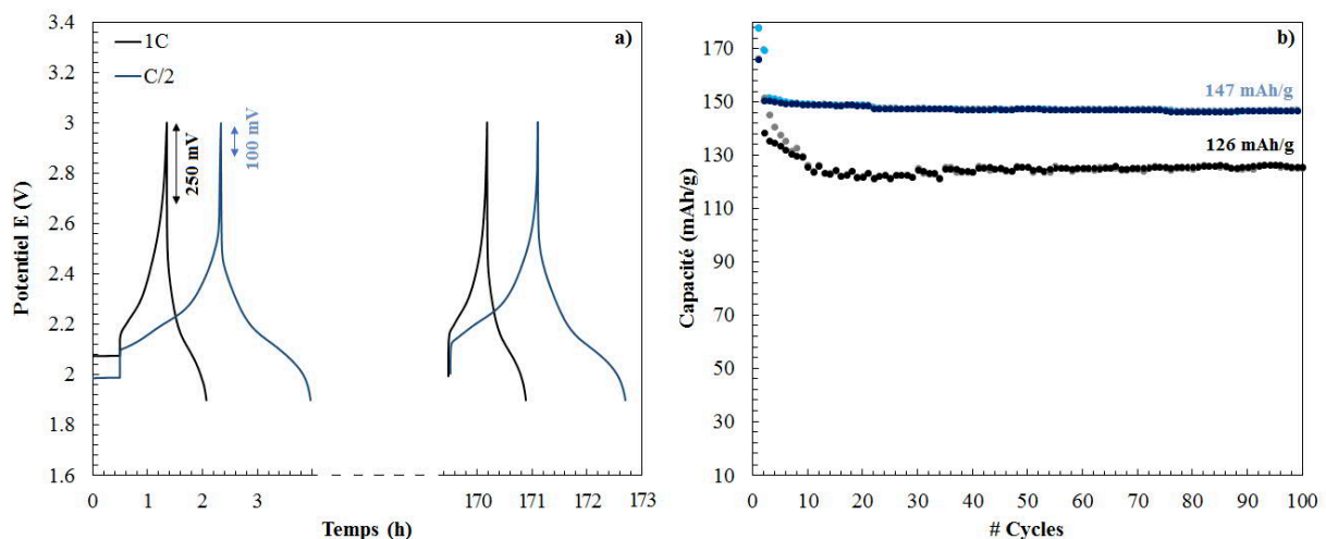
Figure 4-8 : Courbes de cyclage galvanostatique à régimes de charge/décharge C/2-D/2 (bleu) et C/1-D/1 (noir) à 40°C en fonction du temps de cyclage a). Evolution de la capacité en fonction du nombre de cycle pour les cellules complètes LTO vs NMC cyclées à régimes de charge/décharge C/2-D/2 (bleu) et C/1-D/1 (noir) b)
