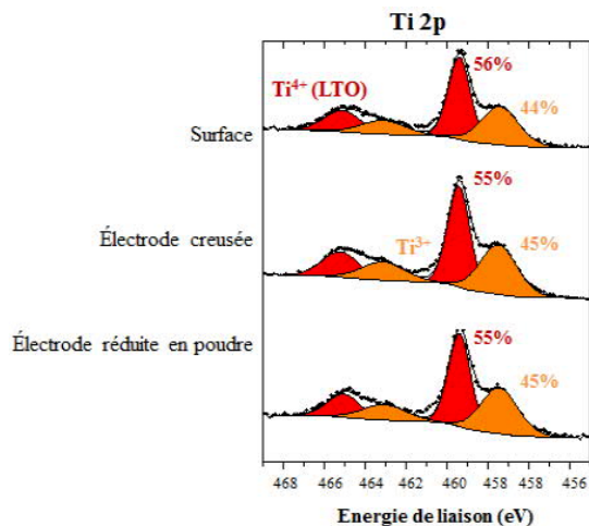
Figure 5-25 : Pics de cœur XPS Ti 2p d'électrodes de LTO lithiées à 40°C à C/2 D/2 en cellules complètes LTO//NMC, avec noir de carbone en surface b)
