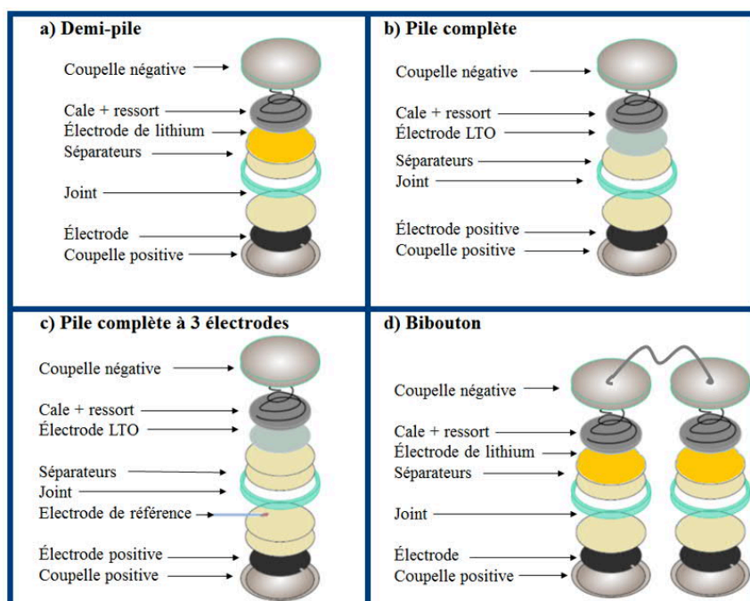
Figure 2-4 : Schéma des différents montages en bouton réalisés au cours des travaux de thèse
