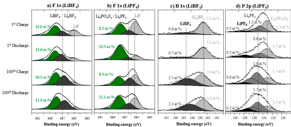
Figure 5-12 : Pics de cœur XPS F 1s, B 1s et P 2p des électrodes de LTO cyclées dans un électrolyte composé du sel \text{LiBF}_4 (a et c) et \text{LiPF}_6 (b et d) en fin de 1 ère charge, fin de 1 ère décharge, fin de 100 ième charge et fin de 100 ième décharge
