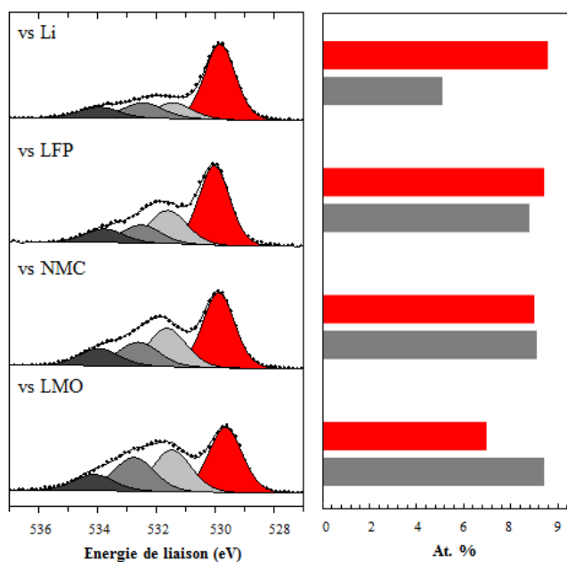
Figure 3-25 : (a) Pics de cœur O 1s des électrodes de LTO, à l'état déchargé, cyclées à 40°C à C/2 D/2 en cellules symétriques avec un premier cycle versus Lithium versus LFP, versus NMC et versus LMO et (b)
