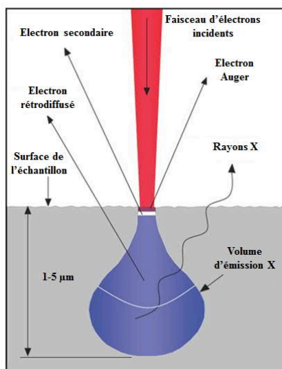
Figure 2-11 : Représentation des différentes zones d'émission lors de l'interaction électron-matière
