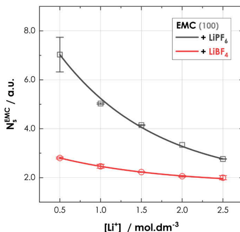
Figure 5-10 : Evolution du nombre de solvation en fonction de la concentration de LiBF 4 (rouge) et de LiPF 6 (noir) selon les mesures FT-IR
