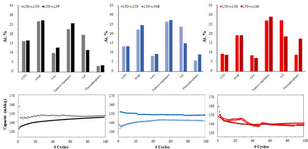
Figure 3-28 : Analyse XPS quantitative sous forme d'histogrammes des électrodes de LTO cyclées en complets face au LFP, NMC et LMO et en symétriques ; et évolutions des capacités au cours des cycles associés
