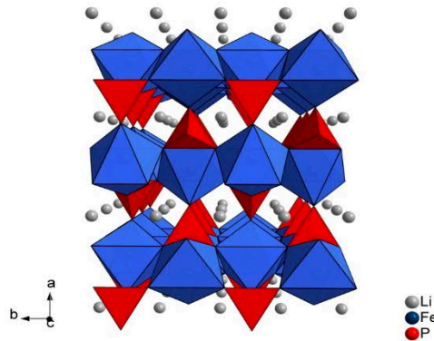
Figure 1-13 : Structure cristallographique du LFP [24]
