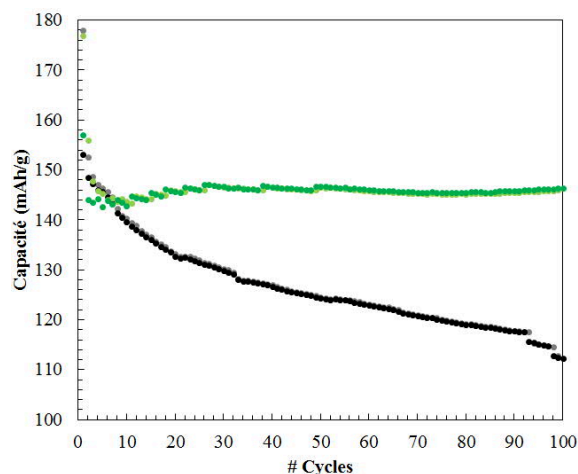
Figure 3-15 : Evolution de la capacité en fonction du nombre de cycle pour les systèmes complets LTO vs LFP (gris et noir), LTO vs LFP industriel (vert clair et vert foncé)
