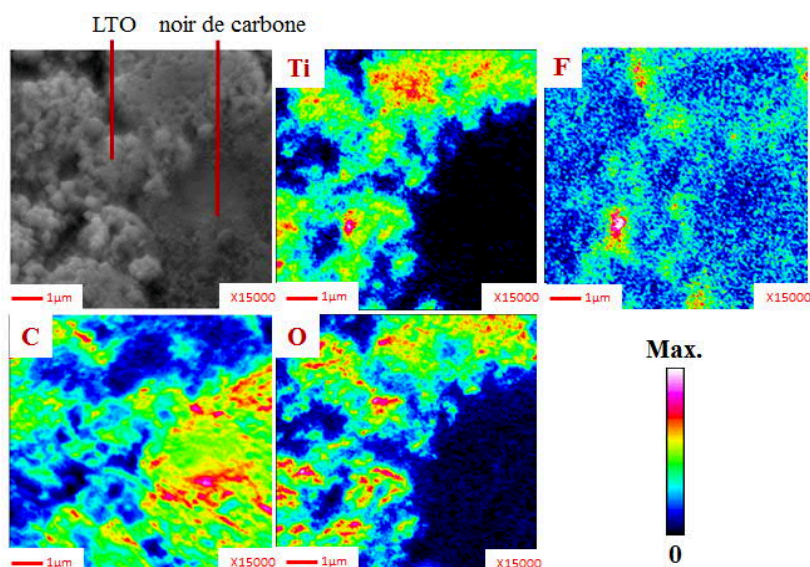
Figure 2-25 : (De gauche à droite et de haut en bas) Cliché SEM de la surface de l'électrode LTO brute non cyclée ; Cartographies chimiques réalisées par spectroscopie des électrons Auger, représentant la répartition chimique du titane (Ti), du fluor (F) du carbone (C), et de l'oxygène (O)
