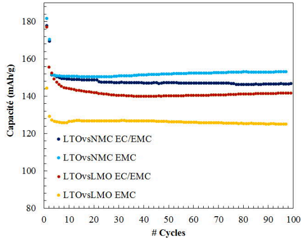
Figure 5-14 : Evolution de la capacité au cours du cyclage des cellules LTO//NMC et LTO//LMO avec un électrolyte constitué de solvant binaire EC/EMC (bleu foncé et rouge) et de mono solvant EMC (bleu clair et jaune)
