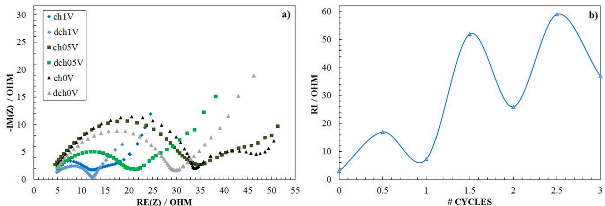
Figure 4-13 : Spectroscopie d'impédance électrochimique réalisée à 25 °C au potentiel à l'abandon (OCV) à l'état lithié et délithié après cyclage a), Evolution de l'impédance (réelle) totale du système LTO//Li au cours des trois premiers cycles b)
