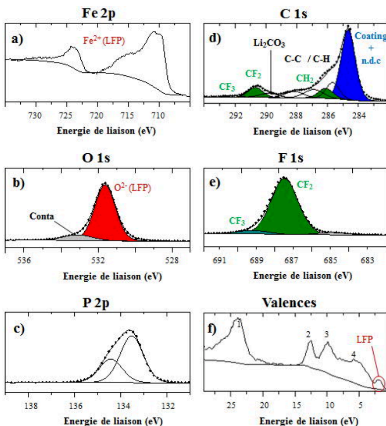
Figure 2-33 : Pics de cœur Fe 2p (a), O 1s (b), P 2p (c), C 1s (d), F 1s (e) et spectres de valences (f) de l'électrode de référence de LFP
