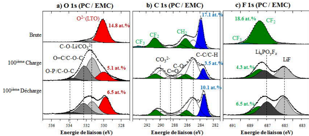
Figure 5-19 : Pics de cœur XPS O 1s a), C 1s b) et F 1s c) de l'électrode LTO de référence non cyclée et des électrodes LTO cyclées face au NMC dans un électrolyte composé de PC/EMC (3:7) LiPF 6 (1M), en fin de 100 ème charge et fin de 100 ème décharge
