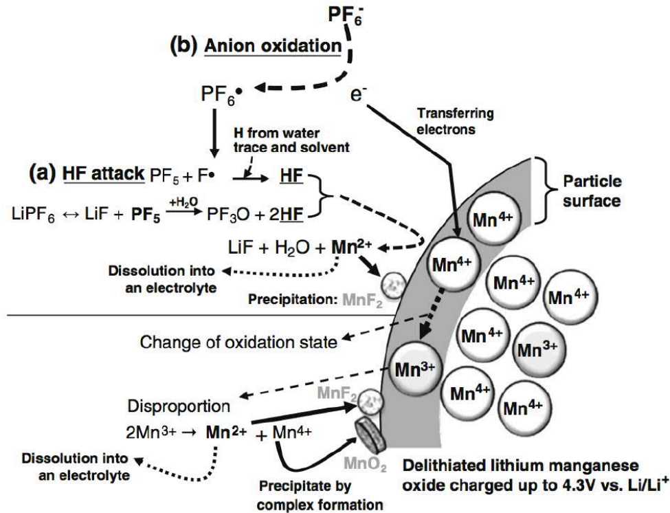
Figure 1-28 : Dissolution du manganèse et modification de surface à partir d'une électrode délithiée par (a) attaque acide de HF et (b) oxydation de l'anion \text{PF}_6^- mises en évidence par DRX, FTIR et ICP (issu de la publication de Choi et al. [61])
