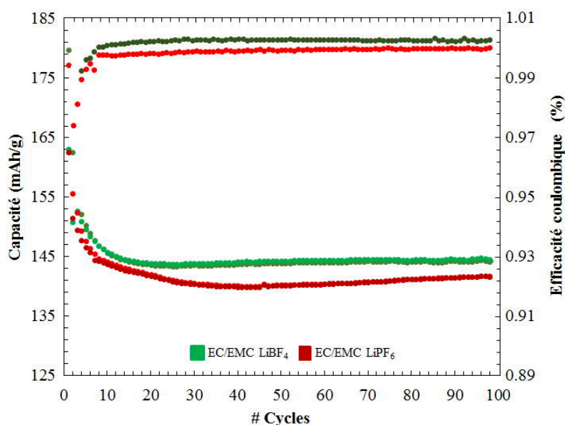
Figure 5-8 : Evolution de la capacité en fonction du nombre de cycle et efficacités coulombiques du système LTO//LMO testé avec deux électrolytes LiPF 6 :EC:EMC (rouge) and LiBF 4 :EC:EMC (vert)
