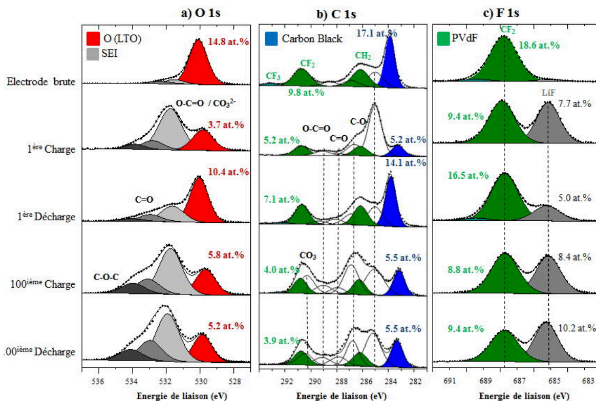
Figure 3-18 : Pics de cœur O 1s (a), pics de cœur C 1s (b) et pics de cœur F 1s (c) l'électrode LTO de référence non cyclée et des électrodes LTO cyclées en bi-boutons face au NMC en fin de 1 ère délithiation, fin de 1 ère lithiation, fin de 100 ième délithiation et fin de 100 ième lithiation
