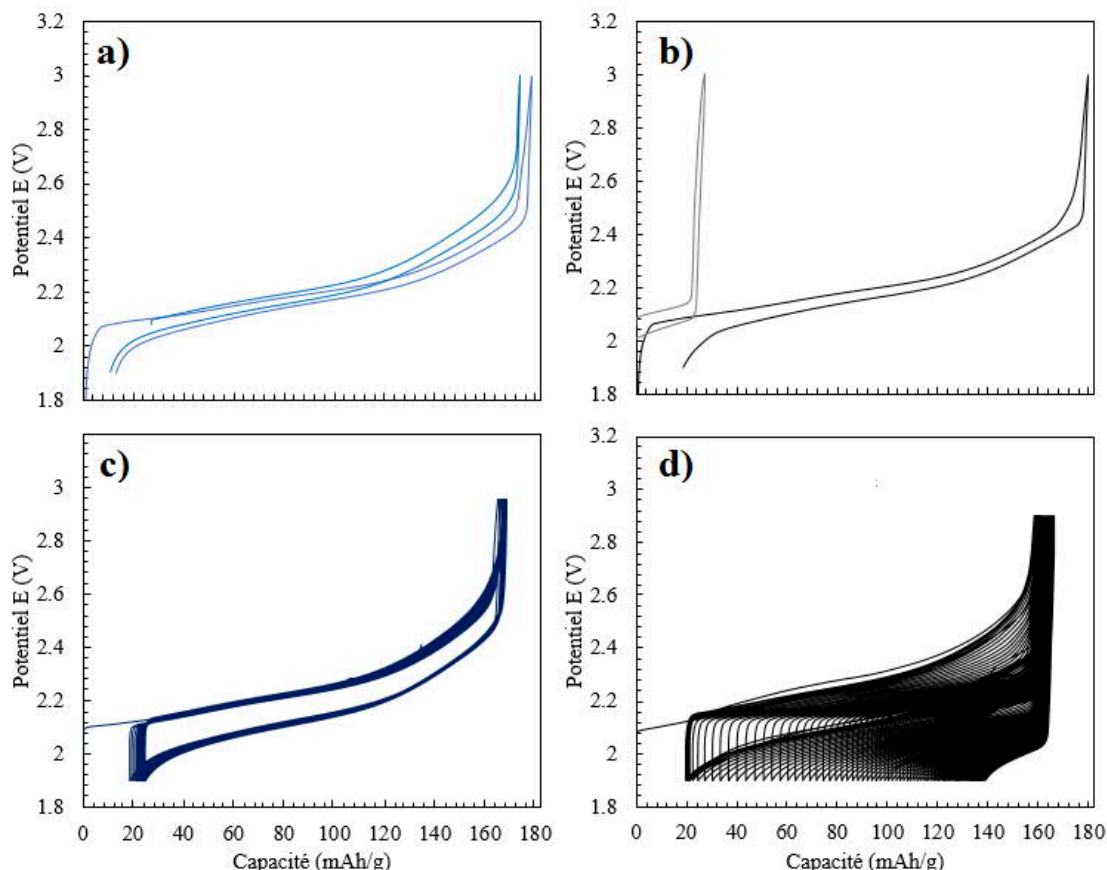
Figure 3-16 : Cyclages galvanostatiques des boutons complets (à droite) et des bi-boutons (à gauche), cycles de formation (bleu et noir) à 60°C et C/10 et cycle de fin (bleus clairs et gris) à 40°C et C/10 (a) et (b), cyclages (bleus foncés et noirs) à 40°C et C/12 (c) et (d)
