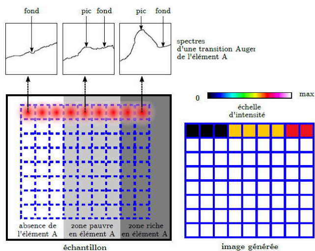
Figure 2-15 : Schéma de principe de l'acquisition d'une cartographie élémentaire SAM [16]
