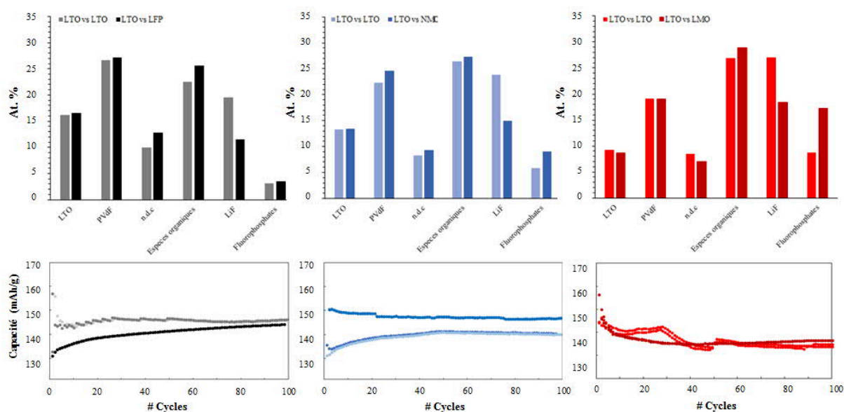
Figure 3-28 : Analyse XPS quantitative sous forme d'histogrammes des électrodes de LTO cyclées en complets face au LFP, NMC et LMO et en symétriques ; et évolutions des capacités au cours des cyclages associés
