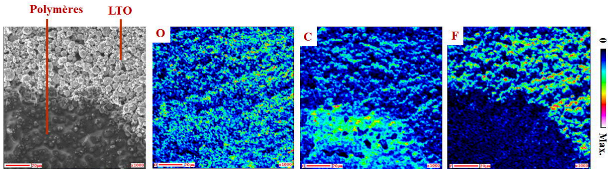
Figure 4-21 : (De gauche à droite) Cliché SEM de la surface de l'électrode LTO en fin de 30 ième délithiation en demi-pile ; Cartographies chimiques réalisées par spectroscopie d'électrons Auger, représentant la répartition chimique de l'oxygène (O), du carbone (C) et du fluor (F)
