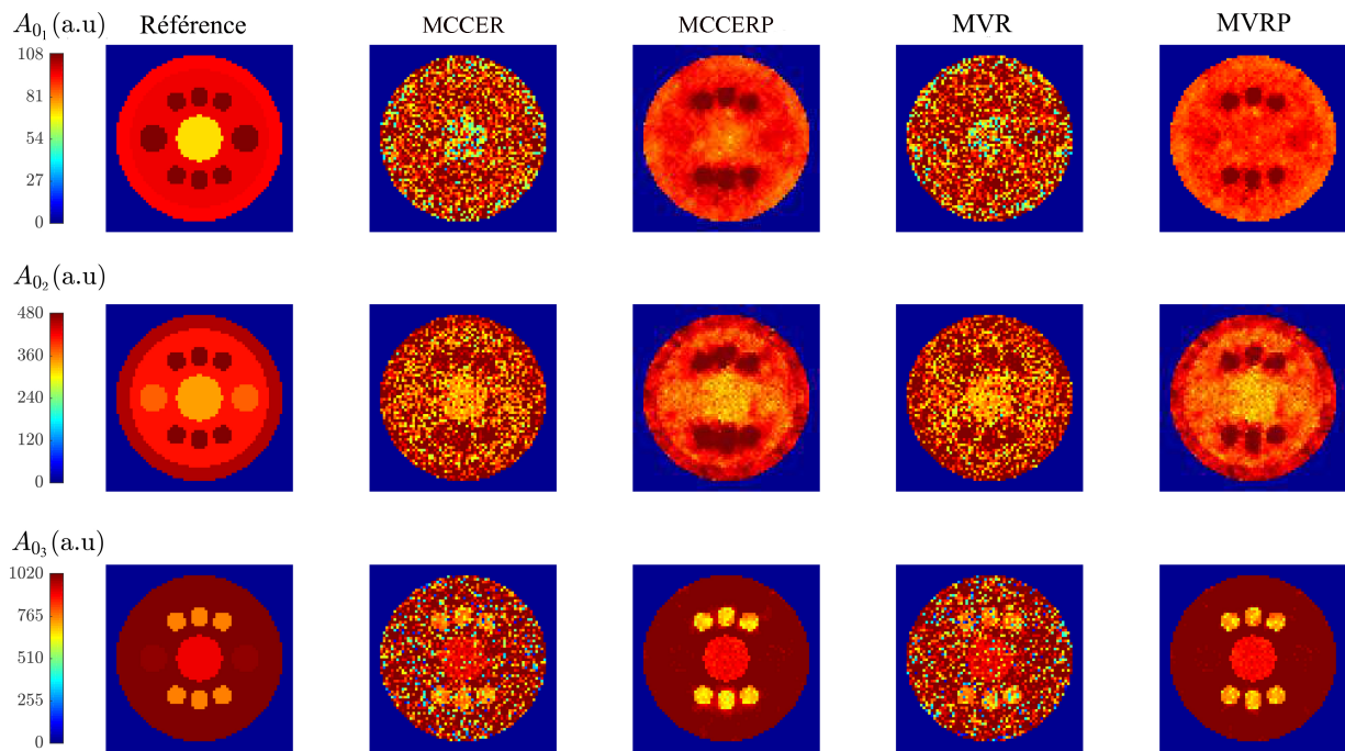
Figure IV.5 – Cartographies d’intensit s reconstruites pour les composantes   d croissance rapide (premi re ligne),   d croissance moyenne (deuxi me ligne) et   d croissance lente (troisi me ligne). Les cartographies de r f rence (premi re colonne) sont compar es aux cartographies estim es par MCCER (deuxi me colonne), MCCERP (troisi me colonne), MVR (quatri me colonne) et MVRP (cinqui me colonne).
