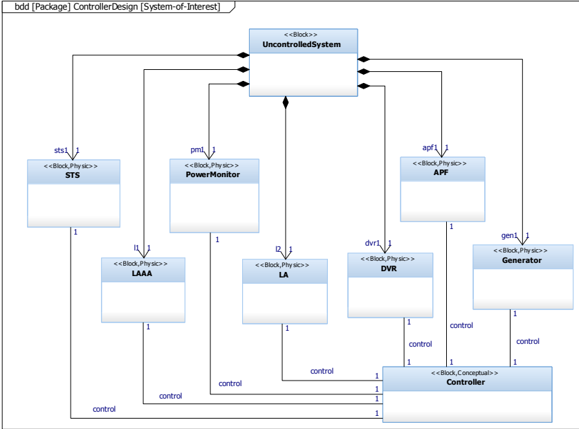
Figure C.19 BDD: Structure du système
