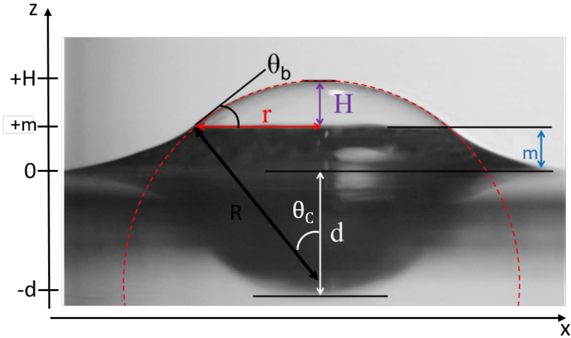
FIGURE 2.4 – Adaptée de [38]. Image d'une bulle à la surface d'un bain liquide, avec les notations utilisées ici. L'axe vertical est noté z et horizontal x . \theta_b est l'angle entre l'horizontale et la tangente au profil de la calotte sphérique en haut du ménisque, \theta_c , l'angle entre la verticale et le segment qui relie le centre de courbure de la calotte sphérique avec le haut du ménisque, H est la hauteur de la calotte sphérique, m celle du ménisque. d est la profondeur de la cavité sous la surface. R est le rayon de la calotte sphérique et r le rayon du cercle défini par le sommet du ménisque.
