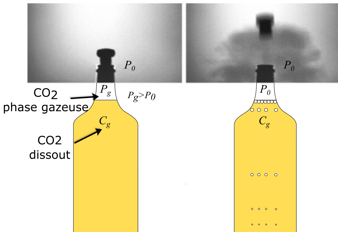
FIGURE 7.3 – Schéma de principe d'un équilibre CO 2 -H 2 O (figure de gauche) et rupture de cet équilibre qui conduit à la génération de bulles (figure de droite). Les photos sont issues de Liger-Belair [13]. Elles sont réalisées à l'aide d'un corps noir comme source d'infrarouge derrière la bouteille et d'une caméra équipée d'un filtre passe-bande centré sur la raie d'absorption du CO 2 à 4,245 \mu\text{m} , de façon à visualiser la dynamique du gaz lorsque la bouteille est ouverte.
