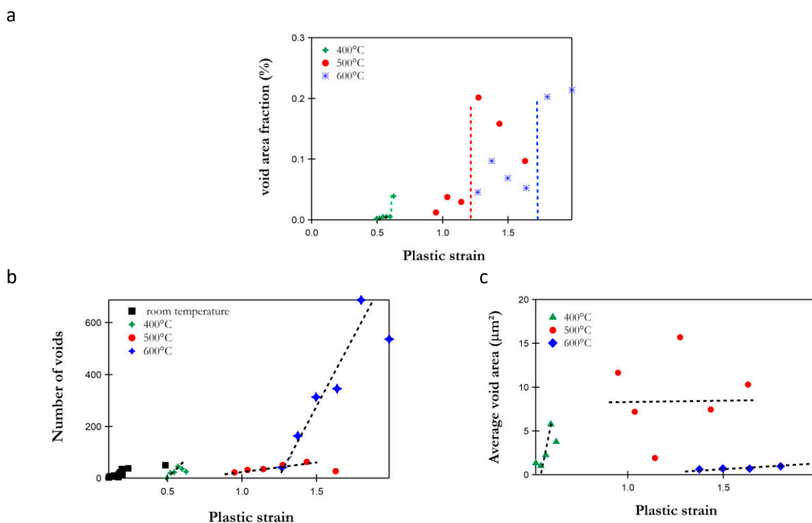
Figure III-3. Evolution (a) de la fraction surfacique des vides, (b) du nombre de vides, et (c) de la croissance des vides en fonction de la déformation plastique pour les éprouvettes de traction ( \eta = 0,33 ).
