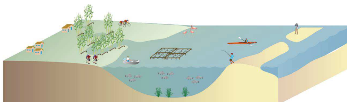
Figure 9 : quelques services écosystémiques fournis par une lagune côtière/ © Sy Mariam Maki.
