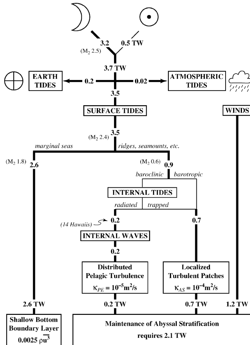
FIGURE 9.1 – Bilan énergétique sur l’océan proposé par Munk and Wunsch [1998]. Ce bilan prend comme sources d’excitation les marées (la contribution de l’harmonique M 2 de marée est notée en italique) et le vent, et évalue les différentes dissipations de cette énergie entre deux réservoirs : l’énergie cinétique dans les couches peu profondes de l’océan et le mélange turbulent qui permet le maintien de la stratification.
