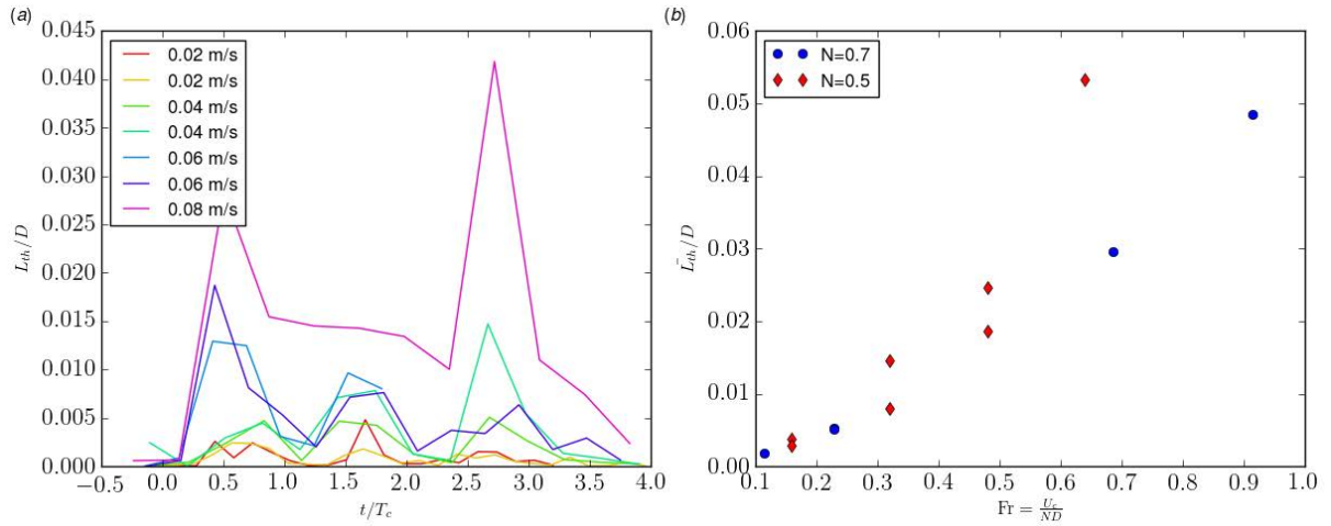
FIGURE 8.13 – Évolution de l'échelle de Thorpe avec la vitesse de la grille. a) Évolution temporelle de L_T pour différentes vitesses de grille à N = 0.5 rad/s. b) Variation de l'échelle moyenne de Thorpe avec la vitesse de grille pour différents N = 0.7 rad/s et N = 0.5 rad/s.
