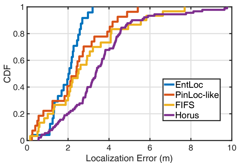
Figure 3: Précision de la localisation de l'EntLoc proposé par rapport à l'état de l'art.
