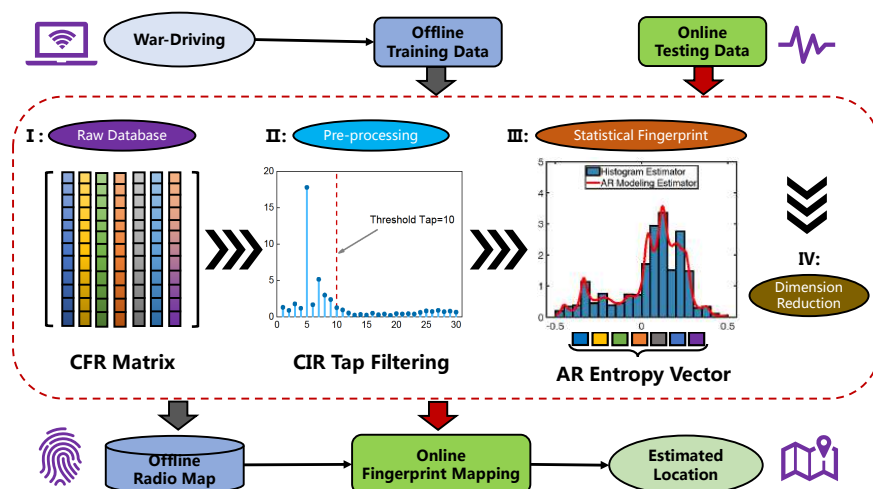
Figure 1: L'architecture du système EntLoc.
