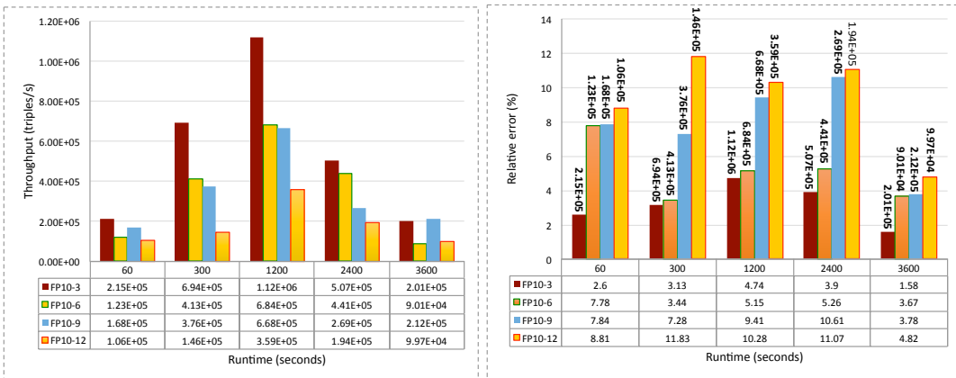
FIGURE 9.14 – Débit avec une probabilité de FP variable.
