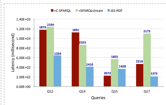
FIGURE 9.9 – Comparaison de latence entre systèmes JSS-RDF et ≈RSP.
