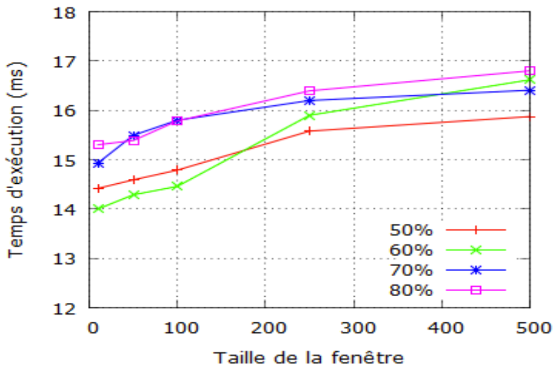
FIGURE 4.8 – Chaîne.
