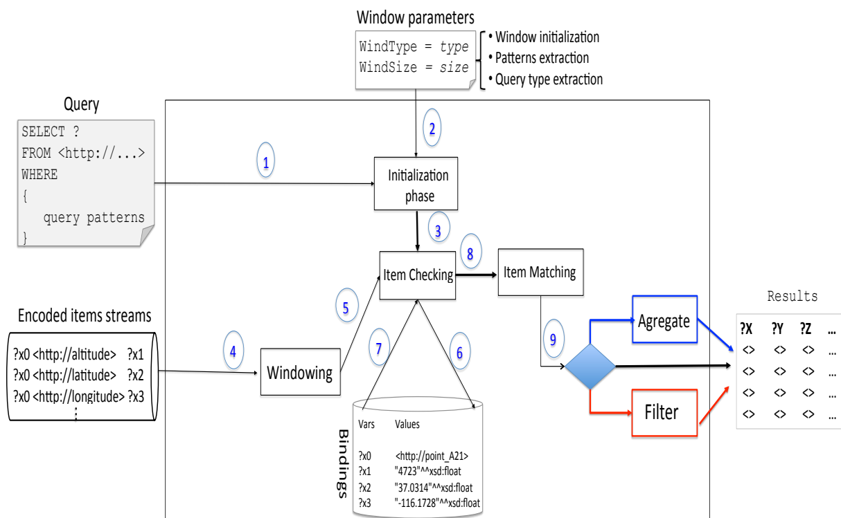
FIGURE 6.3 – Architecture de traitement optimisé de flux de données RDF compressées au format RDSZ.
