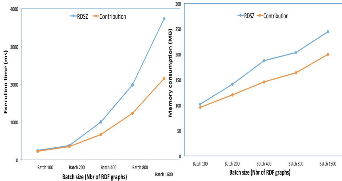
FIGURE 6.5 – Évaluation de la consommation de mémoire d'une requête SPARQL.
