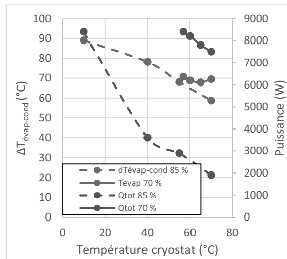
Figure 180 : \Delta T_{\text{évap-cond}} et puissance avant assèchement en fonction de la température de source froide pour TR = 70 % et TR = 85 % (pentane)
