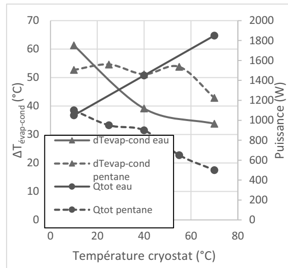
Figure 186 : \Delta T_{\text{évap-cond}} et puissance avant assèchement en fonction de la température de source froide ( TR = 50\% )
