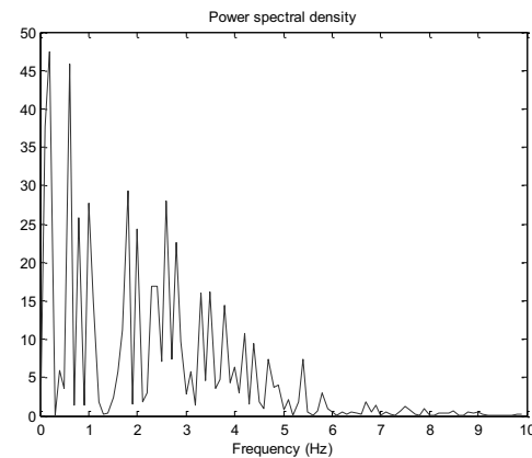
Figure 150 : Densité spectrale de puissance de la température adiabatique (Area 3) mesurée par visualisation IR (eau, TR = 50\% , T_{cryo} = 40^{\circ}C , Q = 4500\ W )
