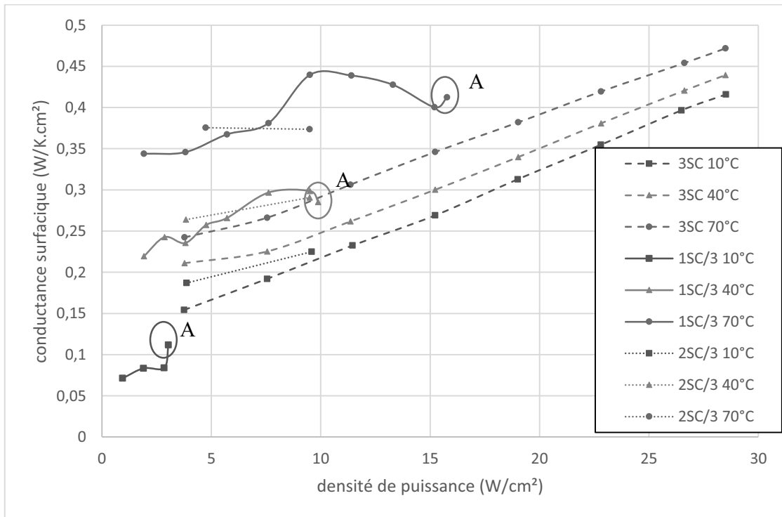
Figure 199 : Conductance surfacique en fonction de la densité de puissance pour différents dispositifs et différentes températures de source froide (méthanol, TR = 50\% )
