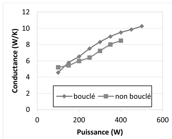
Figure 78 : Conductance globale en fonction de la puissance injectée pour une configuration bouclée et non-bouclée (éthanol, TR = 40\% , T_{cryo} = 10^\circ\text{C} , horizontale)
