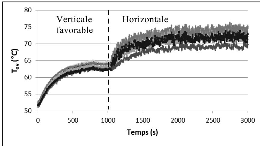
Figure 98 : Réponse thermique du PHP à un changement d'orientation de verticale favorable à horizontale (pentane, TR = 40\% , T_{cryo} = 40^{\circ}\text{C} , Q = 150\text{ W} )
