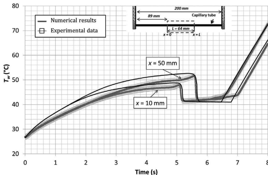
Figure 20 : Comparaison entre numérique et expérience de la température de paroi en fonction du temps (26)
