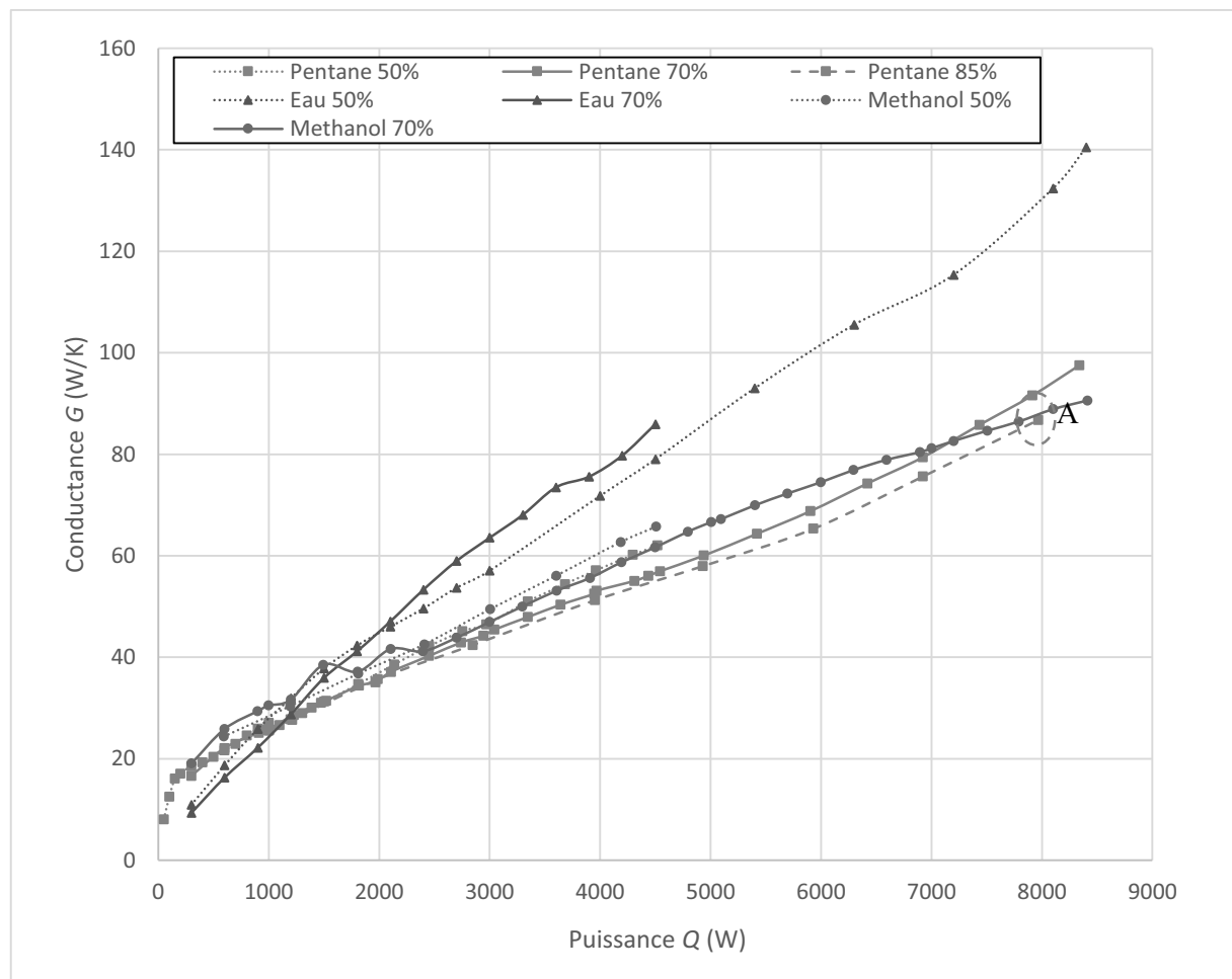
Figure 166 : Conductance en fonction de la puissance pour les trois fluides ( T_{cryo} = 10^\circ\text{C} )
