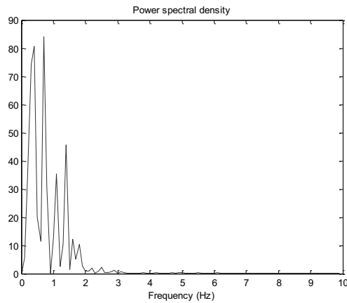
Figure 173 : Densité spectrale de puissance de la température évaporateur (Area 1) mesurée par visualisation IR (eau, TR = 50\% , T_{cryo} = 10^{\circ}\text{C} , Q = 600\text{ W} )
