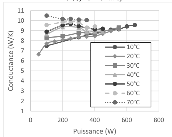
Figure 83 : Conductance globale en fonction de la puissance pour différentes températures de source froide (pentane, TR = 40\% , verticale favorable)
