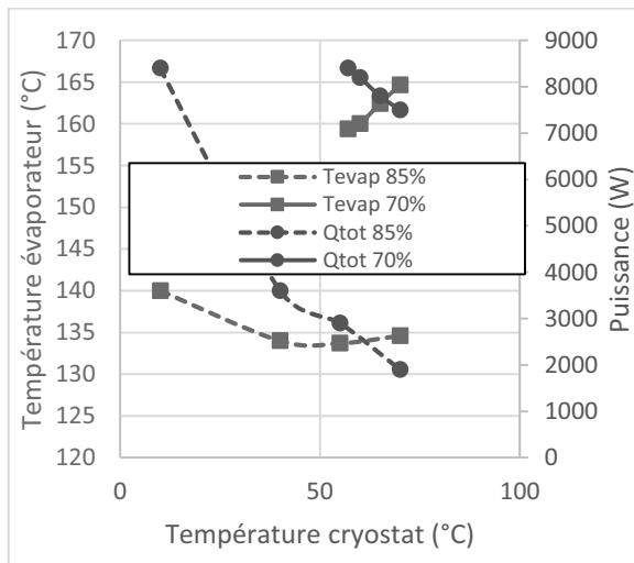
Figure 179 : Température et puissance avant assèchement en fonction de la température de source froide pour TR = 70 % et TR = 85 % (pentane)
