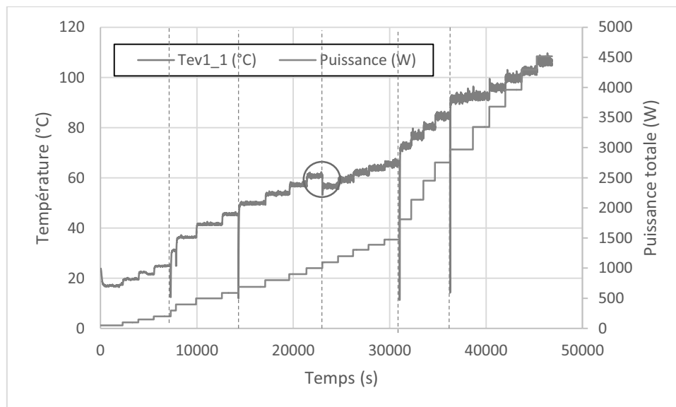
Figure 151 : Evolution de la température durant un essai typique (pentane, TR = 50\% , T_{cryo} = 10^{\circ}\text{C} )
