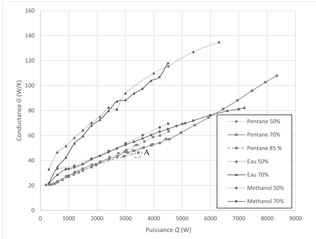
Figure 167 : Conductance en fonction de la puissance pour les trois fluides ( T_{cryo} = 40^{\circ}\text{C} )
