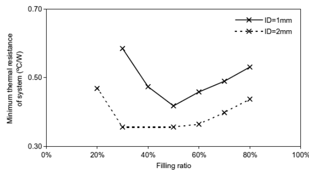
Figure 44 : Evolution de la résistance thermique minimum en fonction du taux de remplissage pour deux diamètres différents (52)
