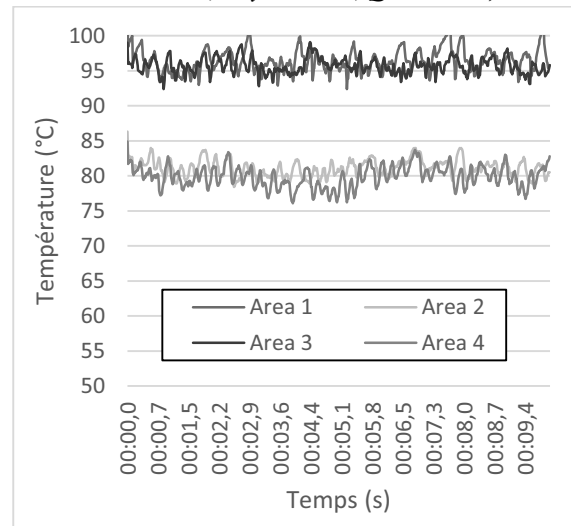
Figure 142 : Evolution temporelle de la température mesurée par visualisation IR (eau, TR = 50 \% , T_{cryo} = 40^{\circ}\text{C} , Q = 4500 \text{ W} )
