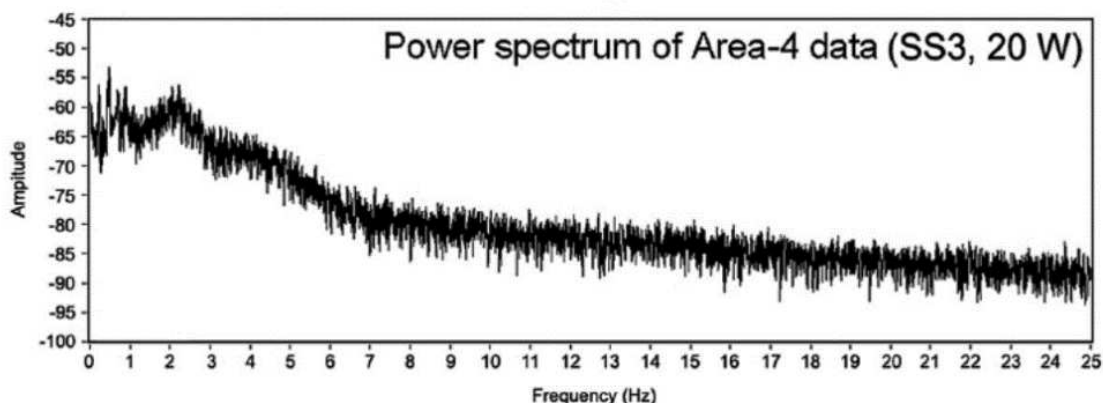
Figure 66 : Densité de puissance spectrale pour l'état SS3 (10)
