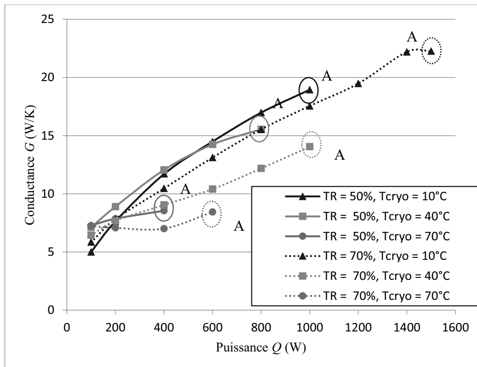
Figure 160 : Conductance en fonction de la puissance injectée pour différents taux de remplissage (pentane, dispositif 1SC)
