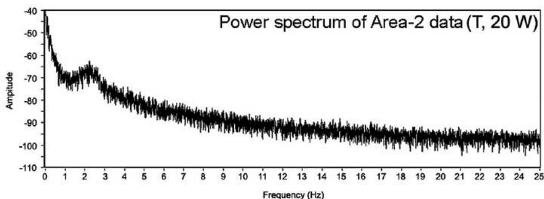
Figure 67 : Densité de puissance spectrale pour l'état T (10)
