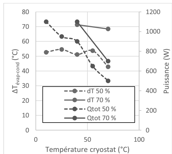
Figure 184 : \Delta T_{\text{évap-cond}} et puissance avant assèchement en fonction de la température de source froide pour TR = 50\% et TR = 70\% (pentane)
