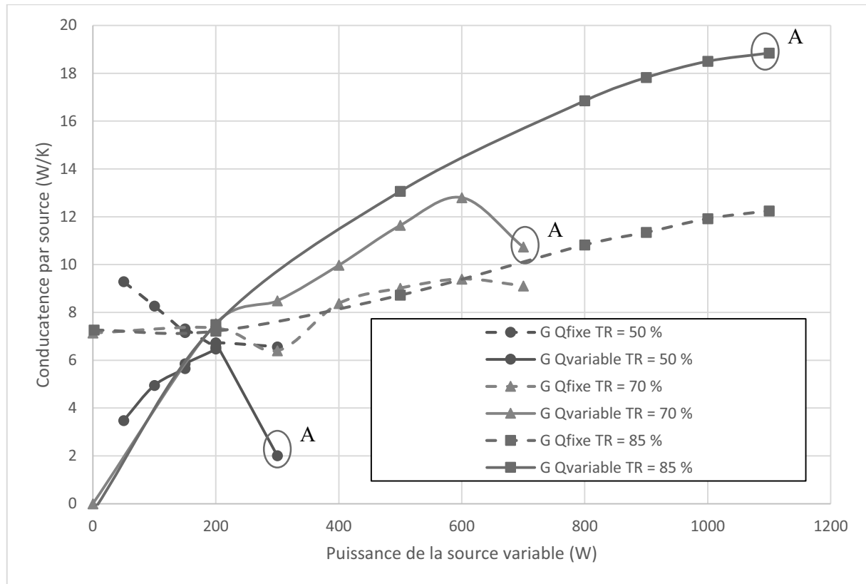
Figure 216 : Conductance par source en fonction de la puissance variable (pentane, T_{cryo} = 40^{\circ}\text{C} , Q_{fixe} = 200 \text{ W} )
