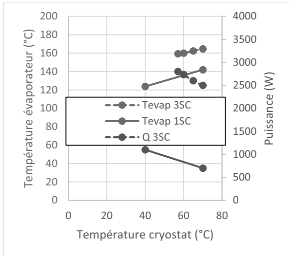
Figure 181 : Température et puissance avant assèchement en fonction de la température de source froide pour deux dispositifs (pentane, TR = 70\% )
