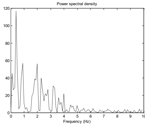
Figure 148 : Densité spectrale de puissance de la température évaporateur (Area 1) mesurée par visualisation IR (eau, TR = 50\% , T_{cryo} = 40^{\circ}C , Q = 4500\ W )
