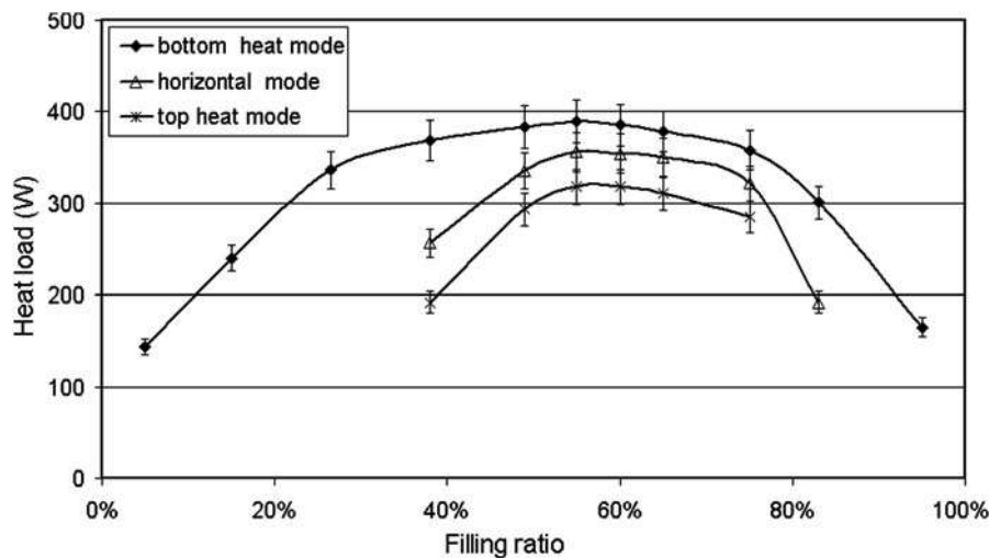
Figure 45 : Evolution de la puissance maximale transférée en fonction du taux de remplissage pour trois orientations différentes (63)
