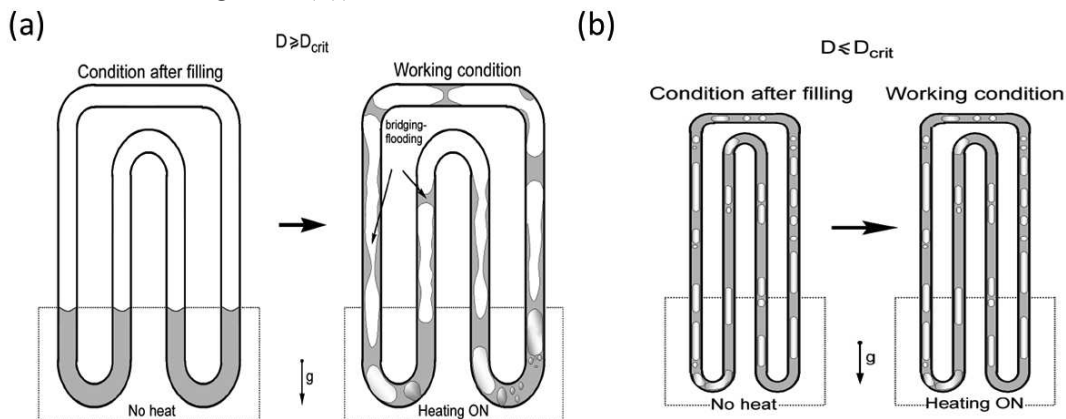
Figure 8 : Type de fonctionnement selon diamètre critique (15)
