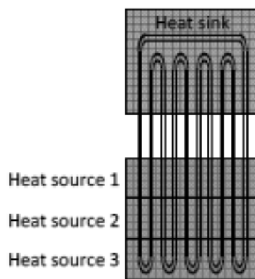
Figure 34 : Chauffage non-uniforme le long d'un caloduc oscillant (53)
