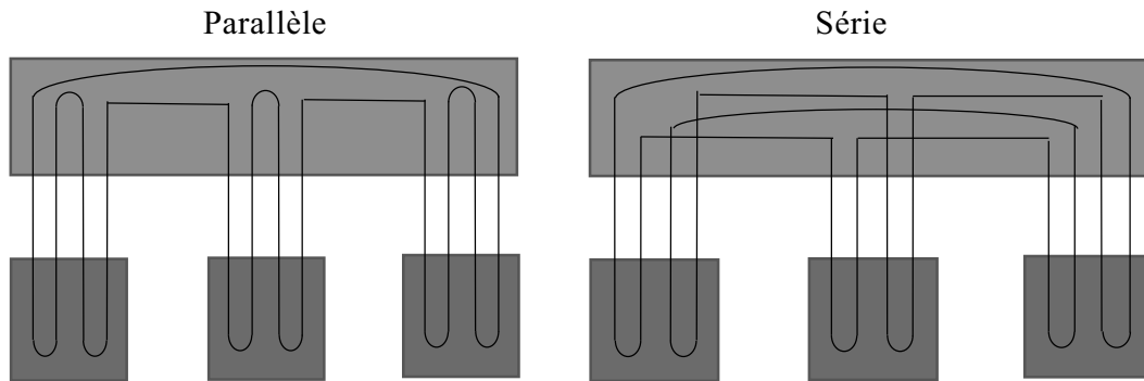
Figure 112 : Schéma de caloduc oscillant avec trois sources en parallèle (gauche) et en série (droite)
