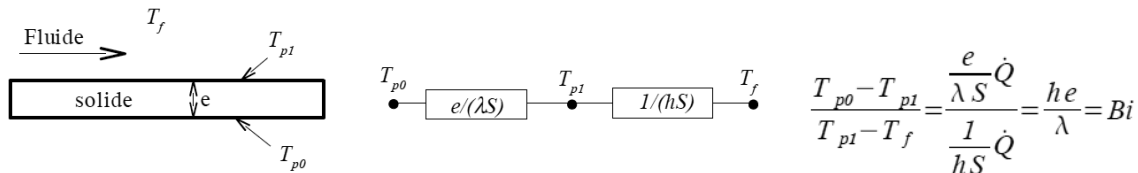
Figure 242 : Schéma d'une paroi solide en contact avec un fluide et du bilan thermique correspondant
