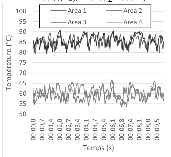
Figure 141 : Evolution temporelle de la température mesurée par visualisation IR (eau, TR = 50 \% , T_{cryo} = 10^{\circ}\text{C} , Q = 4500 \text{ W} )
