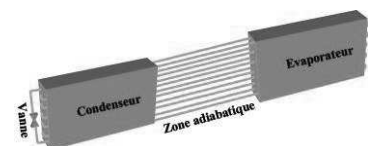
Figure 136 : Vue 3D du caloduc oscillant construit par Bensalem et al. (75)
