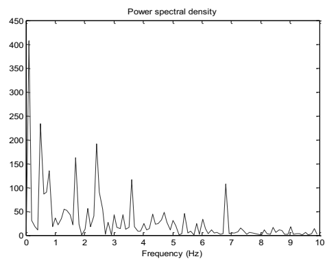
Figure 133 : Densité spectrale de puissance de la température évaporateur (Area 1) mesurée par visualisation IR (eau, TR = 50\% , T_{cryo} = 10^\circ\text{C} , Q = 8400 W)
