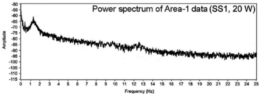
Figure 65 : Densité de puissance spectrale pour l’état SS1 (10)
