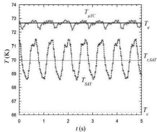
Figure 14 : Mesures de température dans la vapeur et température de saturation correspondant à la pression mesurée (22)
