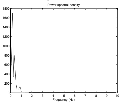
Figure 145 : Densité spectrale de puissance de la température adiabatique (Area 3) mesurée par visualisation IR (eau, TR = 50\% , T_{cryo} = 10^\circ\text{C} , Q = 300\text{ W} )
