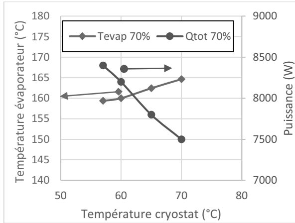
Figure 177 : Température d'évaporateur et puissance à l'assèchement en fonction de la température de source froide (pentane, TR = 70%)
