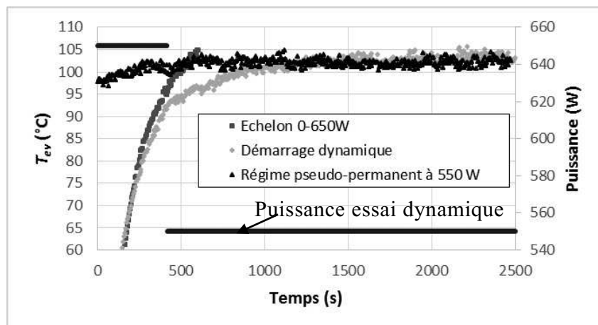
Figure 99 : Réponse dynamique du PHP à différentes sollicitations (pentane, T_{cryo} = 10^{\circ}\text{C} , horizontal)
