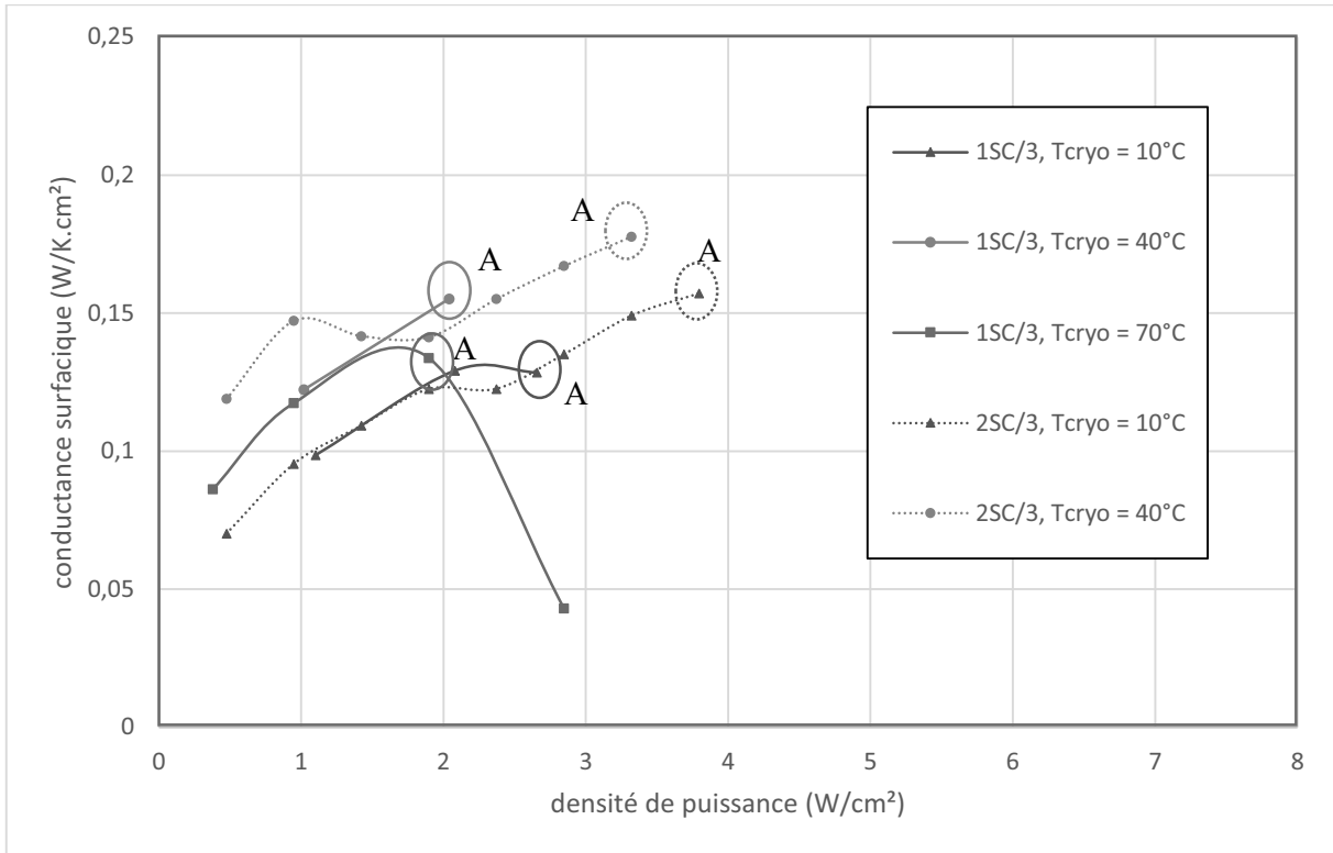
Figure 198 : Zoom sur la conductance surfacique en fonction de la densité de puissance pour différents dispositifs et différentes températures de source froide (pentane, TR = 50\% )
