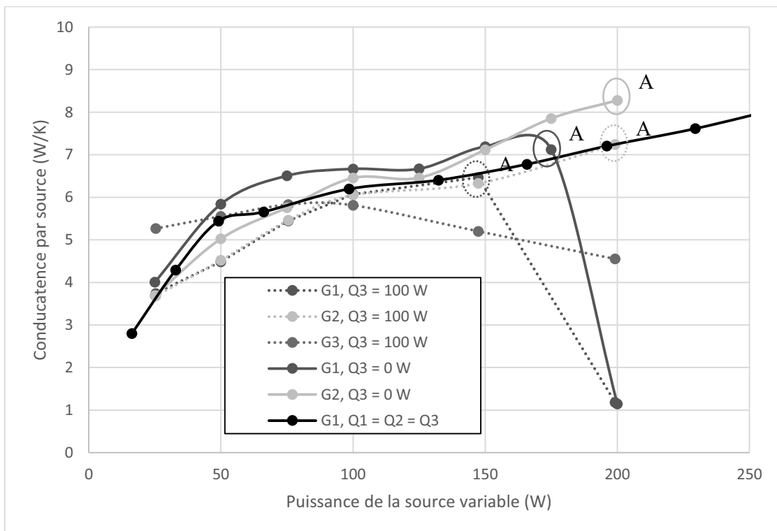
Figure 212 : Conductance par source en fonction de la puissance injectée par source dans les sources à puissance variable (pentane, TR = 50 \% , T_{cryo} = 10^\circ\text{C} )
