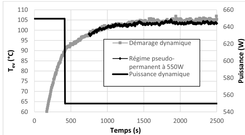
Figure 100 : Réponse transitoire en température pour deux scénarios de puissance appliquée (pentane, T_{cryo} = 10^{\circ}\text{C} , horizontal)
