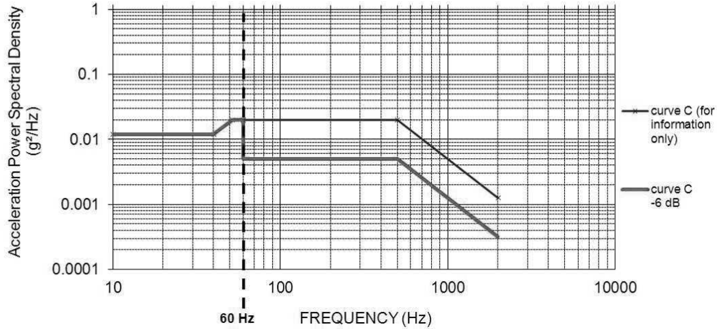
Figure 106 : Courbe qualifiante pour zone de fuselage
