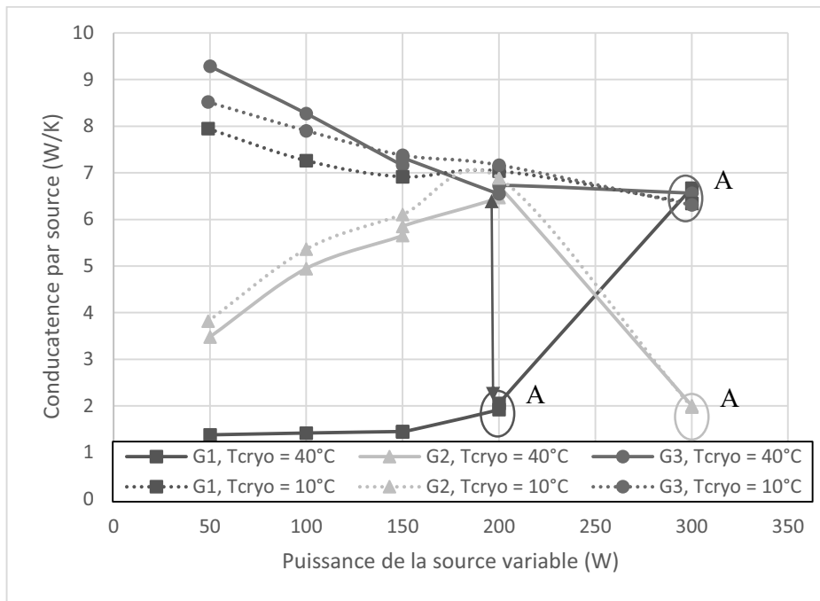
Figure 214 : Conductance par source en fonction de la puissance variable S2 (pentane, TR = 50\% , Q_1 = Q_3 = 200\text{ W} )
