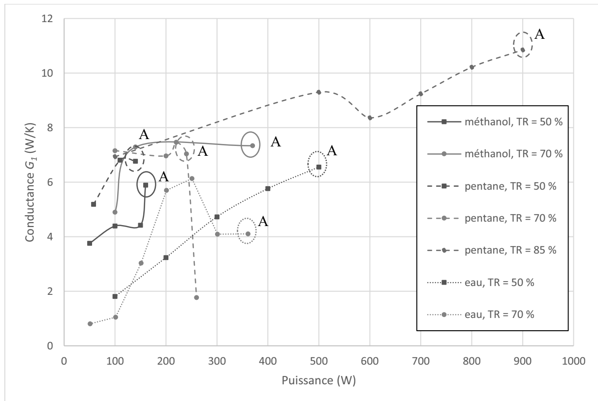
Figure 201 : Conductance G_1 en fonction de la puissance injectée ( Q_2 = Q_3 = 0 \text{ W} , T_{\text{cryo}} = 10^{\circ}\text{C} )
