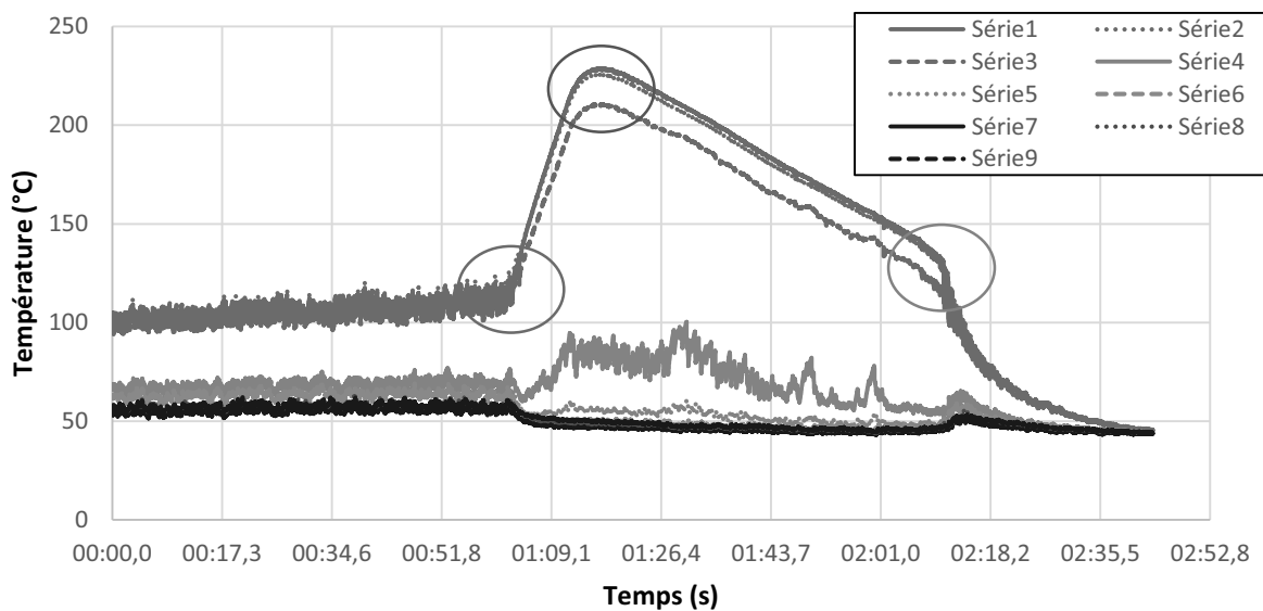
Figure 226 : Relevés de températures mesurées par visualisation IR (méthanol, TR = 70\% , T_{cryo} = 40^\circ\text{C} )
