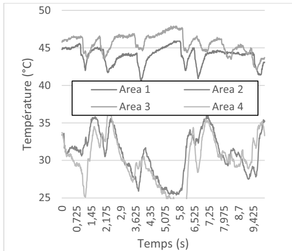
Figure 169 : Evolution temporelle de la température mesurée par visualisation IR dans les zones de mesures (eau, TR = 50\% , T_{cryo} = 10^{\circ}\text{C} , Q = 600\text{ W} )
