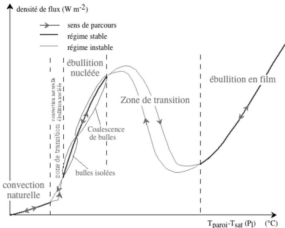
Figure 9 : Courbe d'ébullition au niveau d'une paroi immergée en température imposée (16)
