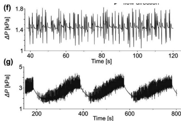
Figure 62 : Oscillations de pressions pour Q = 40 W (f) et Q = 46 W (g) (79)
