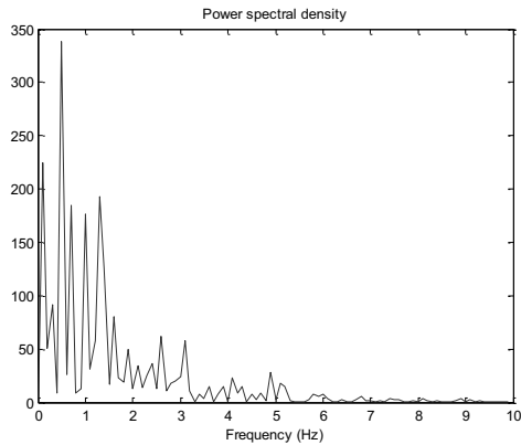
Figure 147 : Densité spectrale de puissance de la température évaporateur (Area 1) mesurée par visualisation IR (eau, TR = 50\% , T_{cryo} = 10^{\circ}C , Q = 4500\ W )
