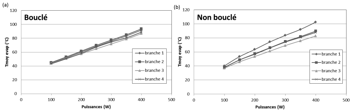
Figure 91 : Comparaisons des températures moyennes dans la zone évaporateur de différentes branches entre les configurations bouclée (a) et non-bouclée (b) (éthanol, TR = 50\% , T_{cryo} = 10^{\circ}C )
