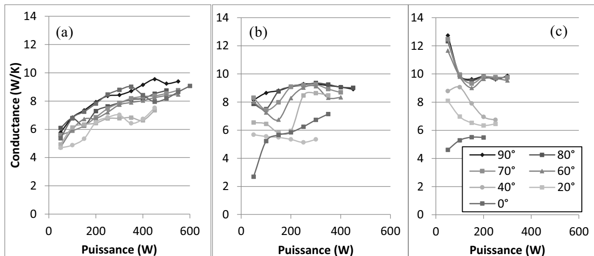
Figure 86 : Conductance globale en fonction de la puissance injectée pour différentes orientations (pentane, TR = 40\% , T_{cryo} = 10^\circ\text{C} (a), 40^\circ\text{C} (b), et 70^\circ\text{C} (c))
