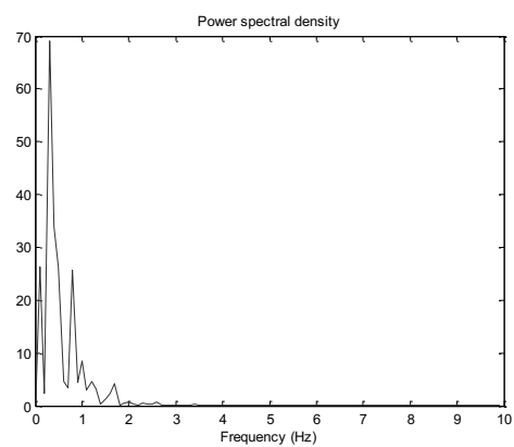
Figure 146 : Densité spectrale de puissance de la température adiabatique (Area 3) mesurée par visualisation IR (eau, TR = 50\% , T_{cryo} = 40^\circ\text{C} , Q = 300\text{ W} )
