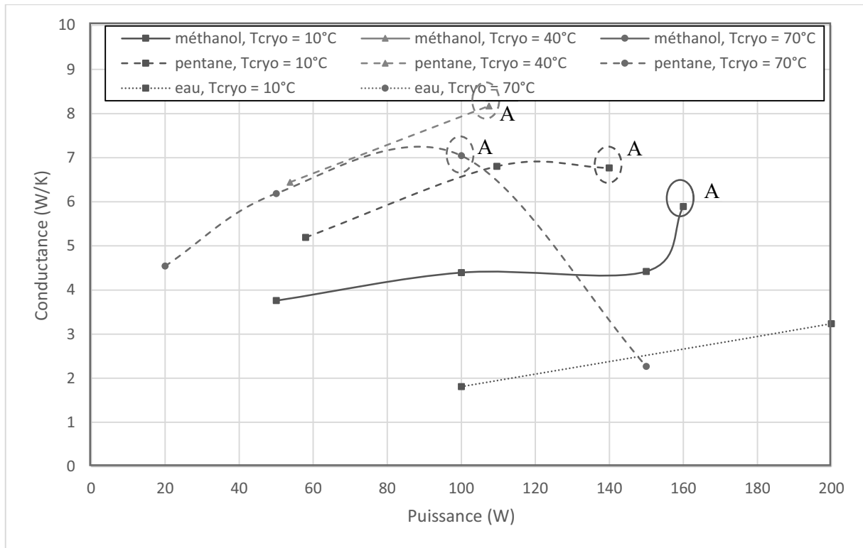
Figure 195 : Zoom sur la conductance de la source active lorsque la puissance est injectée dans une seule source pour différentes températures de source froide (pentane, méthanol, eau, TR = 50\% , Q_1 = Q_2 = 0\text{ W} )
