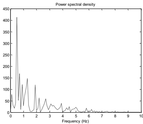
Figure 149 : Densité spectrale de puissance de la température adiabatique (Area 3) mesurée par visualisation IR (eau, TR = 50\% , T_{cryo} = 10^{\circ}C , Q = 4500\ W )
