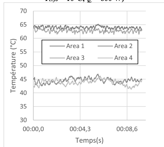
Figure 172 : Evolution temporelle de la température mesurée par visualisation IR dans les zones de mesures (méthanol, TR = 50\% , T_{cryo} = 10^{\circ}\text{C} , Q = 1500\text{ W} )
