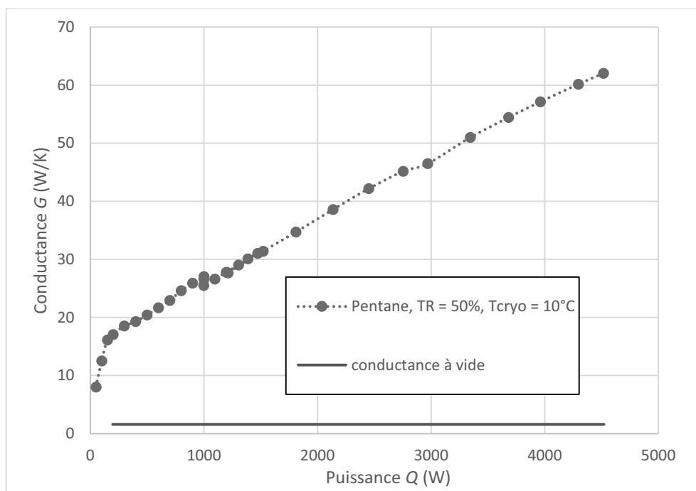
Figure 152 : Conductance globale avec la puissance (pentane, TR = 50 %, T cryo = 10°C)
