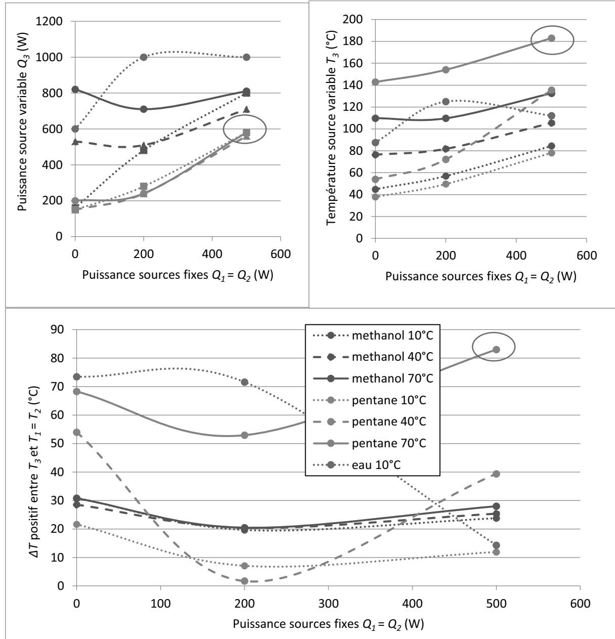
Figure 233 : Limites d'assèchement pour différents fluides et températures de source froide en fonction de la puissance dans les sources fixes ( TR = 50\% Q_1 = Q_2 )
