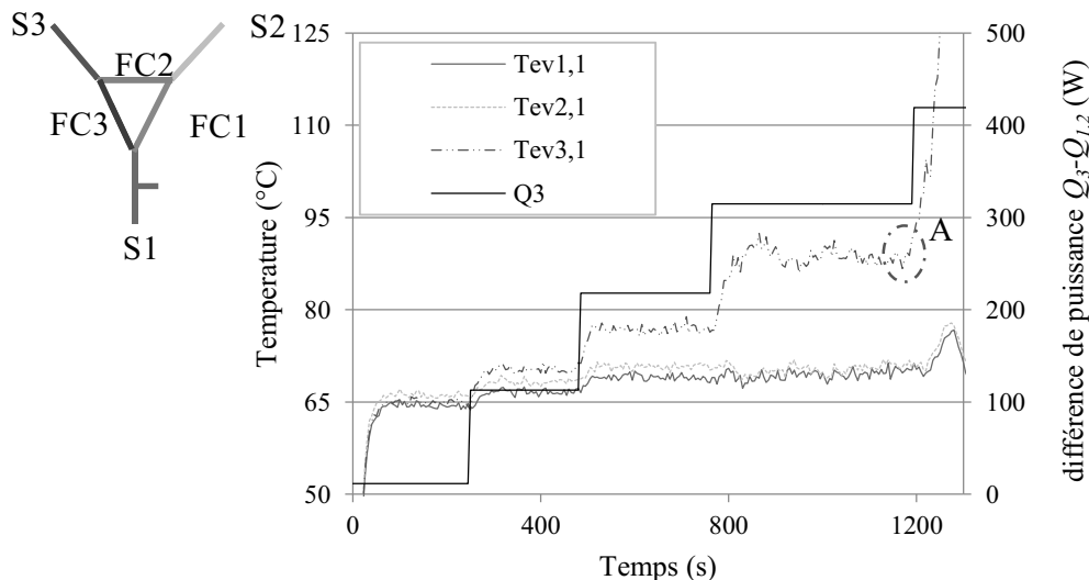
Figure 206 : Evolution temporelle des températures dans les différents évaporateurs lorsque la puissance est augmentée dans S3 (pentane, TR = 70\% , T_{cryo} = 10^{\circ}\text{C} , Q_1 = Q_2 = 500\text{ W} )
