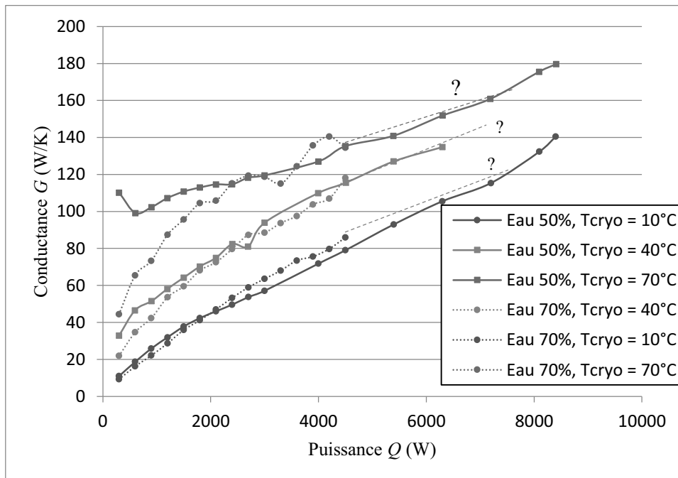
Figure 165 : Conductance en fonction de la puissance pour 3 températures de source froide et deux taux de remplissage (eau)
