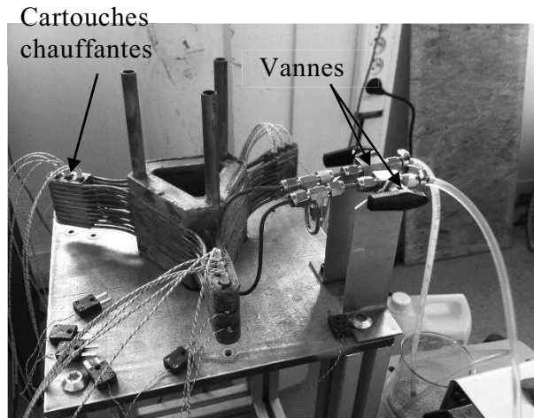
Figure 114 : Photo du dispositif expérimental (durant la phase de nettoyage/oxydation du tube).
