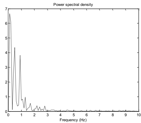
Figure 144 : Densité spectrale de puissance de la température évaporateur (Area 1) mesurée par visualisation IR (eau, TR = 50\% , T_{cryo} = 40^\circ\text{C} , Q = 300\text{ W} )
