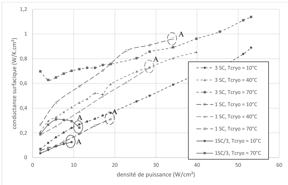
Figure 200 : Conductance surfacique en fonction de la densité de puissance pour différents dispositifs et différentes températures de source froide (eau, TR = 50\% )
