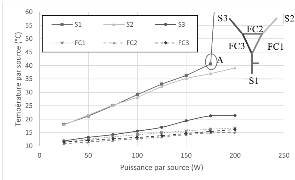
Figure 190 : Température dans chaque source de l'évaporateur et chaque faces du condenseur en fonction de la puissance injectée dans la source 1 et 2 (pentane, TR = 50\% , T_{cryo} = 10^\circ\text{C} , Q_3 = 0\text{ W} )
