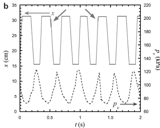
Figure 59 : Mesures du déplacement et de la pression ( P_r = 90 kPa, T_{evap} = 65^{\circ}\text{C} , T_{cond} = 0^{\circ}\text{C} ) (69)
