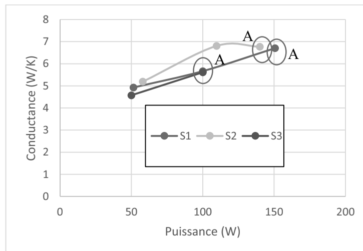
Figure 187 : Conductance de la source active en fonction de la puissance (pentane, TR = 50\% , T_{cryo} = 10^\circ\text{C} )
