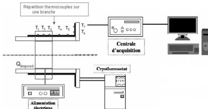
Figure 76 : Schéma global du dispositif expérimental
