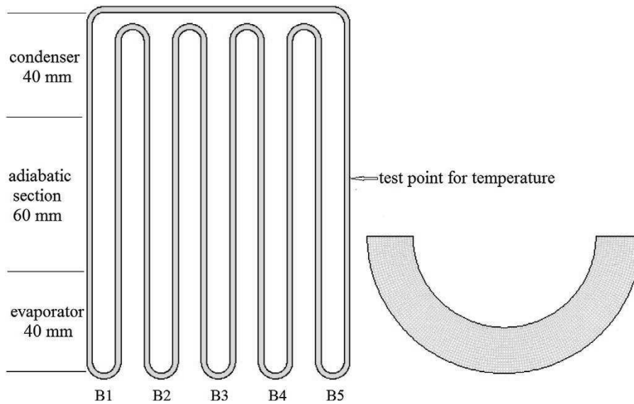
Figure 35 : Chauffage différent d'un tube à l'autre (54)
