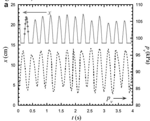
Figure 57 : Mesures du déplacement et de la pression ( P_r = 90 \text{ kPa} , T_{evap} = 45^\circ\text{C} , T_{cond} = 10^\circ\text{C} ) (69)
