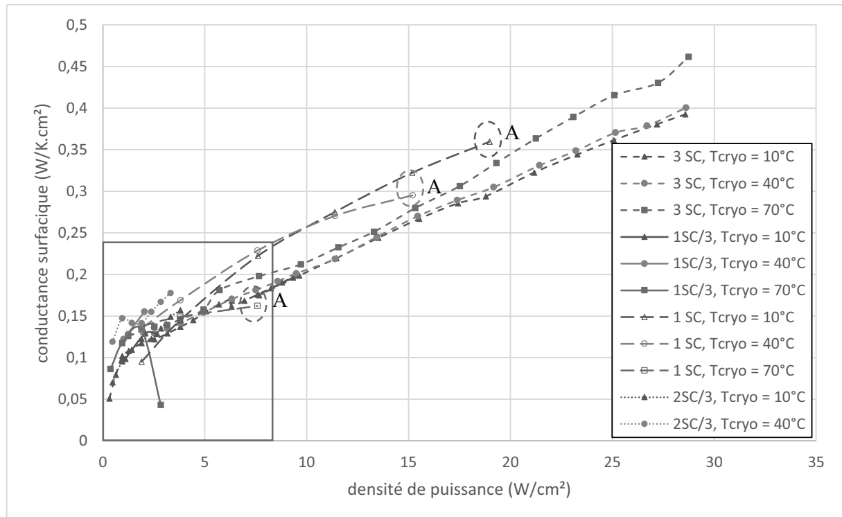
Figure 197 : Conductance surfacique en fonction de la densité de puissance pour différents dispositifs et différentes températures de source froide (pentane, TR = 50\% )
