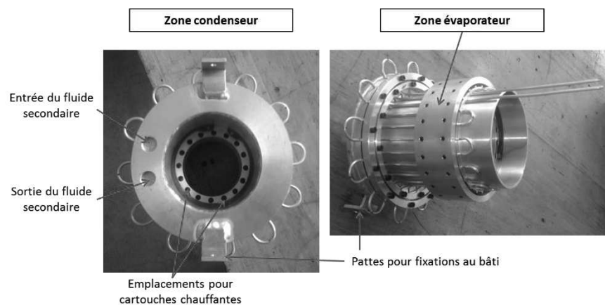
Figure 73 : Vue d'ensemble du système PHP (9)
