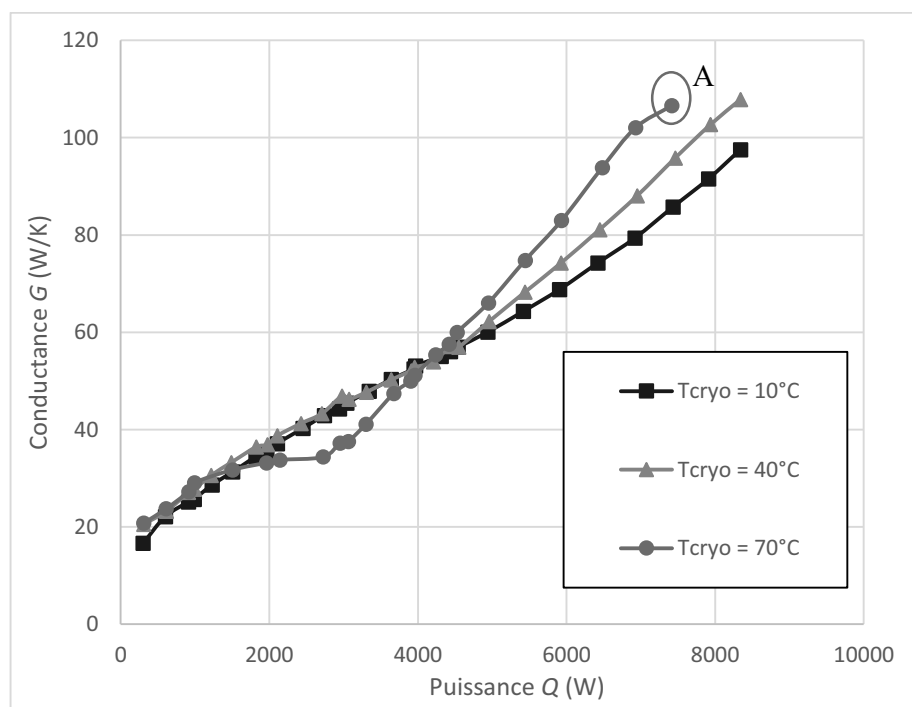
Figure 161 : Conductance en fonction de la puissance injectée pour 3 températures de source froide (pentane, TR = 70\% )
