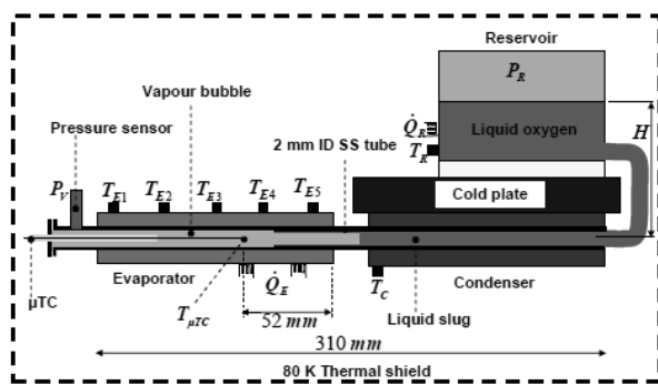
Figure 13 : Schéma du dispositif expérimental monobranche horizontal cryogénique (22)
