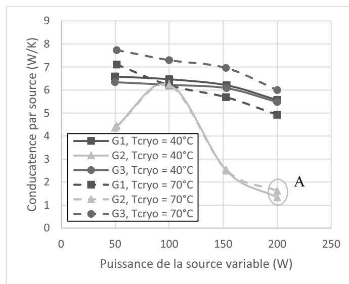
Figure 213 : Conductance par source en fonction de la puissance variable S2 (pentane, TR = 50\% , Q_1 = Q_3 = 100 W)
