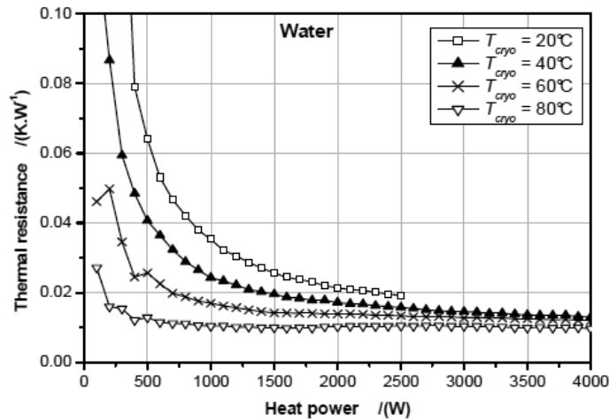
Figure 37 : Evolution de la résistance thermique globale avec la variation de la température de source froide (fluide : eau) (56)
