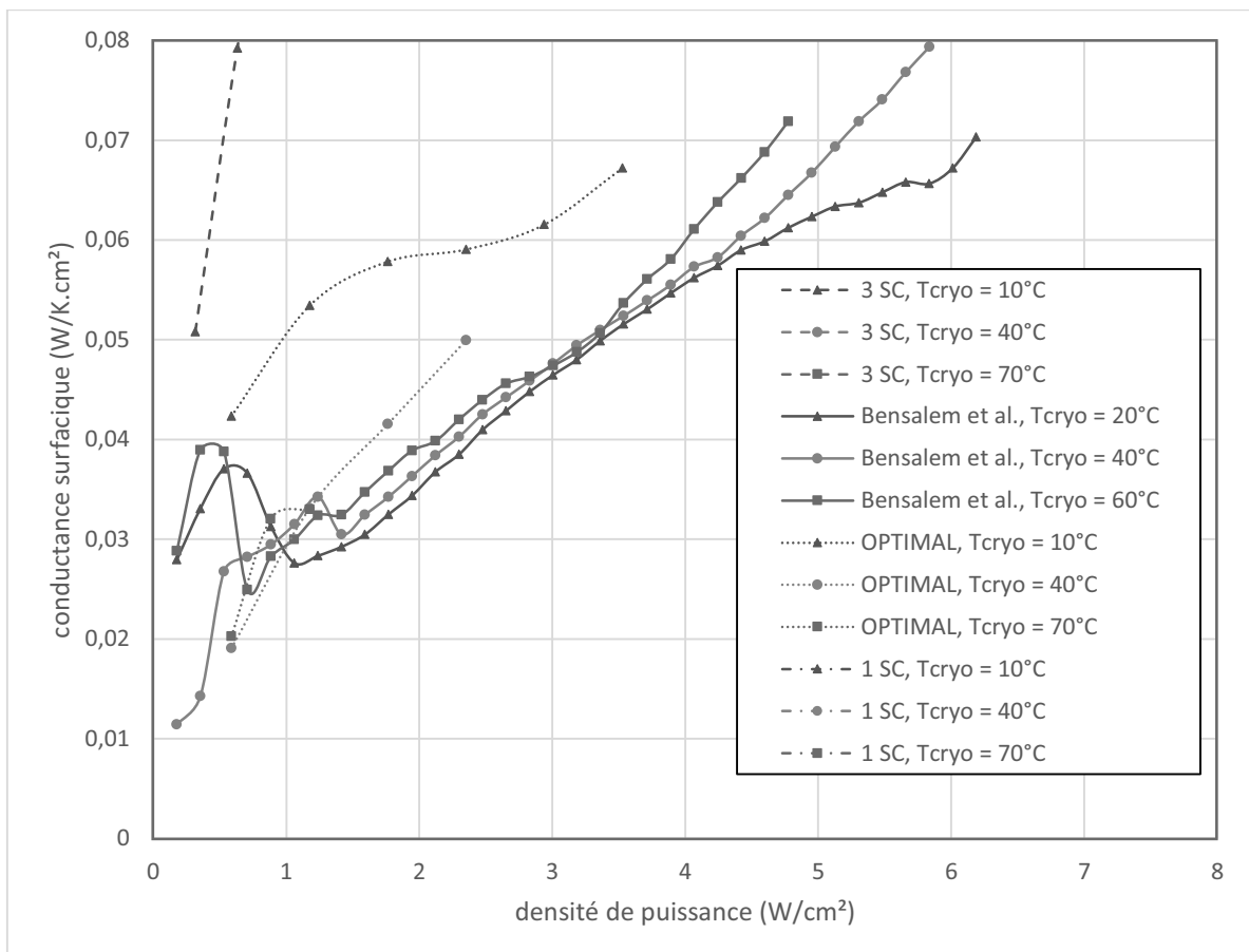
Figure 155 : Zoom sur la conductance surfacique en fonction de la densité de puissance pour différents dispositifs (pentane, TR = 50 %)
