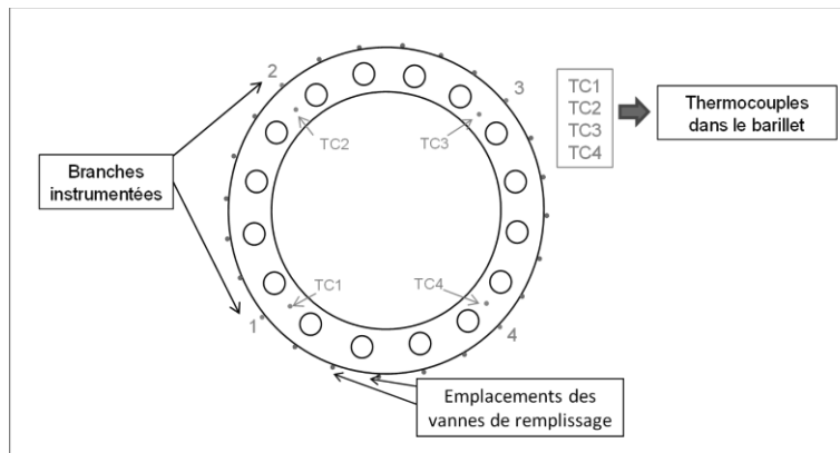
Figure 75 : Schéma des branches instrumentées sur une vue en coupe
