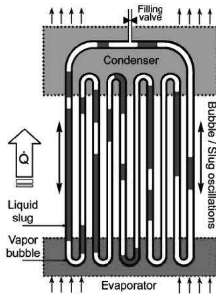
Figure 1 : Schéma de principe du caloduc oscillant (10)
