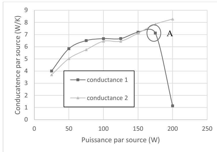
Figure 189 : Conductance des sources actives en fonction de la puissance injectée par source (pentane, TR = 50\% , T_{cryo} = 10^\circ\text{C} , Q_3 = 0\text{ W} )
