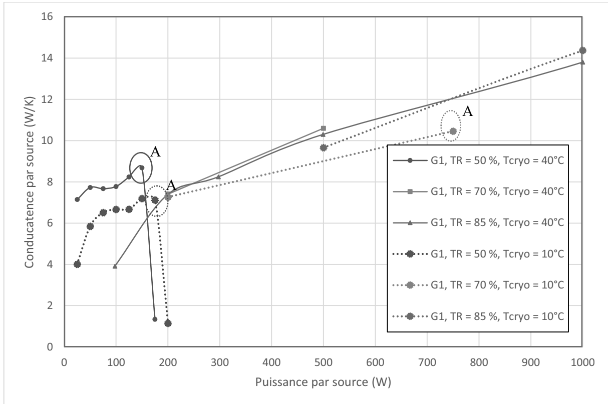
Figure 203 : Zoom sur la conductance G_1 en fonction de la puissance injectée ( Q_3 = 0 W, pentane)
