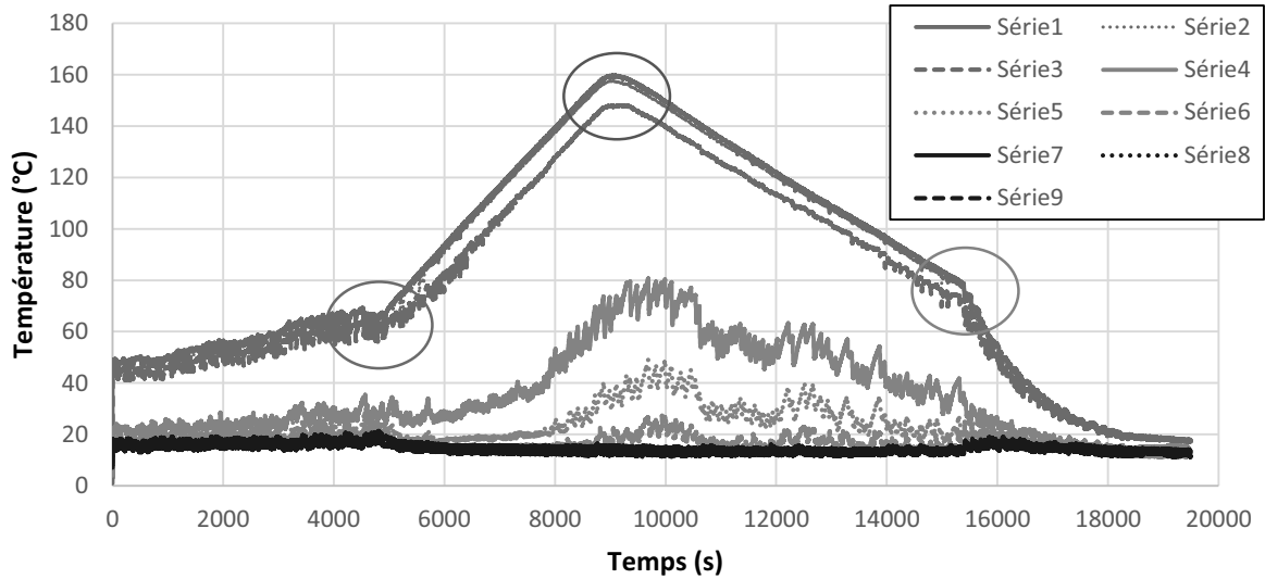
Figure 225 : Relevés de températures mesurées par visualisation IR (méthanol, TR = 70\% , T_{cryo} = 10^\circ\text{C} )
