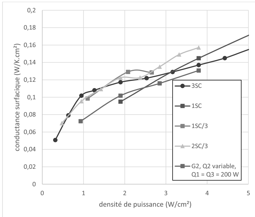
Figure 217 : Conductance dans la source S2 pour différentes configurations de la répartition de la puissance (Pentane, TR = 50\% , T_{cryo} = 10^{\circ}C )
