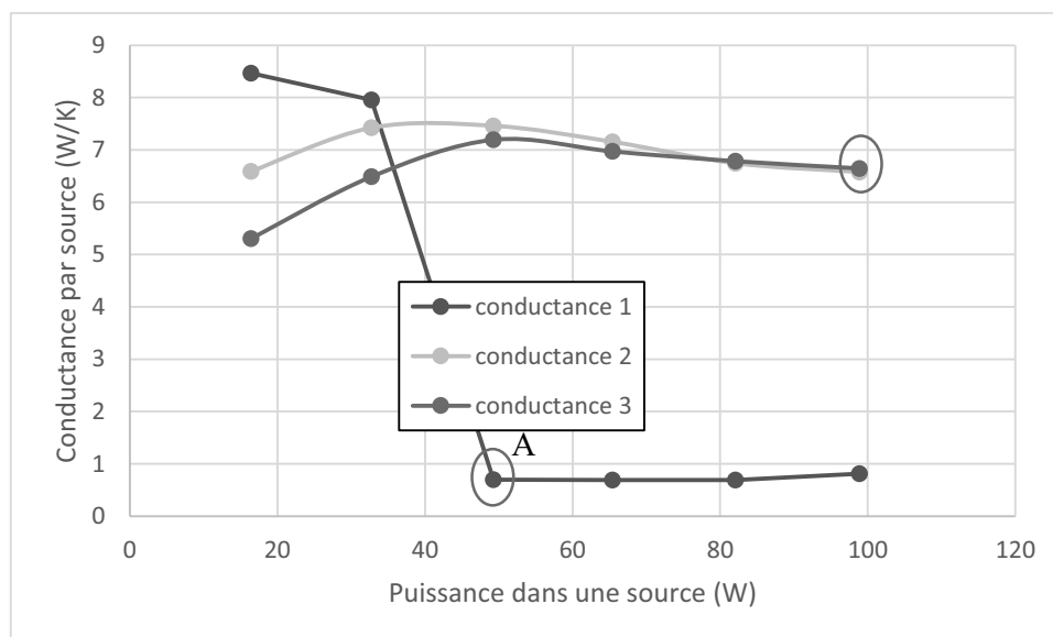
Figure 156 : Conductance par source en fonction de la puissance injectée par source (pentane, TR = 20\% , T_{cryo} = 10^{\circ}C )
