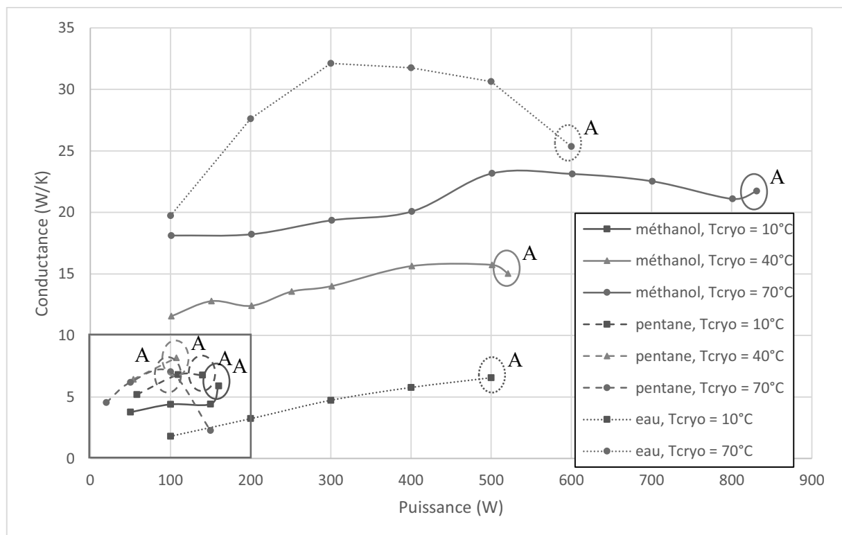
Figure 194 : Conductance de la source active lorsque la puissance est injectée dans une seule source pour différentes températures de source froide (pentane, méthanol, eau, TR = 50\% , Q_1 = Q_2 = 0 W)
