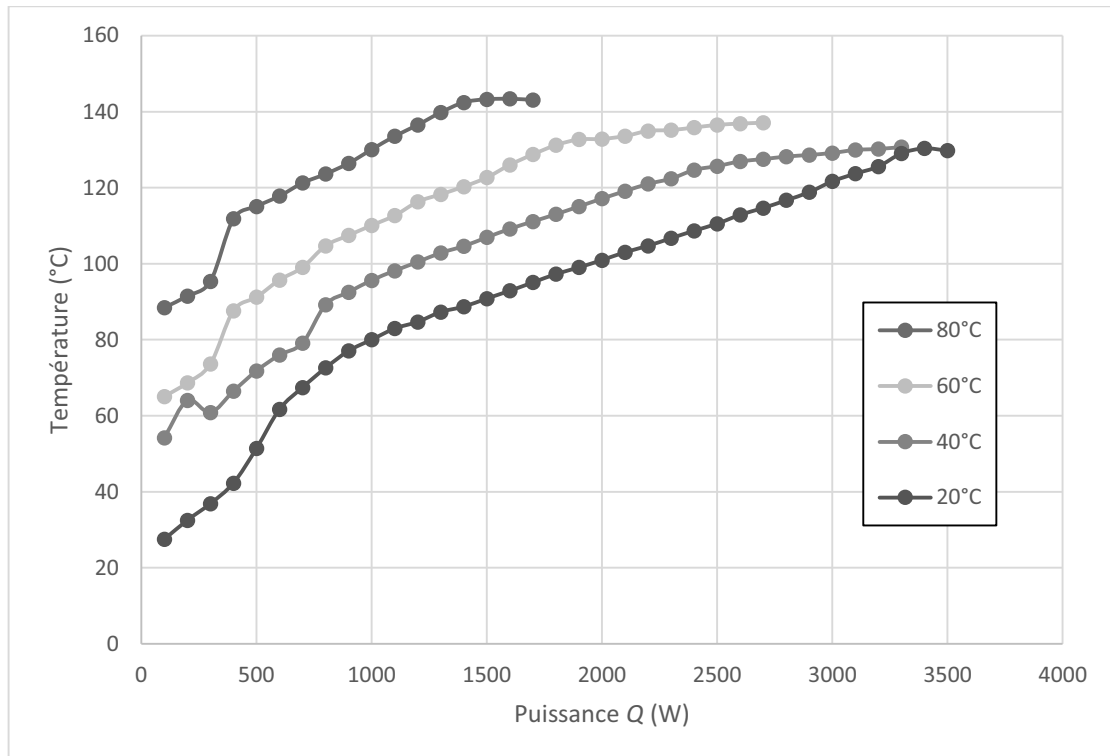
Figure 163 : Température d'évaporateur en fonction de la puissance injectée pour 4 températures de source froide (pentane, TR = 50\% , dispositif Bensalem et al. (75))
