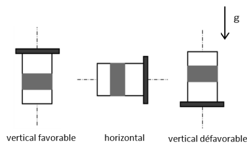
Figure 74 : Schéma des principales positions d'orientation
