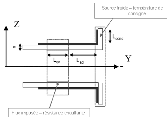
Figure 107 : Schéma des axes de vibrations sur le dispositif
