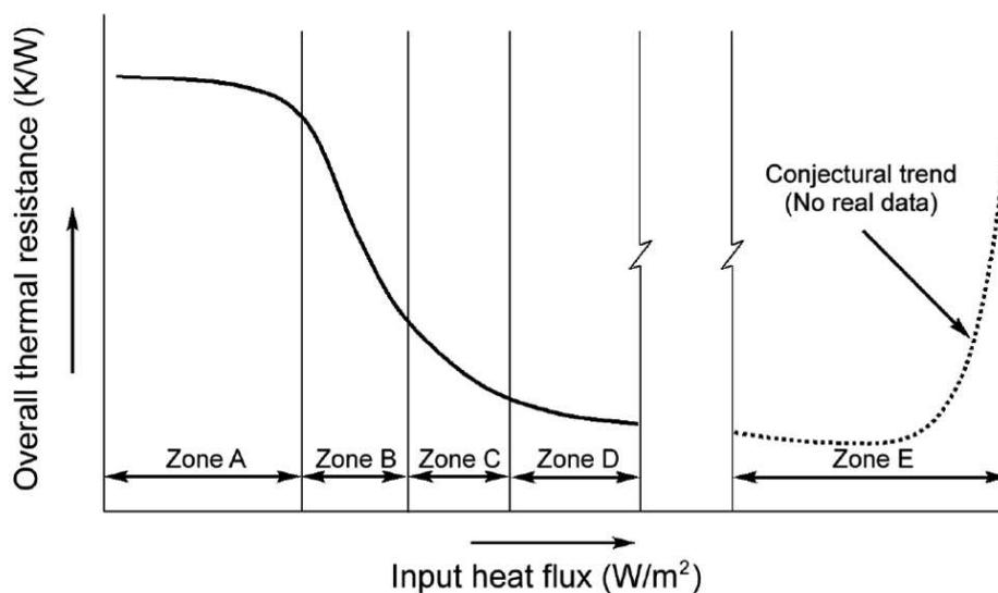
Figure 11 : Performance et localisation des régimes fluidiques en fonction du flux imposé (18)
