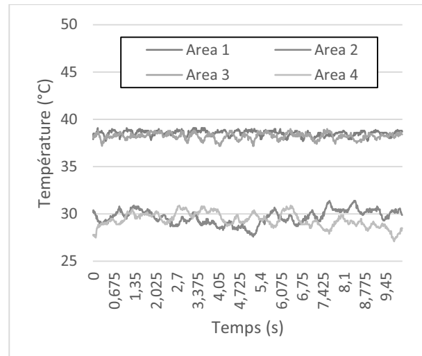
Figure 170 : Evolution temporelle de la température mesurée par visualisation IR dans les zones de mesures (méthanol, TR = 50\% , T_{cryo} = 10^{\circ}\text{C} , Q = 600\text{ W} )
