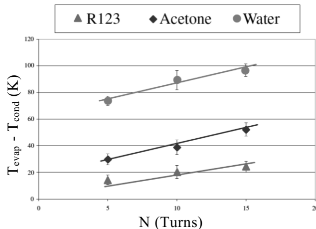
Figure 51 : Influence du nombre de boucles sur la différence de température évaporateur-condenseur nécessaire au démarrage (67)
