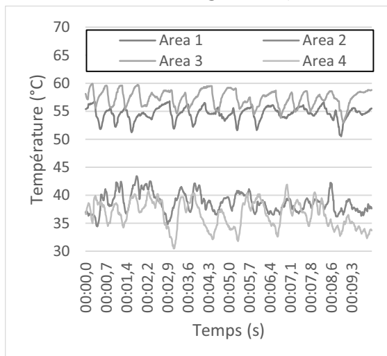
Figure 171 : Evolution temporelle de la température mesurée par visualisation IR dans les zones de mesures (eau, TR = 50\% , T_{cryo} = 10^{\circ}\text{C} , Q = 1500\text{ W} )
