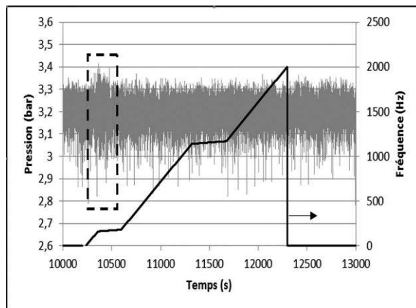
Figure 109 : Influence de la fréquence sur le signal de pression ( 1g , T_{cryo} = 40^{\circ}C , Q = 300 W )
