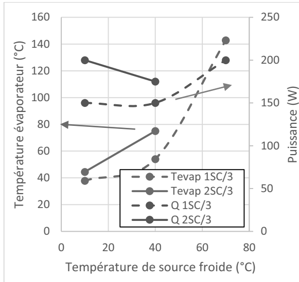
Figure 229 : Température et puissance avant assèchement en fonction de la température de source froide pour deux configurations (pentane, TR = 50\% )
