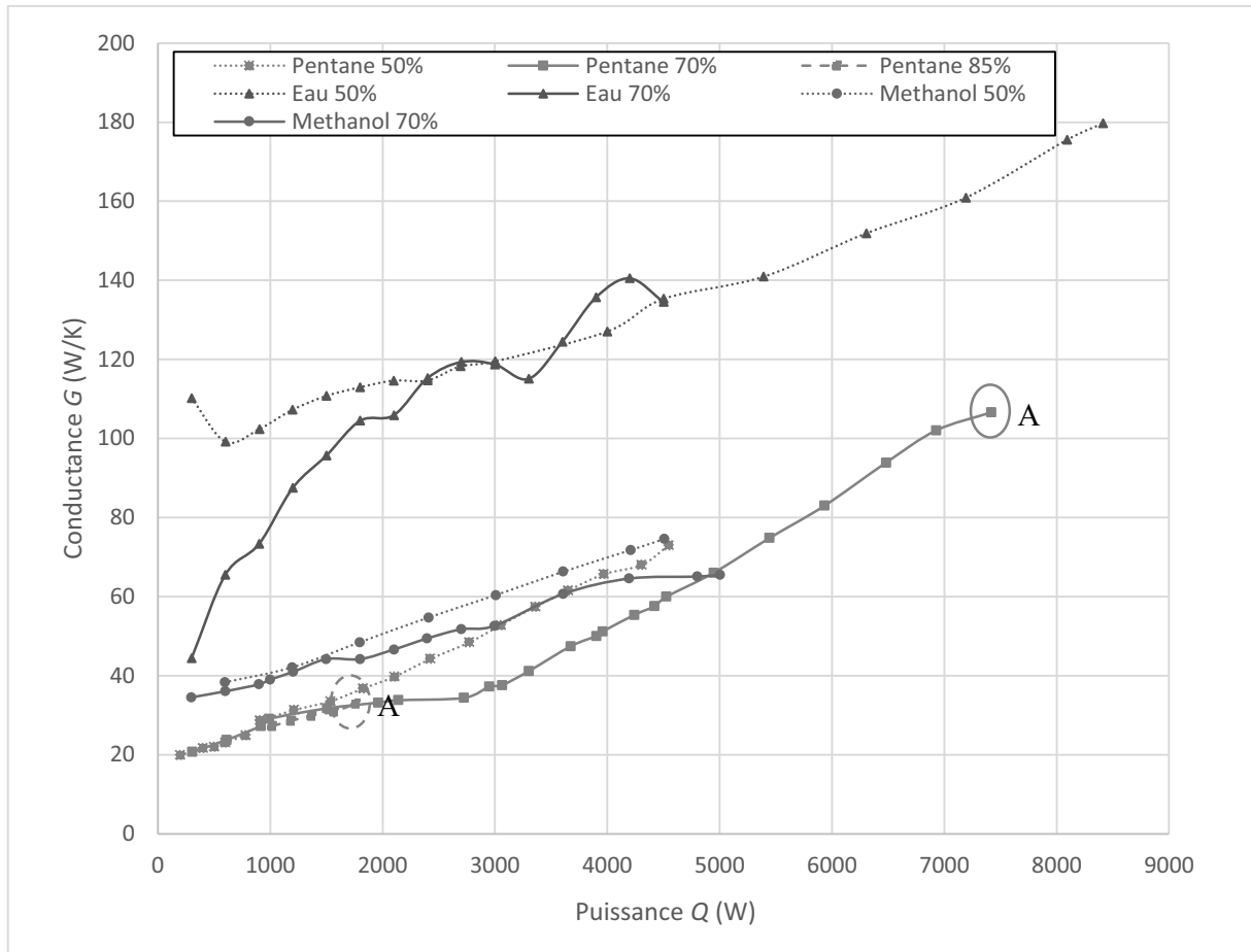
Figure 168 : Conductance en fonction de la puissance pour les trois fluides ( T_{cryo} = 70^{\circ}\text{C} )
