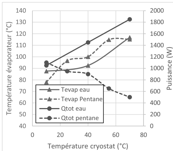
Figure 185 : Température et puissance avant assèchement en fonction de la température de source froide ( TR = 50\% )
