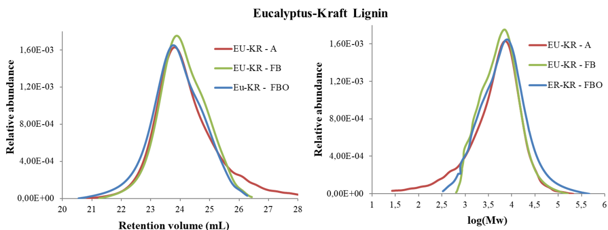
Figure 33. Profils d'élution SEC des différentes lignines dérivées – dans le système THF et calibration universelle : Abondance relative en fonction du volume de rétention ( gauche ) et abondance relative en fonction de log (Mw) ( droite ) (A - acétylée, FB - fluorobenzylée et FBO - fluorobenzoylée)
