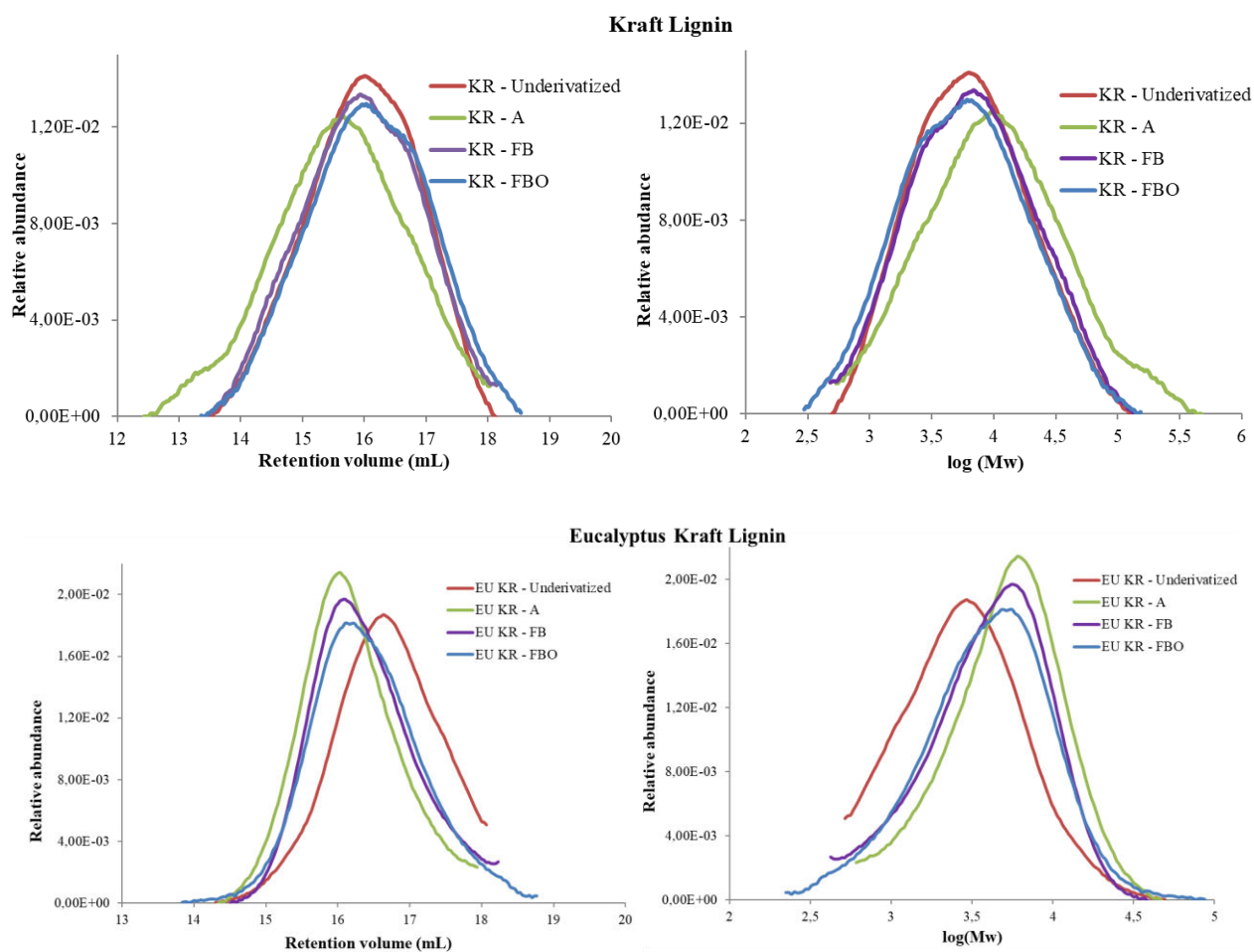
Figure 32. Profils d'élution SEC des lignines non dérivées et dérivées (acétylation, fluorobenzoylation et fluorobenzoylation), abondance relative en fonction du volume de rétention (gauche) et abondance relative en fonction de log (Mw) (droite)
