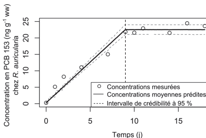
Figure 42. Cinétiques d’accumulation et d’élimination du PCB 153 chez le radix. Le trait vertical pointillé délimite la phase d’exposition de la phase de dépuration. Le trait plein représente les concentrations moyennes prédites dans le radix et les traits pointillés l’intervalle de crédibilité à 95 % des prédictions.
