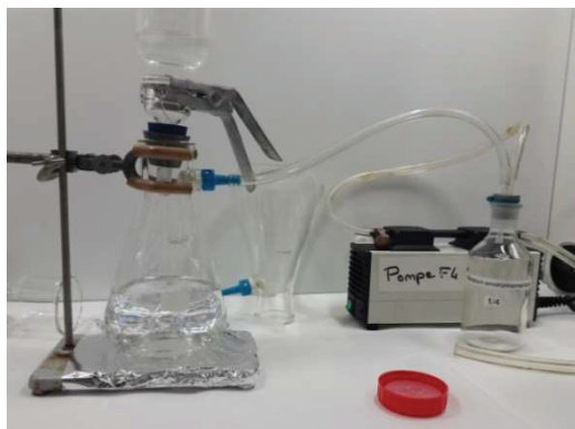
Figure 39. Système de filtration des échantillons d'eau.
