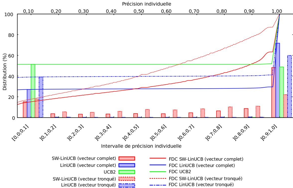
FIGURE 5.3 – Distribution de la précision individuelle pour chaque algorithme sur le jeu de données Coverttype ( vc et vt )
