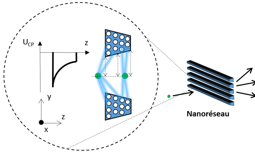
FIGURE III.12 – Schéma illustrant la méthode de calcul du déphasage atomique par « paire atomique ». Le graphe donne l'allure du potentiel d'interaction en fonction de z .
