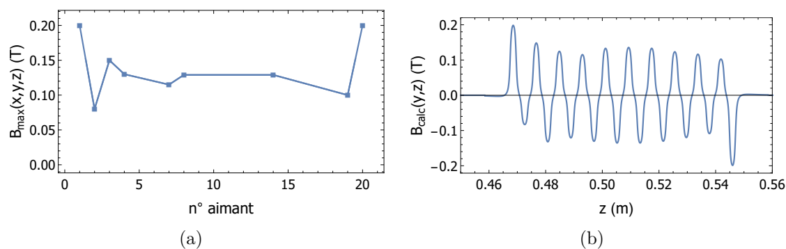
FIGURE II.16 – (a) Points de mesure à B_{max} ( i.e. courant de 10 A) relevés par Bouhnik®. La constante de temps vaut dans ce cas 50 \mu\text{s} . Les variations temporelles du champ ont été mesurées à l'aide d'une sonde à effet Hall. (b) Allure théorique du champ magnétique statique dont le calcul est présenté en annexe E.
