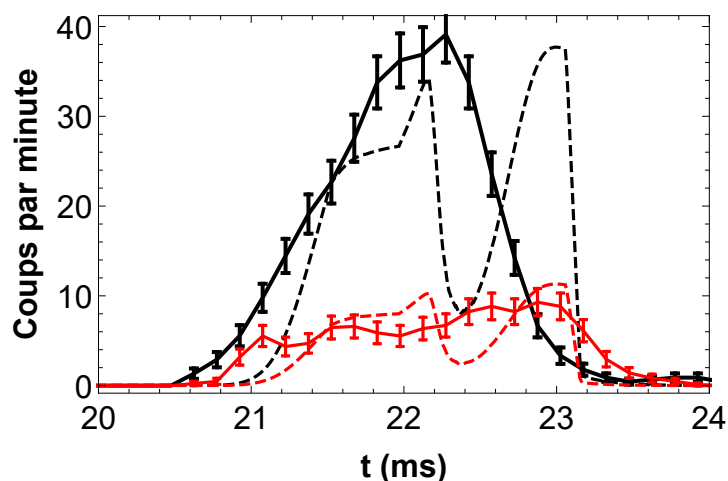
FIGURE II.26 – Spectres de temps de vol théoriques et expérimentaux d'atomes à 50 \text{ m.s}^{-1} dans le sous-niveau magnétique |m_J = -2\rangle pour le calcul à l'ordre 0. En trait noir plein, le spectre de référence expérimental en l'absence de potentiel; en trait rouge plein, le spectre modifié expérimental pour un temps de déclenchement t_{ON} = 10,57 \text{ ms} ; en trait noir hachuré, le spectre modifié théorique sans atténuation du flux; en trait rouge hachuré, le spectre modifié calculé à l'aide de II.2.23 ou II.2.38 en tenant compte de la transmission donnée par le graphe de la figure II.20
