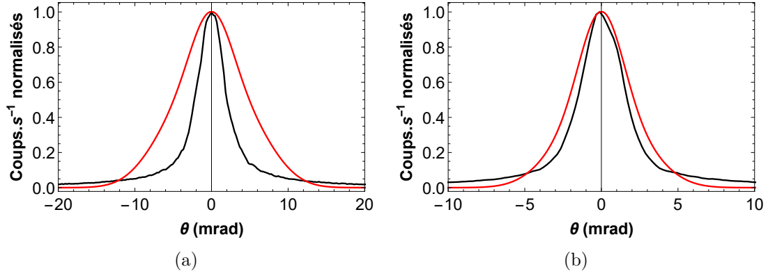
FIGURE III.15 – Courbes théoriques qui donnent des profils de diffraction calculés à partir de la valeur de la fente effective et ce, en fonction de la vitesse atomique longitudinale, (a) à 100 \text{ m.s}^{-1} , (b) à 150 \text{ m.s}^{-1} .
