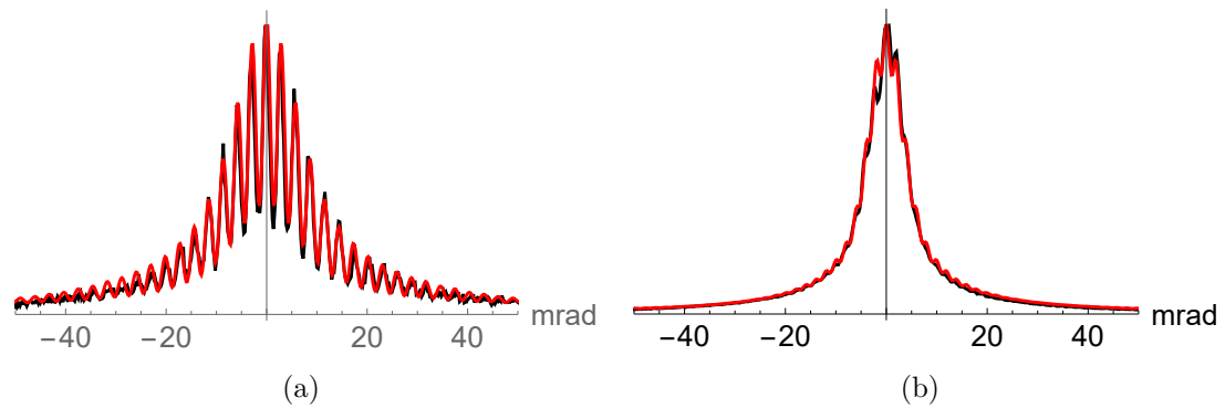
FIGURE III.26 – Profils de diffraction atomique par un réseau de tailles e = 65 nm et L = 130 nm pour des atomes à vitesse de (a) 34,5 \text{ m.s}^{-1} , R_C = 136 nm et (b) 50 \text{ m.s}^{-1} , R_C = 80 nm. En noir, l'expérience. En rouge, le calcul de type « paire atomique » d'après l'équation III.2.19 pour un paquet d'ondes.
