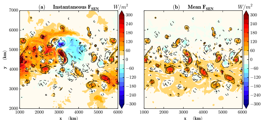
FIGURE 3.1 – Flux turbulent sensibles. Flux de chaleur sensible de l’océan vers l’atmosphère (en couleurs et en W/m^2 ) à un instant donné (a) et en moyenne temporelle (b). Les contours correspondent aux anomalies de SST (-4 K, -2 K, 2 K et 4 K). Obtenu à partir de la simulation EDDY .
