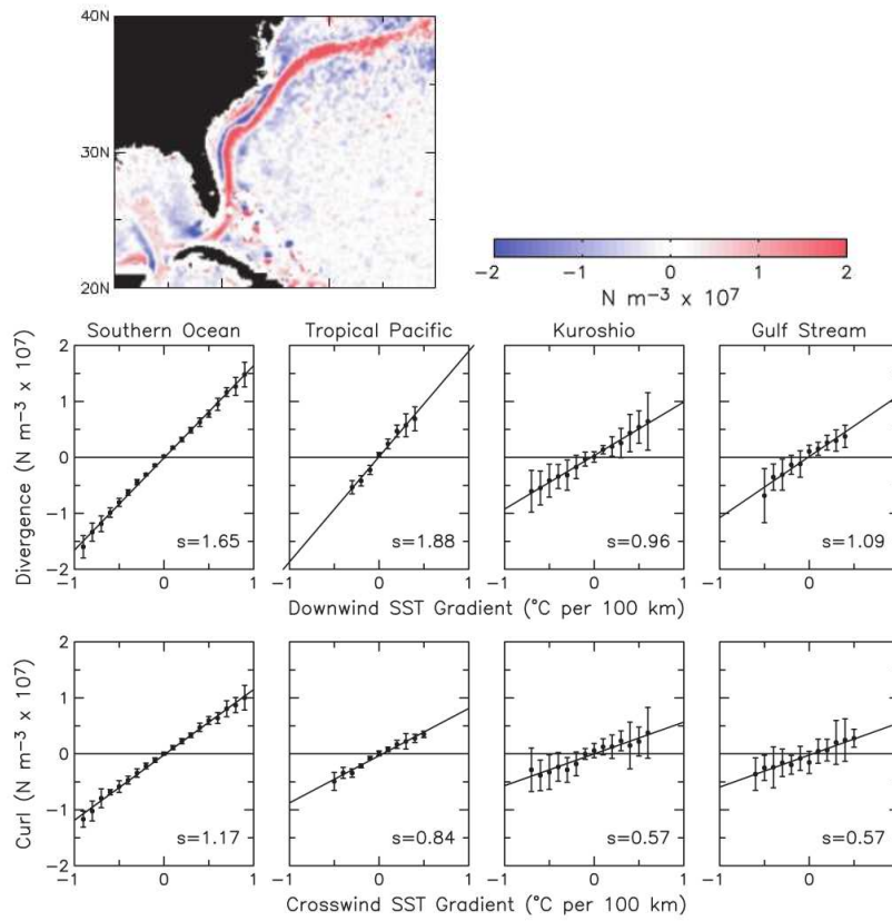
FIGURE 1.7 – Observation du rotationnel de tension de vent au niveau du Gulf Stream. (a) Rotationnel de la tension de vent (en 10^{-7} N/m ^{-3} ), obtenu à partir des mesures par diffusionmètre QuickSCAT sur une période de 4 ans (1999-2003). La tension de vent correspondant à la circulation atmosphérique moyenne de grande échelle a été filtrée. (b) Valeurs moyennes, pour différentes valeurs des gradients de SST dans la directions parallèle au vent, de la divergence de la tension de vent, à partir des données QuickSCAT moyennées sur 6 semaines. Les coefficients de régression linéaire utilisés pour estimer \alpha_D sont indiqués pour chacune des quatre régions d'étude. (c) Valeurs moyennes, pour différentes valeurs des gradients de SST dans la direction perpendiculaire au vent, du rotationnel de la tension de vent, avec les estimations de \alpha_C . Tiré de Chelton et al. (2004) .
