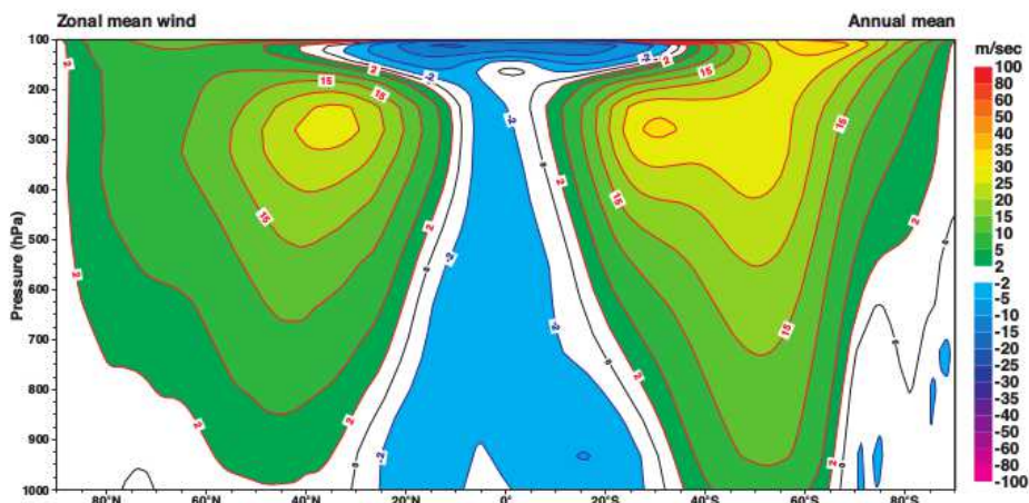
FIGURE 2 – Courant jet. Moyenne annuelle et zonale du vent zonal (en \text{m/s} ), à partir de la réanalyse ERA-40 (ECMWF).
