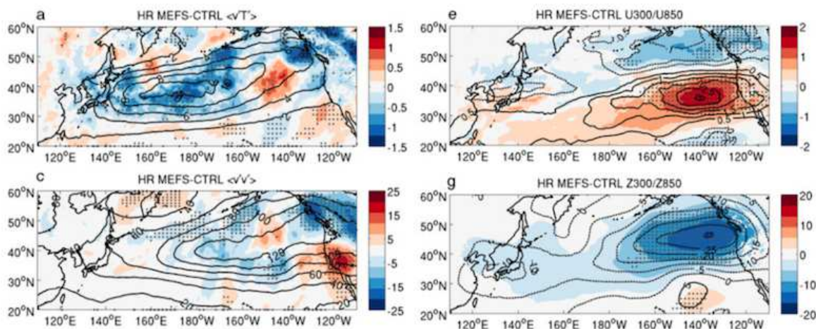
FIGURE 1.12 – Réponse à distance à la suppression de la mésoéchelle océanique sur différentes grandeurs atmosphériques. Tiré de Ma et al. (2017). Les différentes quantités sont obtenues à partir de deux jeux de simulations à haute résolution (27 km, MEFS et CTRL), avec leurs climatologies sur dix hivers dans le Pacifique Nord. Les simulations CTRL sont forcées par les SST de l'hiver 2007-2008 (observations dans les micro-ondes et interpolation optimale). Pour les simulations MEFS, un filtre spatial ( 15^\circ \times 5^\circ ) est appliqué à la SST de manière à éliminer la mésoéchelle. L'anisotropie du filtre permet de limiter la réduction du gradient méridien de SST. La figure présente les différences MEFS-CTRL pour (a) le flux de chaleur méridien à 850 hPa ( \text{m/s K} ), (c) la variance du vent méridien à 300 hPa ( \text{m}^2/\text{s}^2 ), (e) le vent zonal à 850 hPa ( \text{m/s} ), (g) le géopotentiel à 850 hPa ( \text{m} ). Pour (a) et (c), les contours représentent les mêmes quantités pour les moyennes de CTRL. Pour (e) et (g), ils représentent les différences MEFS-CTRL pour les mêmes quantités à 300 hPa. Les zones hachurées délimitent les régions où les différences sont significatives à plus de 95%, sur la base d'un test de somme des rangs de Wilcoxon et en supposant que les sorties journalières constituent des réalisations indépendantes.
