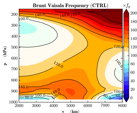
FIGURE 2.13 – Fréquence de Brunt-Väisälä divisée par f_0=9.4 \times 10^{-5} \text{ s}^{-1} , pour la simulation CTRL , calculée à partir du champ de température en moyenne zonale et temporelle (sans unité).
