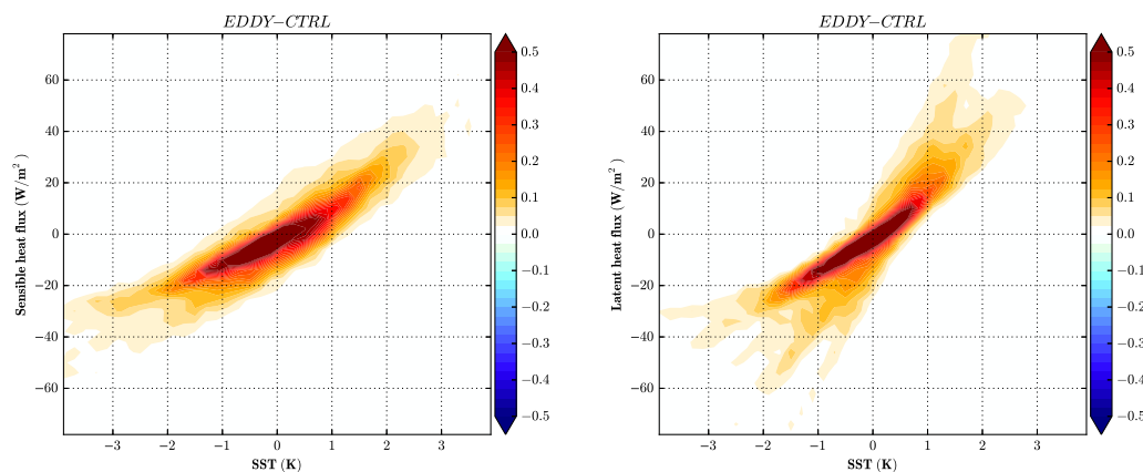
FIGURE 3.2 – PDF des flux de surface. Densité de probabilité jointe des flux de chaleur (en \text{W}/\text{m}^2 ) et des SST (en K). Gauche : flux sensible. Droite : flux latent. La densité a été construite à partir des différences EDDY-CTRL des moyennes temporelles des flux turbulents de surface et des SST, pour chacun des points de l'espace situés dans la bande de latitudes entre y=3600 km et y=5400 km. Les figures construites à partir des anomalies de EDDY par rapport à la moyenne zonale présentent la même forme caractéristique incurvée (non-montrées).
