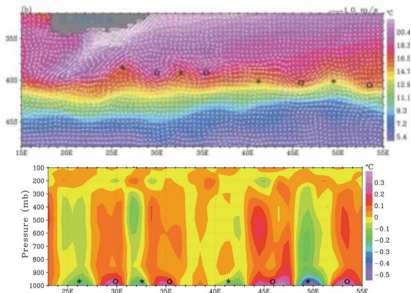
FIGURE 3.4 – Réponse observée en température aux méandres de l'ARC. Tiré de Liu et al. (2007). Haut : SST (en K, observations AMSR-E) et courants de surface (mesures Lagrangiennes) moyens sur 3 années au niveau du courant de retour des Aiguilles. Bas : Profil longitude-pression de température atmosphérique (en K) à 40° S et aux petites échelles. Il est obtenu à partir des températures obtenus à partir des mesures de radiance dans l'infrarouge de l'instrument AIRS, sur la même période. Les ronds et les croix correspondent aux positions des anomalies de SST chaudes et froides respectivement, dont les amplitudes varient entre 0.5 K et 1 K. Liu et al. (2007) estiment que les différences supérieures à 0.07 K sont significatives devant les erreurs sur les mesures instantanées de l'instrument AIRS si ces mesures ne sont pas biaisées.
