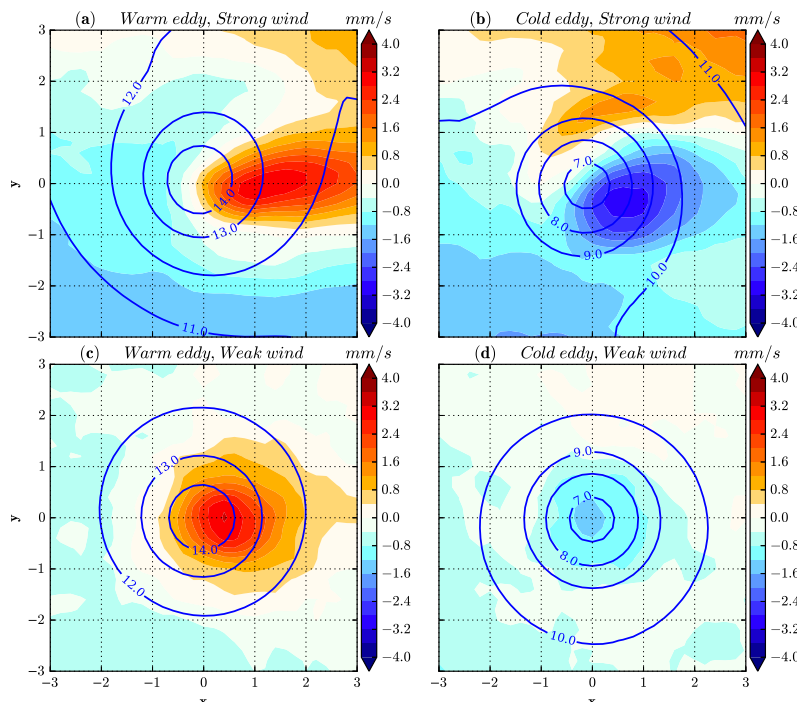
FIGURE 2.15 – Composite de vitesse verticale sur les tourbillons. Composites des vitesses verticales dans la couche limite, moyennées verticalement entre la surface et 500 m (en mm/s). Ils sont obtenus à partir de la simulation EDDY 1K . Les différents panneaux correspondent à des tourbillons chauds (a, c) et froids (b, d), et des vents forts (a-b, supérieurs à 10 m/s) ou faibles (c-d, inférieurs à 5 m/s).
