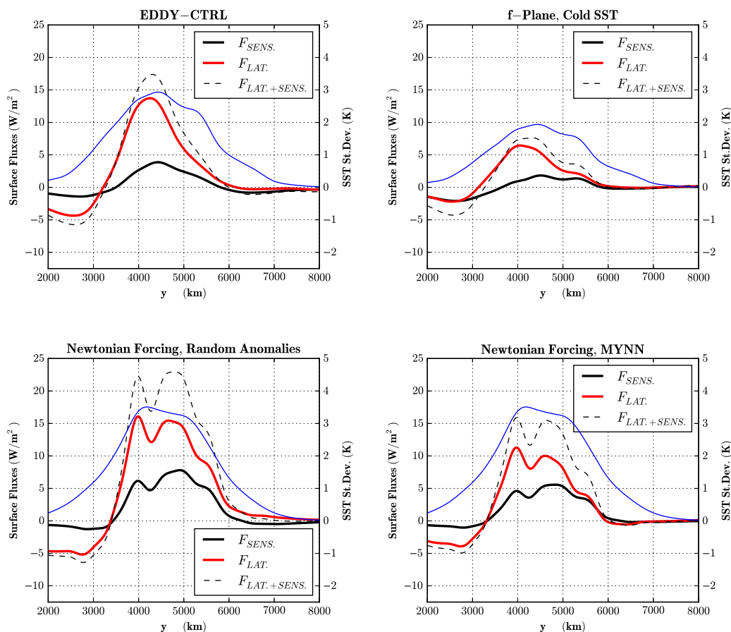
FIGURE 3.3 – Effet net sur les flux de surface. Différences EDDY-CTRL des flux turbulents de l’océan vers l’atmosphère, pour la partie latente F_{LAT} (rouge) et la partie sensible F_{SEN} (noir), en W/m^2 . La courbe bleue correspond à l’écart type des anomalies de SST en fonction de la latitude, pour le cas EDDY (en K). Un filtre Gaussien G(y) = \exp(-y^2/r^2) a été appliqué en latitude, avec r = 300 km. Le panneau (a) concerne la configuration de référence, décrite par la suite. Les panneaux (b-d) présentent des configurations issues de simulations préliminaires ou complémentaires qui sont légèrement différentes de CTRL et EDDY . Dans (b), le schéma radiatif d’atmosphère grise est utilisé. Le paramètre de Coriolis (Eq. A.1, p.170) a été remplacé par une valeur constante f_0 = 9.35 \times 10^{-5} \text{ s}^{-1} . La résolution verticale a été raffinée dans la couche limite (20 niveaux dans les premiers 1000 mètres), et l’ensemble des SST a été diminué de 2 K (soit SST_{front} = 283 K). Les cas (c-d) sont basés sur un forçage alternatif en température (annexe A.1), dans lequel le forçage principal du rail des dépressions n’est pas lié à la présence du front océanique. Par ailleurs, la figure (d) a été réalisée avec le schéma de couche limite Mellor–Yamada–Nakanishi–Niino (Nakanishi et Niino, 2004, MYNN).
