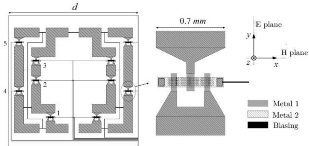
Figure 2.36 : Cellule composée de pseudo-anneaux et de MEMS permettant un déphasage sur une gamme de phase de 360° [112]
