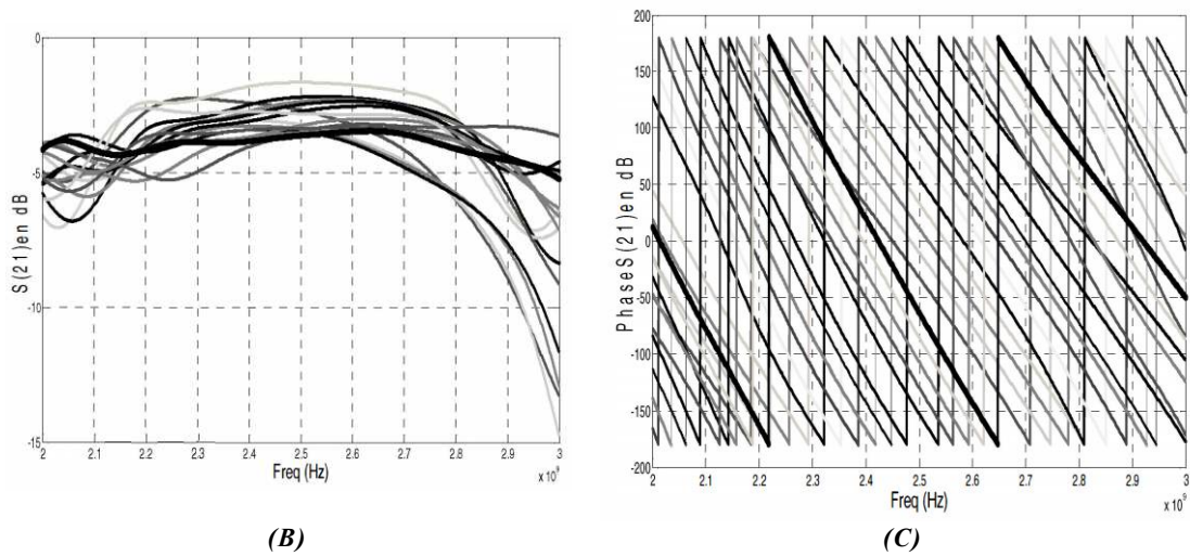
Figure 2.26 : Déphaseur 4-bits en réflexion (RTPS) à base de FET : (A) photographie, (B) pertes d'insertion et (C) phase [84]
