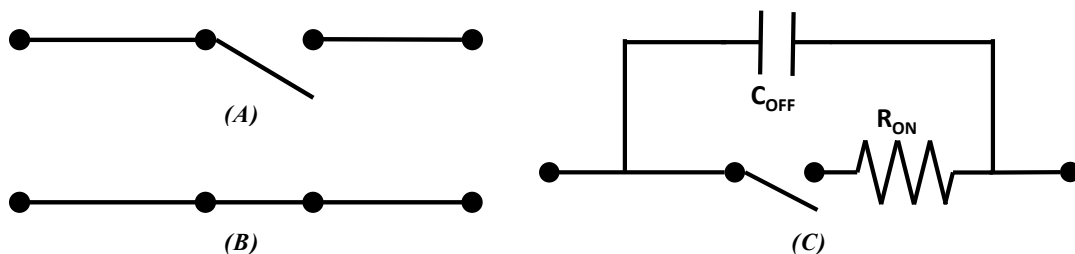
Figure 2.10 : Schéma électrique équivalent d'un commutateur idéal à l'état (A) OFF, (B) ON et (C) d'un commutateur RF réel
