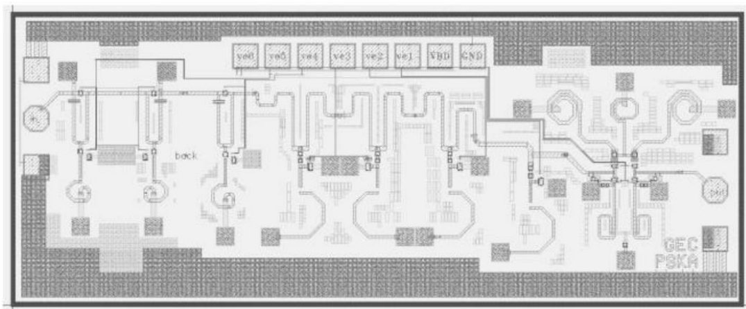
Figure 2.24 : Déphaseur 4-bits à base de FET : (A) photographie, (B) pertes d'insertion et (C) déphasage relatif [82]
