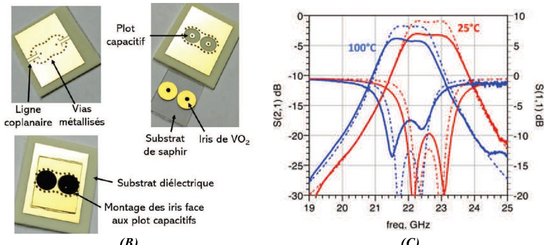
Figure 3.17 : (A) Vue de coupe et des faces supérieure et inférieure, (B) photographie et (C) performances du filtre SIW à base de commutateurs de VO 2 [54]
