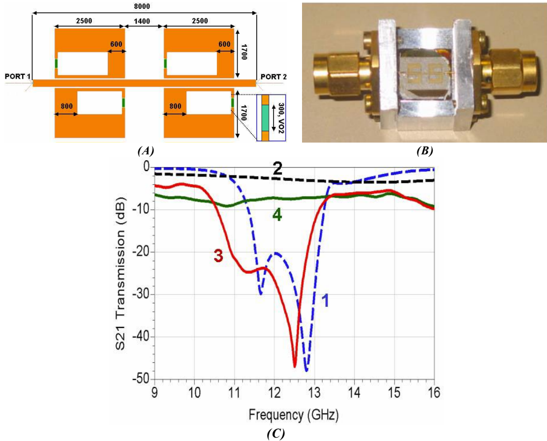
Figure 3.16 : (A) Schéma du filtre stop bande à base de VO_2 , (B) photographie du filtre réalisé et (C) sa réponse fréquentielle RF [51]
