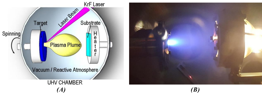
Figure 3.22 : (A) Schéma de principe de fonctionnement de l'ablation par laser impulsif (source schéma IRCER) et (B) photo du plasma généré dans la chambre de dépôt
