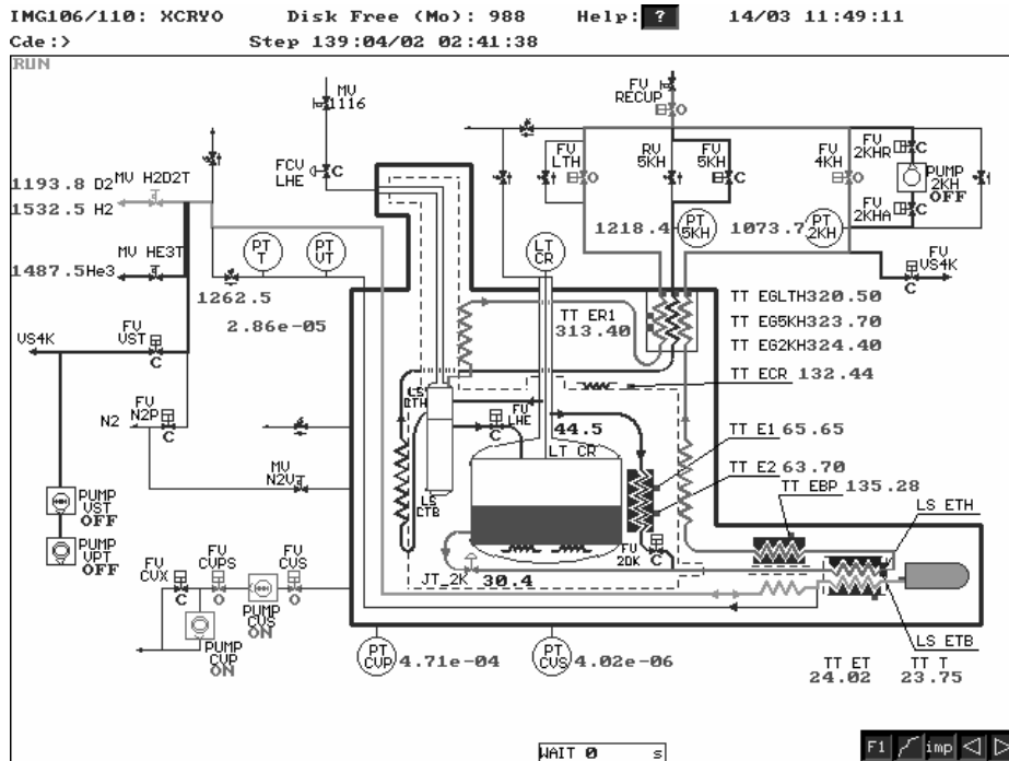
FIG. 2.20 – Schéma de l'écran de contrôle général de la cible. La température de la cible est donnée par TT_T en bas à droite.
