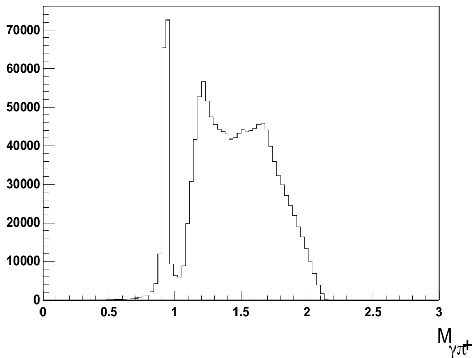
FIG. 4.14 – Masse manquante M_{\gamma\pi^+} quand le \pi^+ au moins est détecté (l'abscisse est en GeV). ( 0,48 < E_\gamma < 2,3 GeV)
