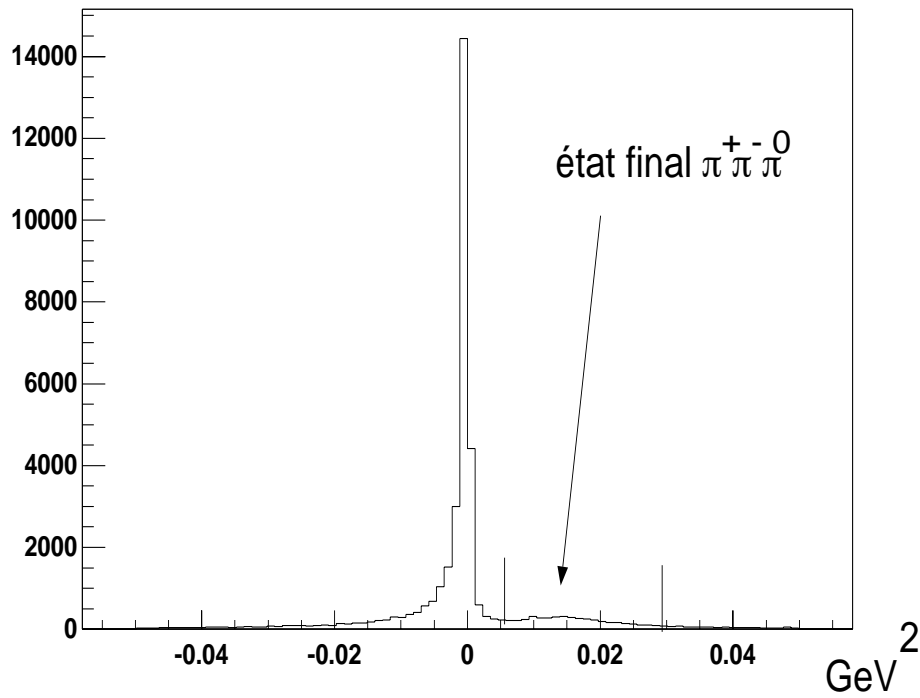
FIG. 4.18 – Masse manquante au carré M_{\gamma p \pi^+ \pi^-}^2 quand p, \pi^+, \pi^- sont détectés. Les bornes correspondent au minimum et maximum que l'on prend pour isoler un état final à trois pions.
