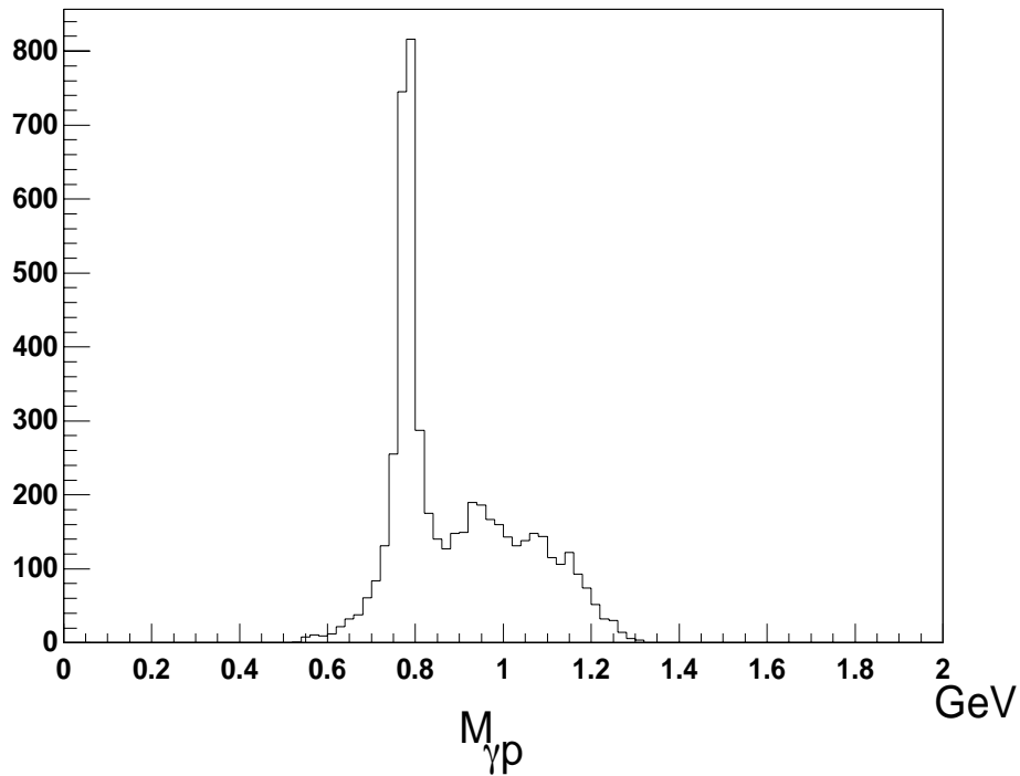
FIG. 4.19 – Masse manquante M_{\gamma p} quand p, \pi^+, \pi^- sont détectés et que la masse manquante carré M_{\gamma p \pi^+ \pi^-}^2 est celle du \pi^0 . On distingue très clairement le \omega sortir du bruit de fond. ( 0,48 < E_\gamma < 2,3 \text{ GeV} )
