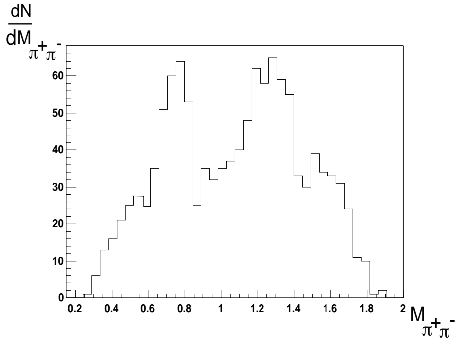
FIG. 4.24 – Masse invariante M_{\pi^+\pi^-} pour les angles arrières. Le méson tenseur f_2 apparaît très clairement à la masse 1270 \text{ MeV} . ( 3 < E_\gamma < 4 \text{ GeV} et |u| < 1 \text{ GeV}^2 )
