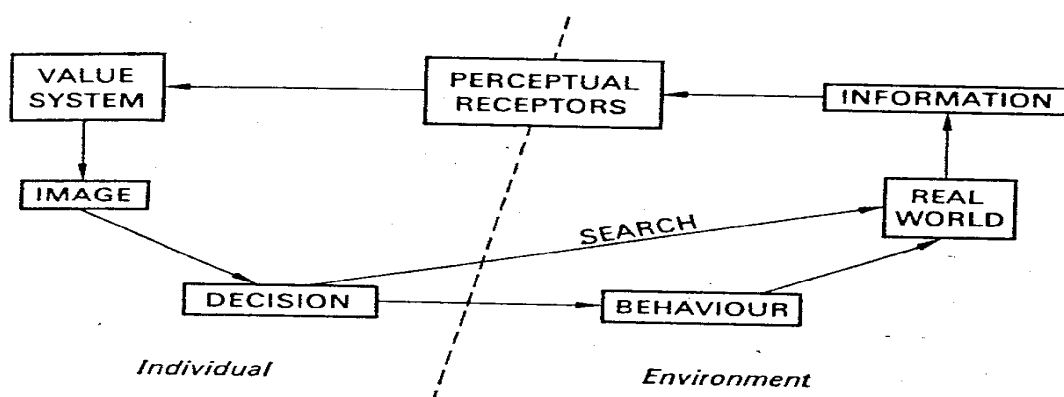
Figure n°2: Schémas des perceptions
