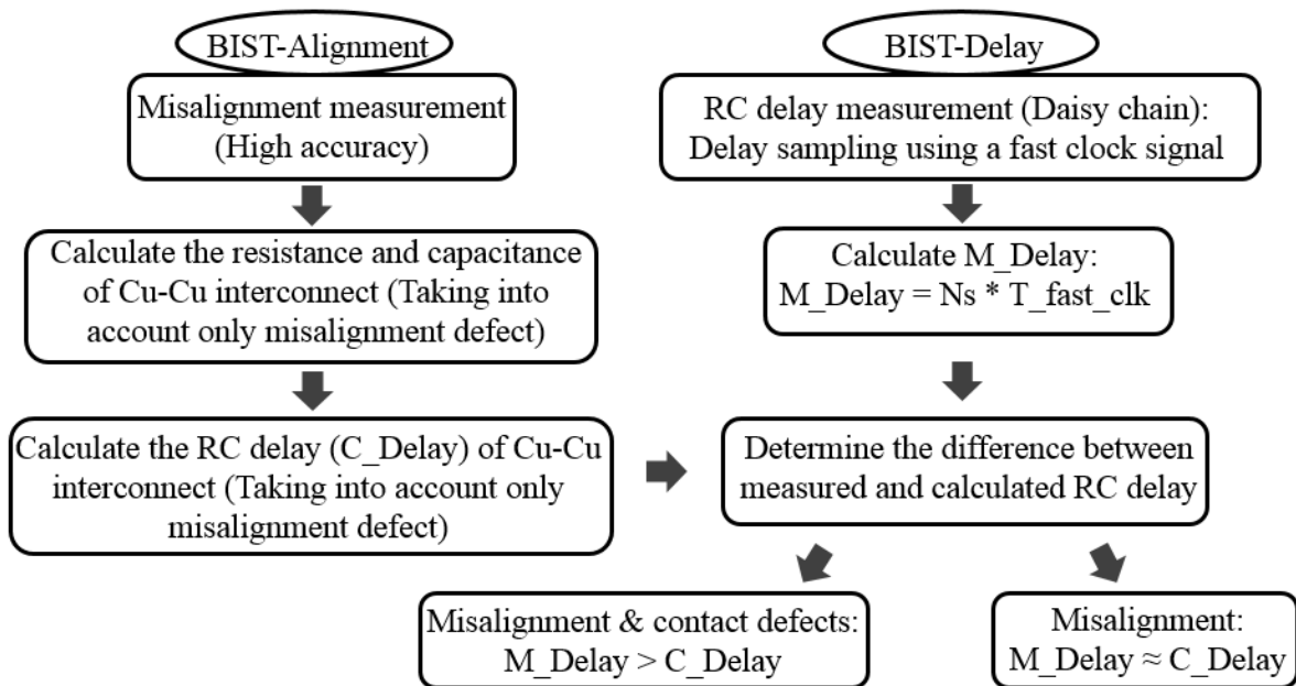
Flow de test proposé
