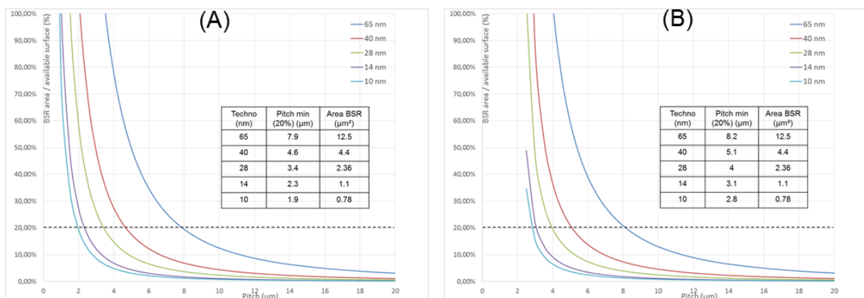
Le rapport entre la surface d'un BSR et la surface disponible en fonction du pas : (a) F2F, (b) F2B
