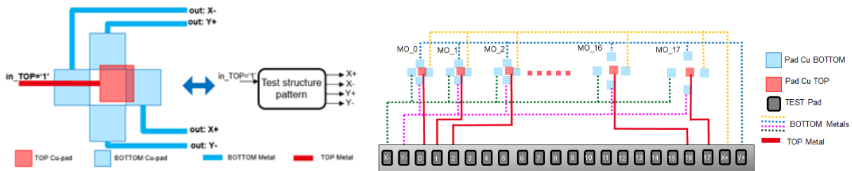
Motif pour la mesure de désalignement
