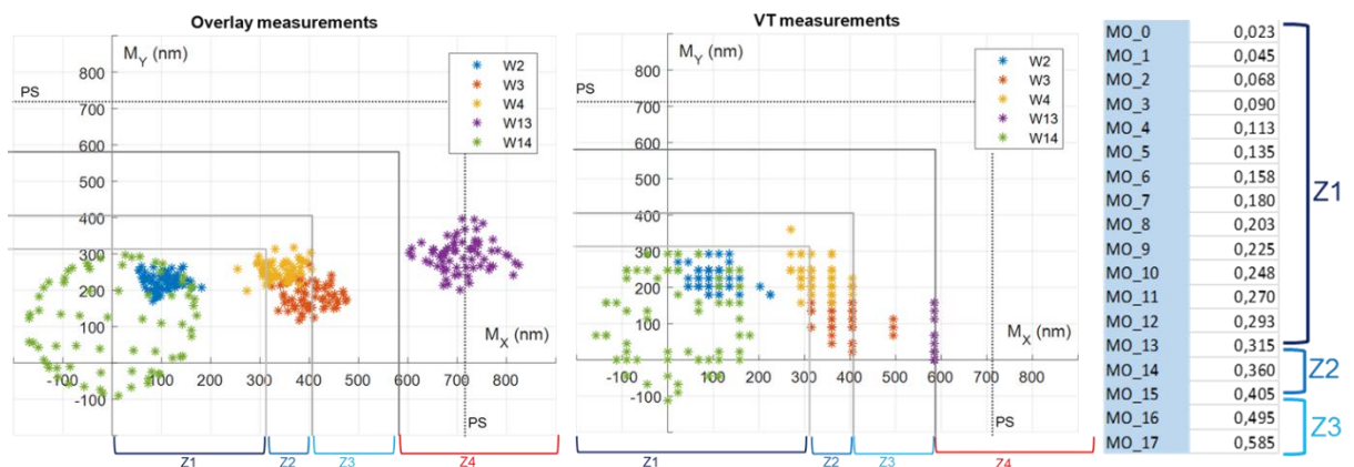
Distribution des mesures du désalignement
