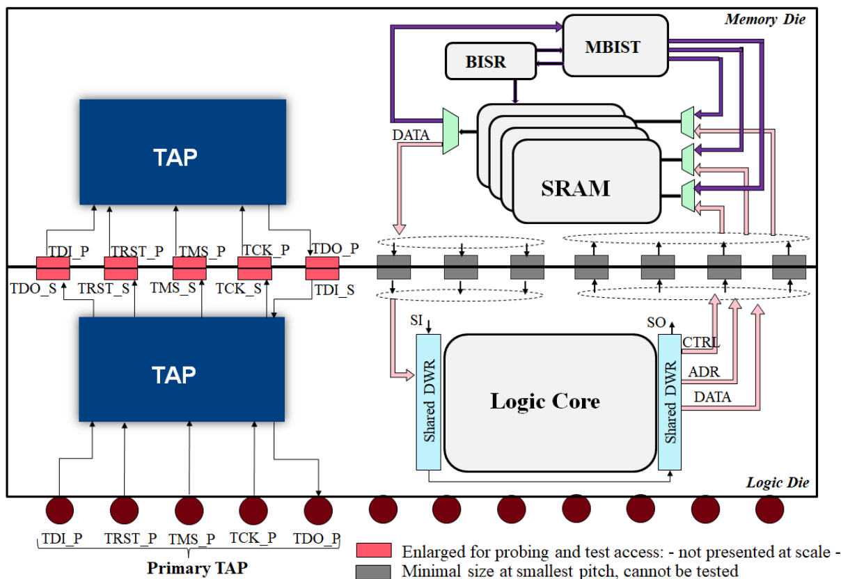
L'architecture DFT-3D proposé
