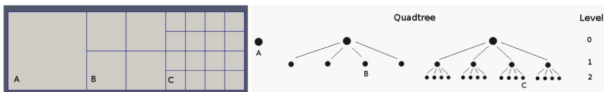
FIGURE 3.6 – Illustration d'un arbre de parenté quaternaire 2D extrait de ANTEPARA et al. [5]
