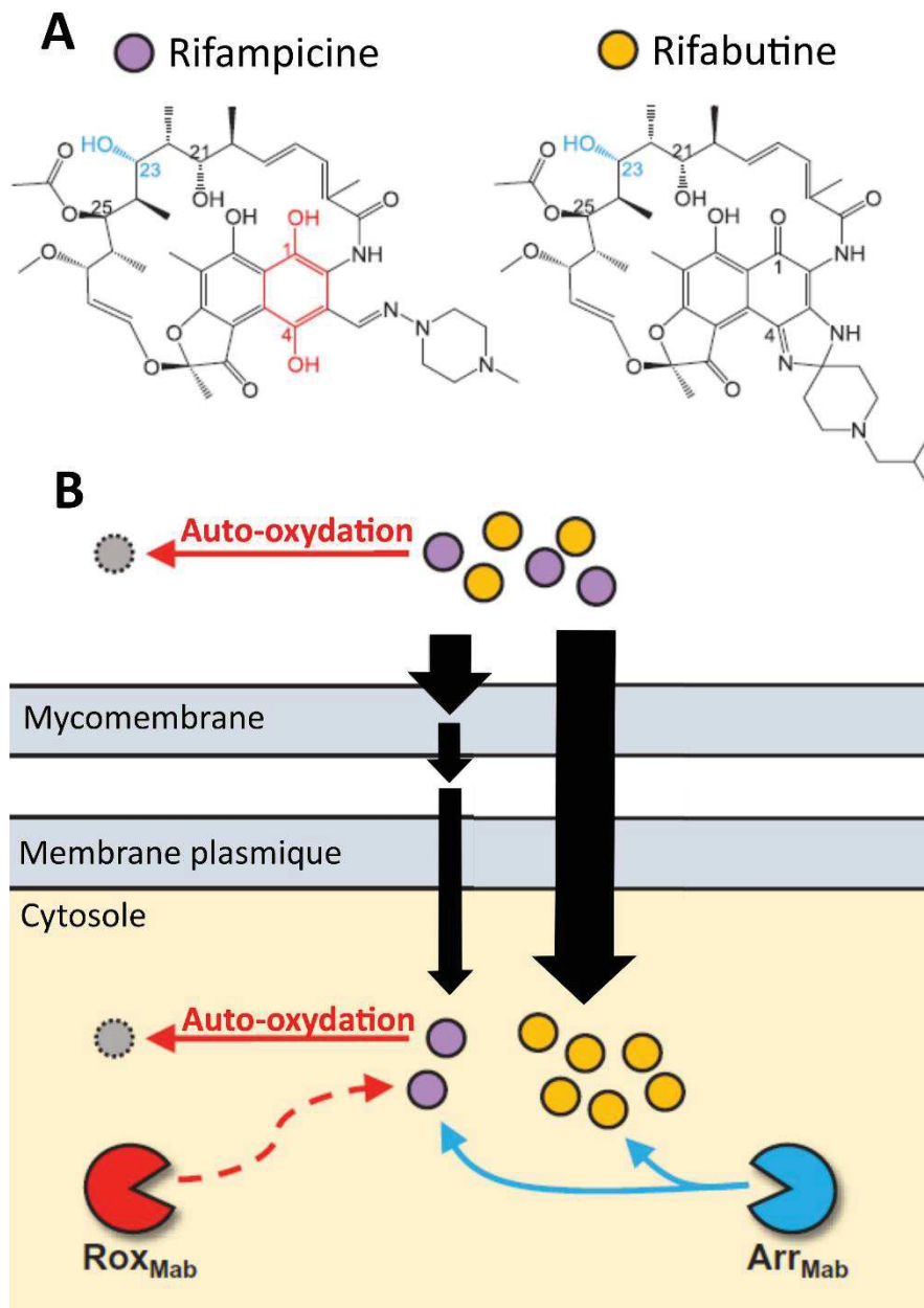
Figure 26. La rifabutine possède des propriétés structurales lui conférant une meilleure absorption ainsi qu'une meilleure résistance à l'auto-oxidation et aux dégradations enzymatiques. (A) Le C23 ADP-ribosylée modifié par Arr Mab est marqué en bleu sur les structures de la rifampicine et de la rifabutine. Le cycle naphthoquinone responsable de l'auto-oxidation et de la dégradation par Rox Mab est marqué en rouge sur la structure de la rifampicine. (B) La rifabutine pénètre de manière plus efficace la paroi mycobactérienne que la rifampicine et possède alors une meilleure pharmacocinétique. La rifabutine n'est pas sensible à l'auto-oxidation de Rox Mab mais ces deux rifamycines sont sensibles à Arr Mab (Adopté de Ganapathy et al 2019).
