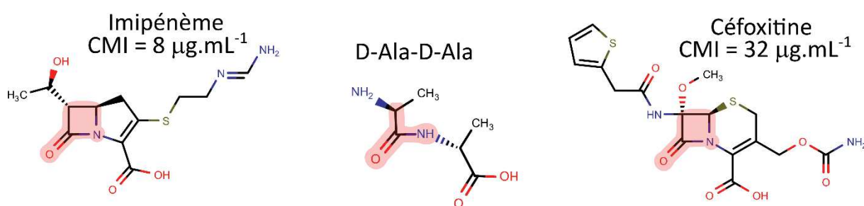
Figure 14. Structures des β-lactamines utilisées dans le traitement de M. abscessus . Le D-Ala-D-Ala, substrat des D, D-transpeptidases, est représenté au centre. La partie du substrat imitée par les β-lactamines via leurs noyaux β-lactames est encadrée en rouge pour l'imipénème (à gauche) et la céfoxitine (à droite).
