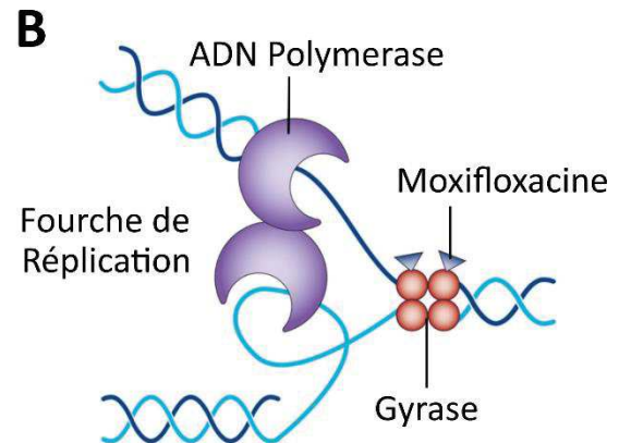
Figure 19. Structure de la moxifloxacin (A) et représentation schématique de son interaction avec l'ADN gyrase lors de la réplication de l'ADN (B). L'ADN gyrase va dénouer l'ADN en générant des coupures temporaires de la double-hélice permettant à l'ADN polymérase de répliquer le matériel génétique. La moxifloxacin va former un complexe avec l'ADN et l'ADN gyrase ce qui provoquera un arrêt de la réplication et laissera l'ADN clivé. Ces cassures de l'ADN généreront un fort stress oxydatif déclenchant la mort cellulaire (Adapté de Kohanski et al. 2010).
