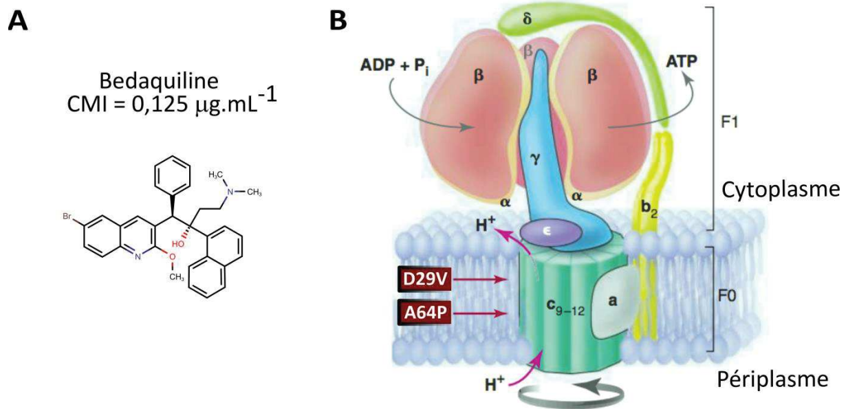
Figure 23. Structure de la bédaquiline (A) et représentation schématique de sa cible, l'ATP synthase (B). L'ATP synthase est constituée d'une partie cytoplasmique F_1 et d'une partie transmembranaire F_0 . Les sous-unités c sont arrangées en disques symétriques capables de rentrer en rotation grâce à la force proto-motrice, qui est nécessaire par la suite pour la synthèse d'ATP. Les mutations D29V et A64P confèrent à M. abscessus de hauts niveaux de résistance (Adapté de Cole et Alzari 2005).
