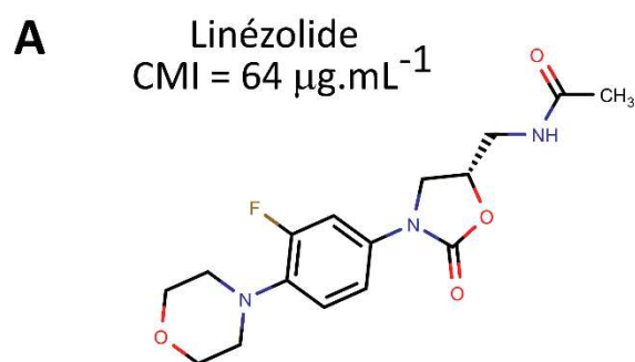
Figure 20. Structure du linézolide (A) et du tédzolide (B)
