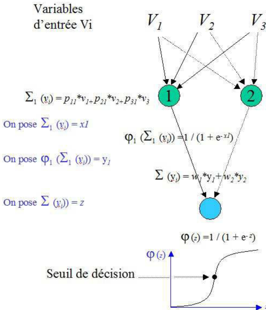
Figure 12 : Description d'un réseau de neurones simplifié présentant une couche d'entrée à 2 neurones et une couche de sortie à 1 neurone
