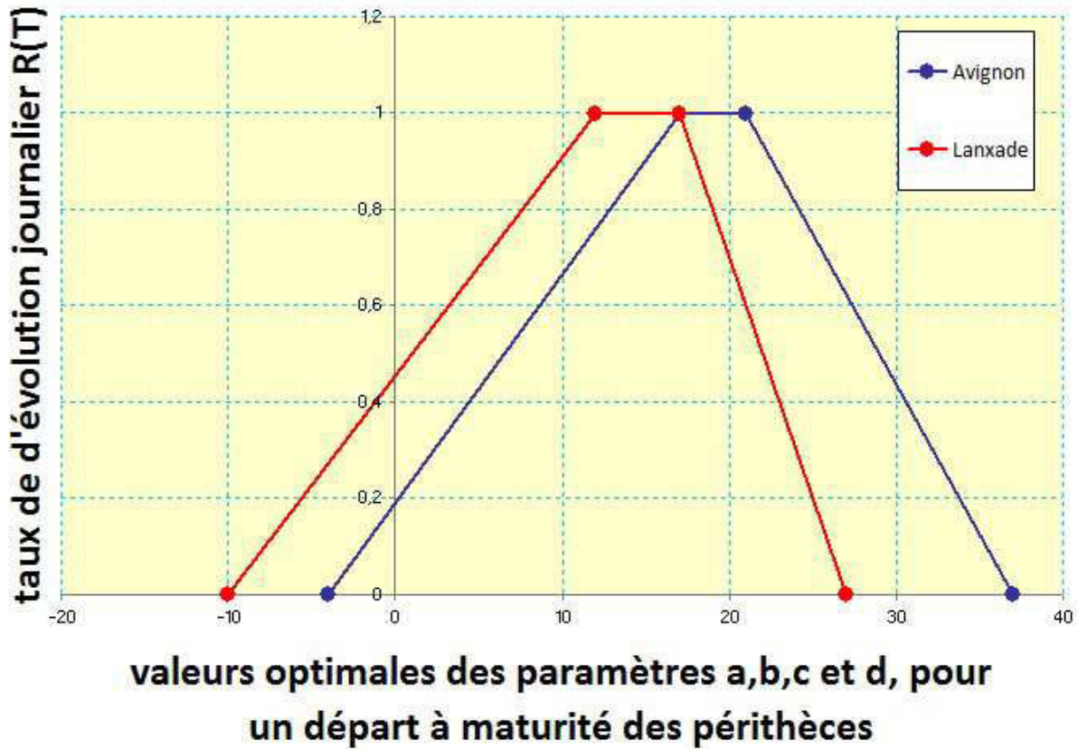
Figure 22 : Fonctions comparées du taux d'évolution journalier de l'inoculum primaire de la tavelure du pommier, établies à maturité des pseudothèces par optimisation numérique pour deux localités, Avignon et Lanxade
