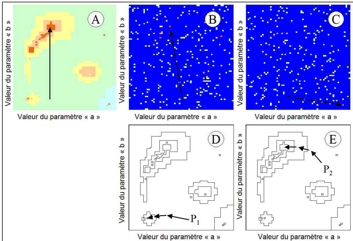
Figure 19 : Représentation graphique d'une fonction critère hypothétique \rho pour l'optimisation de deux paramètres a et b et exemples de résultats produits lors d'optimisation (A) par recherche systématique sur grille (100 valeurs de a en abscisse et 100 valeurs de b en ordonnée ; les couleurs les plus chaudes correspondent aux valeurs les plus élevées de la fonction critère ; la flèche indique un choix empirique de l'optimum) ; (B) et (C) par tirage aléatoire (deux exemples de tirages au sort de 500 paires (a,b) ; les flèches indiquent l'optimum obtenu) ; (D) et (E) par descente de gradient (deux exemples partant de points d'initialisation P_1 et P_2 différents ; les flèches indiquent les étapes itératives de l'optimisation).
