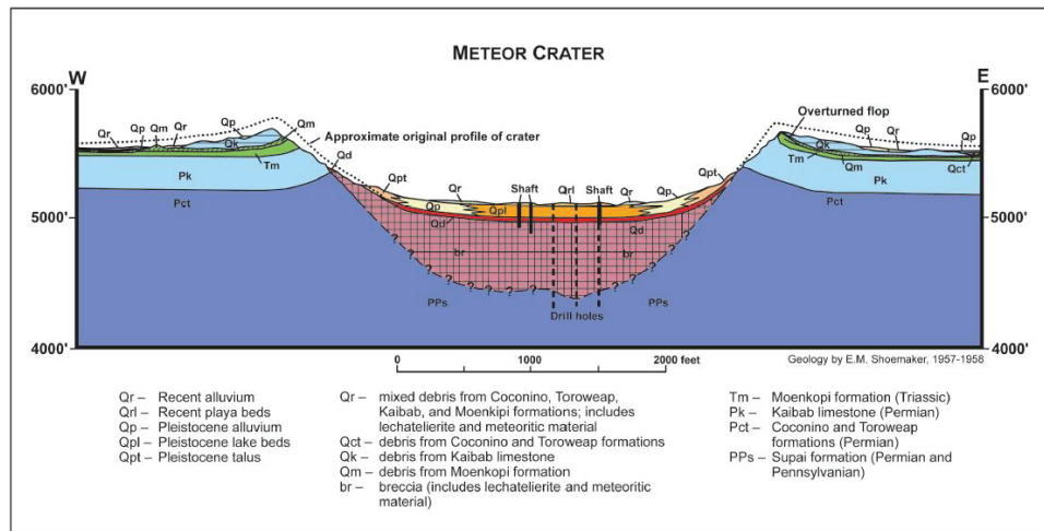
Figure 1.28: Coupe de Meteor crater, Arizona, Etats-Unis, à partir de Kring (2007).
