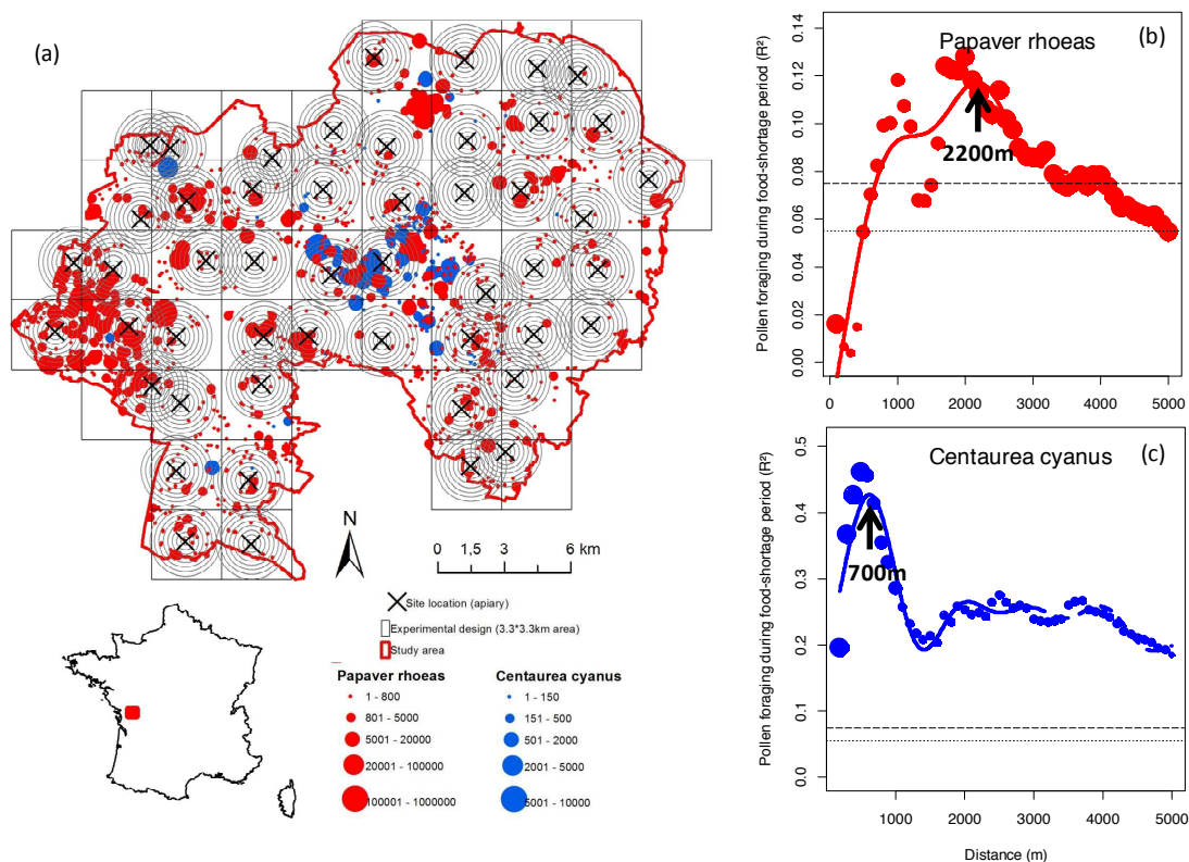
Figure 2 : Sélection des ressources par l'abeille domestique selon un compromis distance-quantité, (a) distribution spatiale des ressources coquelicot et bleuet, résultats des corrélations récolté-disponible par pats de distance pour (b) le coquelicot et (c) le bleuet. Les lignes horizontales renseignent les seuils de significativité des corrélations, ---<0.05, ...<0.1. Chaque point résulte du R^2 de la corrélation entre le nombre de patches disponibles (transformé en \log_{10} ) et la biomasse de pollen maximale collectée (transformé en \log_{10} ) par pat de distance, n=50 . La taille des points renseigne sur la valeur de la pente de corrélation (toutes positives, variant de 0.13 à 0.83). Le patron du corrélogramme de distance est représenté par un GAM, n=50 .
