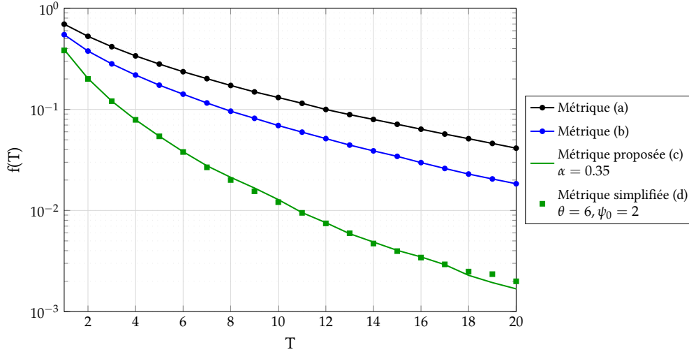
FIGURE 3.8: Comparisons des métriques pour (N,K) = (1024,512) avec SNR= 2.0dB
