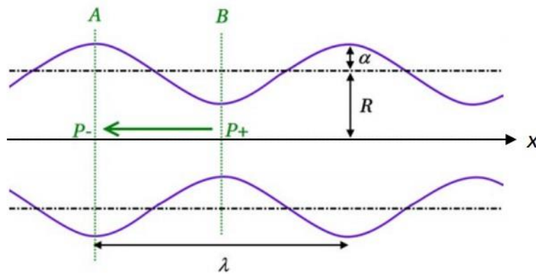
Figure II. 14 : Perturbation de longueur d'onde \lambda et d'amplitude \alpha à la surface d'un jet cylindrique de rayon R . La flèche verte représente l'écoulement généré par le gradient de pression. 85
