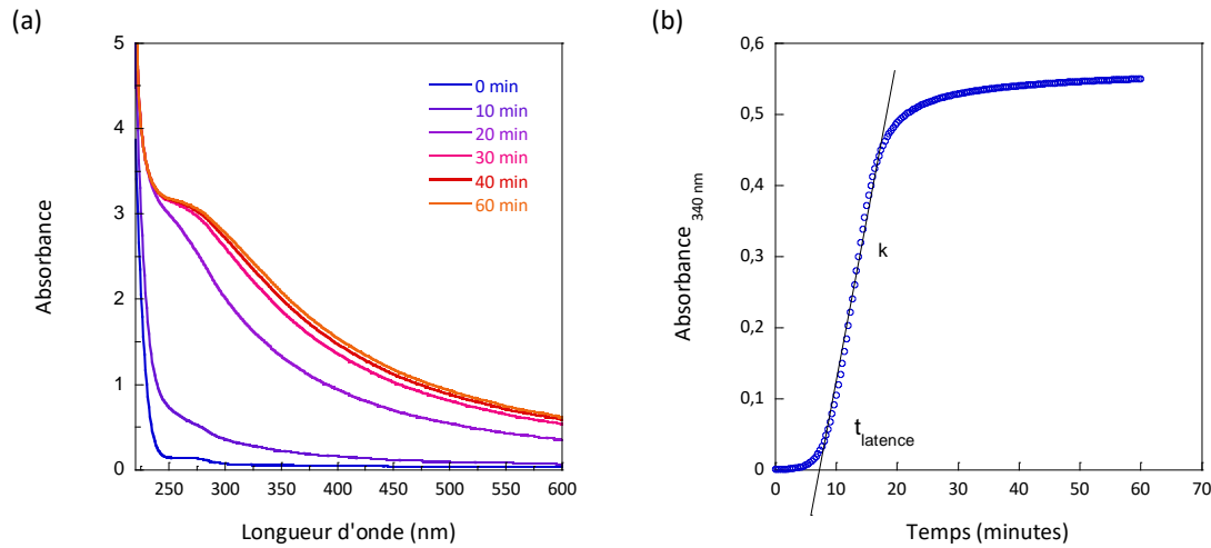
Figure II. 19 : (a) Spectres d'absorption d'une solution de collagène. Conditions : 1\text{mg.mL}^{-1} , pH neutre et à 20^\circ\text{C} . (b) Une Courbe sigmoïdale caractérise l'agrégation du collagène. Conditions : 2\text{mg.mL}^{-1} , pH neutre et à 20^\circ\text{C}
