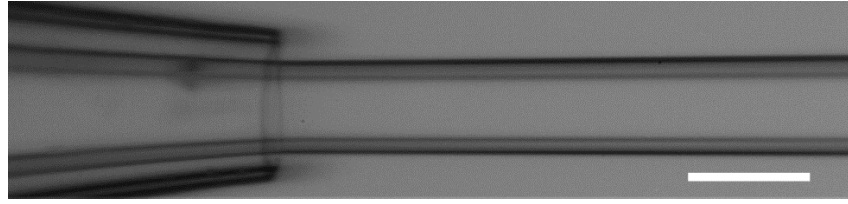
Figure II. 9 : Co-écoulement concentrique des fluides. Cœur et coque : eau ; Intermédiaire : solution de glycérol à 60 %m. Q_{tot} = 300 \text{ mL.h}^{-1} ; R_q = 2 ; r_q = 1 . La barre d'échelle correspond à 200 \mu\text{m} .
