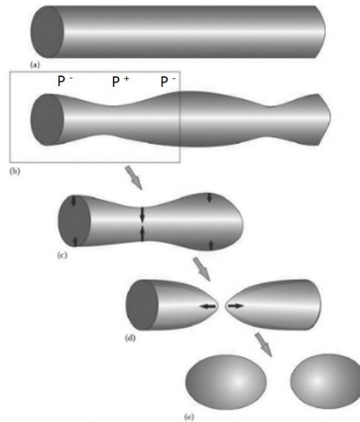
Figure 1. 4 : Mécanisme physique de l'instabilité de Rayleigh-Plateau. Jet cylindrique (a) est soumis à des perturbations externes de pression qui le déforme (b). Les déformations en surface sont amplifiées par les effets de la pression de Laplace (c) jusqu'à ce que le jet se fragmente (d) en des gouttes de forme sphérique (e).
