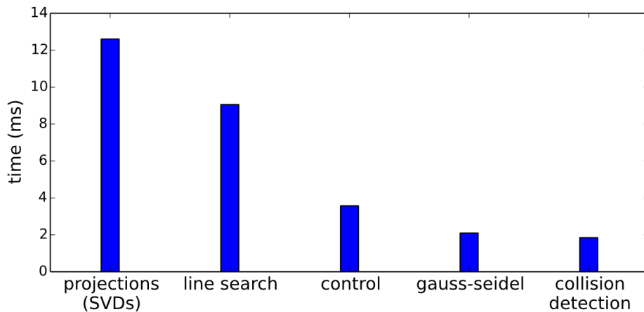
FIGURE 12 – Répartition des temps de calcul sur un pas de temps impliquant 50 contraintes de collision et 110 contraintes de lèvres collantes.
