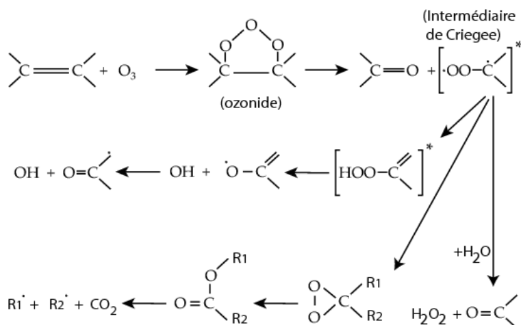
Figure 2.8 – Mécanisme d'oxydation gazeuse d'un composé organique insaturé par l'ozone (d'après Valorso, 2011).
