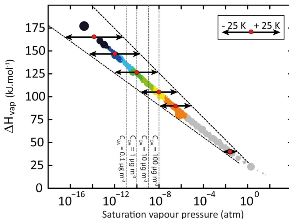
Figure 2.14 - Influence de la température sur la volatilité et le partage gaz/particules des composés organiques secondaires, exemple des produits de l'oxydation de l'octadécane selon une étude de modélisation avec GECKO-A. Les bulles représentent la distribution des espèces en terme de volatilité ( P_i^{sat} ) et d'enthalpie de vaporisation ( \Delta H_{vap,i} ), toutes deux estimées selon Nannoolal et al. (2004 et 2008). En pointillés gris sont représentées les droites d'équi-répartition 50-50 entre les phases gazeuse (à droite) et aérosol (à gauche) pour quatre valeurs de C_{OA} . L'effet d'une variation de \pm 25 \text{ K} sur la P_i^{sat} est présenté par des flèches pour 6 espèces (points rouges) de \Delta H_{vap,i} égales à 40, 90, 105, 125, 145 et 165 \text{ kJ.mol}^{-1} .
