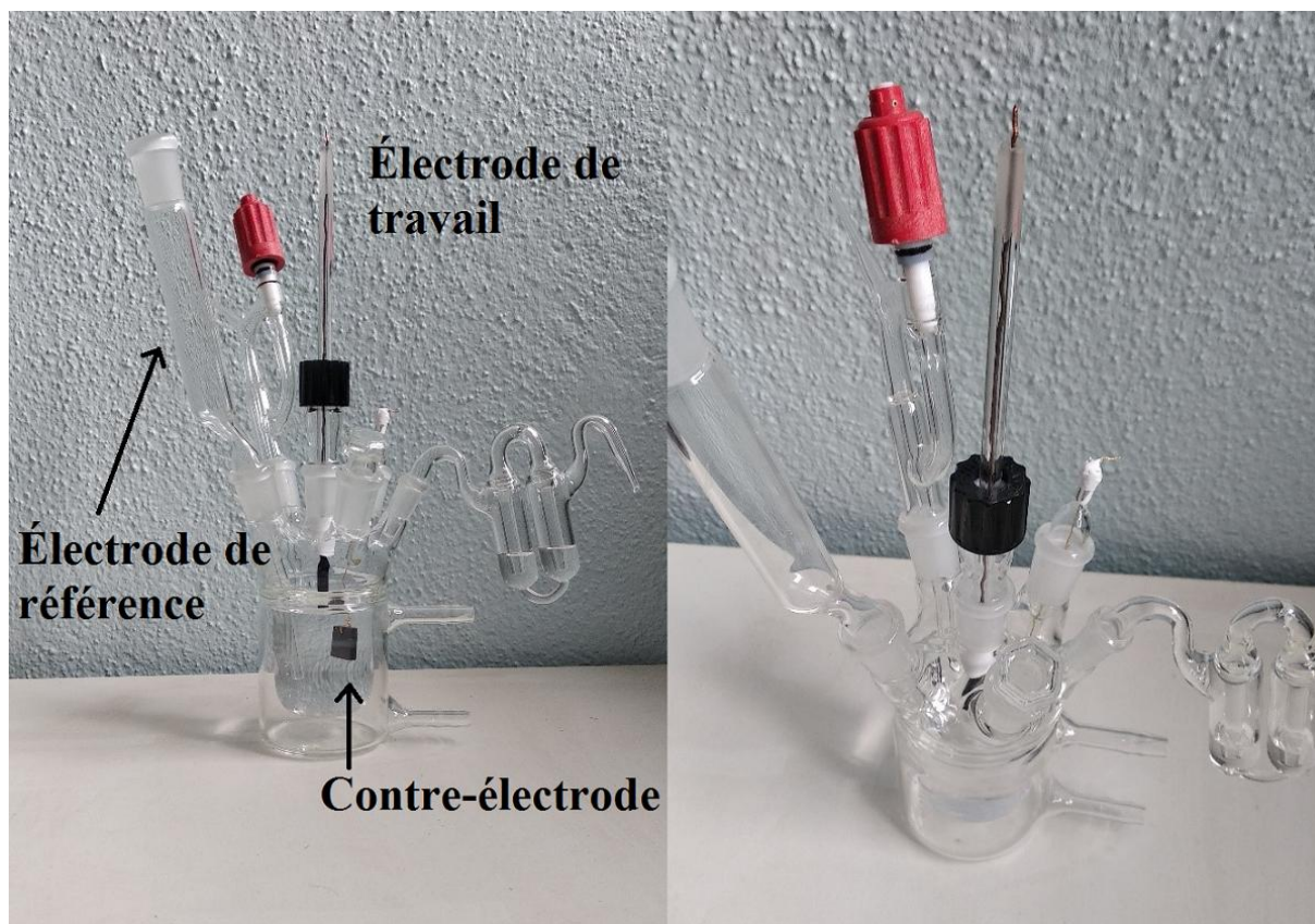
Figure II.1 : Photographies de la cellule électrochimique.
