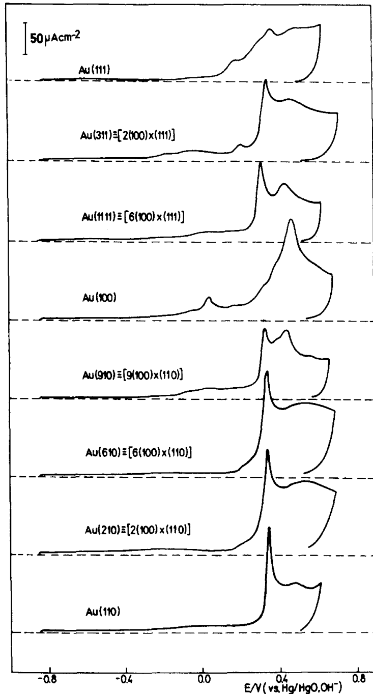
Figure I.7 : Voltammogrammes d'électrodes monocristallines d'or de différents indices de Miller en milieu 0,1 \text{ mol.L}^{-1} \text{ NaOH} et à 50 \text{ mV.s}^{-1} . Reproduit de la référence [57].
