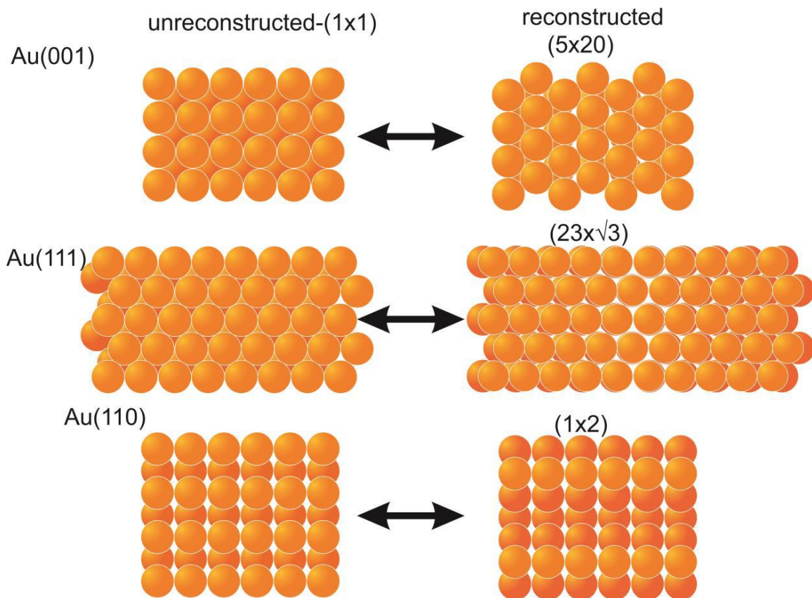
Figure I.5 : Représentation schématique des surfaces de l'or monocristallines de bas indices et de leurs reconstructions.
