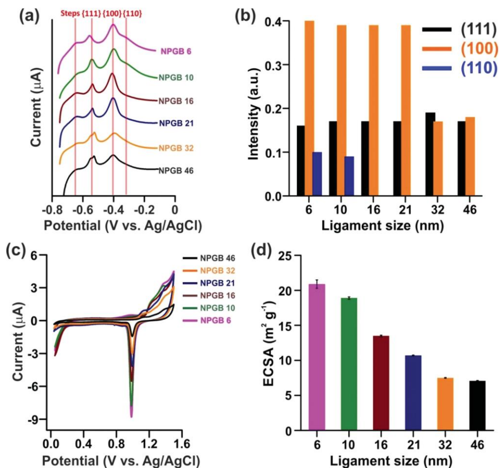
Figure I.11 : Caractérisations électrochimiques de nanostructures poreuses d'or avec des tailles de ligaments variées : a) étape de désorption du plomb : voltammétrie cyclique des électrodes d'or en milieu 0,1 \text{ mol.L}^{-1} \text{ NaOH} + 1 \text{ mmol.L}^{-1} \text{ Pb(NO}_3)_2 enregistrés à 5 \text{ mV.s}^{-1} ; b) intensités relatives des faces ; c) voltammogrammes des électrodes d'or nanoporeux en milieu 0,5 \text{ mol.L}^{-1} \text{ H}_2\text{SO}_4 enregistrés à 5 \text{ mVs}^{-1} ; d) Surfaces spécifiques actives calculées (EASA). Reproduit de la référence [162].
