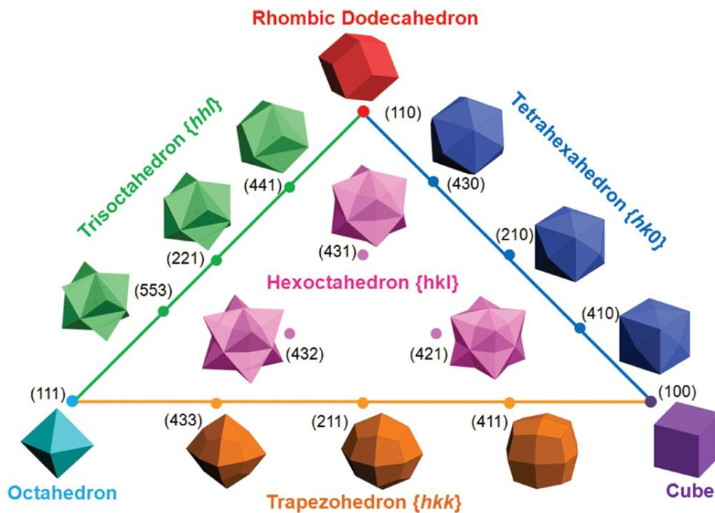
Figure I.9 : Triangle stéréographique représentant les nanocristaux. Reproduit de la référence [89].
