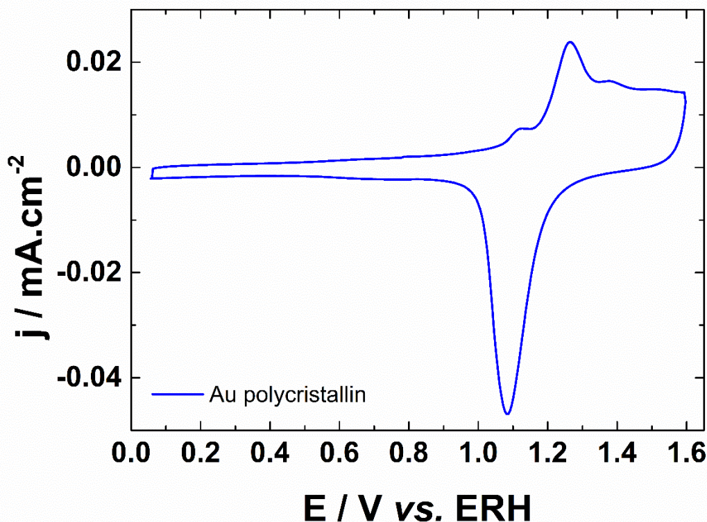
Figure II.3 : Voltammogramme d'une électrode d'or polycristalline en milieu 0,1 \text{ mol.L}^{-1} NaOH enregistré à 20 \text{ mV} \cdot \text{s}^{-1} à une température de 20 \text{ }^\circ\text{C} .
