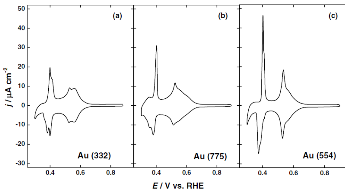
Figure I.8 : Voltammogrammes de monocristaux d’or de différents indices de Miller en milieu 0,05 \text{ mol.L}^{-1} \text{ H}_2\text{SO}_4 + 1 \text{ mmol.L}^{-1} \text{ CuSO}_4 enregistrés à 5 \text{ mV.s}^{-1} . Reproduit de la référence [63].
