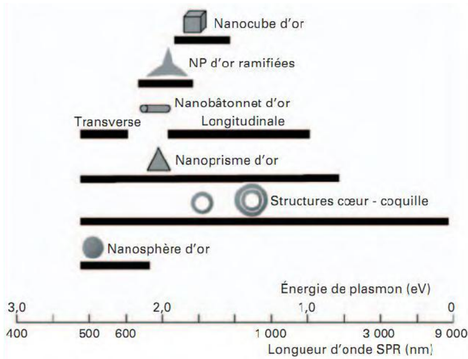
Figure I.3 : Gammes des longueurs d'onde et énergies de résonance plasmon pour différentes morphologies et structures de nanoparticules d'or. Reproduit de la référence [33].
