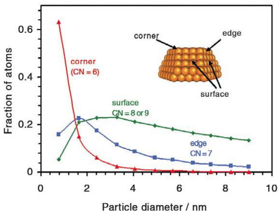
Figure I.12 : Fractions calculées d'atomes de coins, d'arêtes et des faces cristallines dans un modèle de particule (moitié d'un octaèdre tronqué) en fonction du diamètre de la particule. L'insert montre l'octaèdre tronqué ainsi que les différents atomes. Reproduit de la référence [30].
