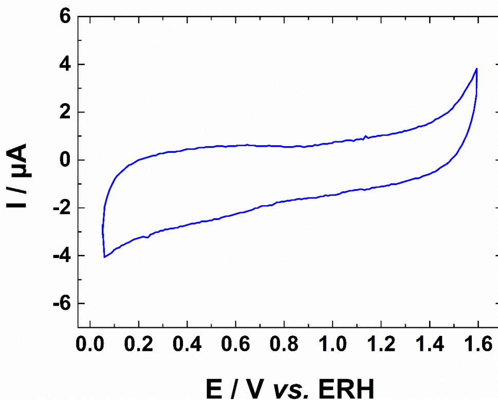
Figure II.2 : Voltammogramme du carbone vitreux en milieu 0,1 \text{ mol.L}^{-1} \text{ NaOH} enregistré à 50 \text{ mV.s}^{-1} à une température contrôlée de 20 \text{ }^\circ\text{C} .
