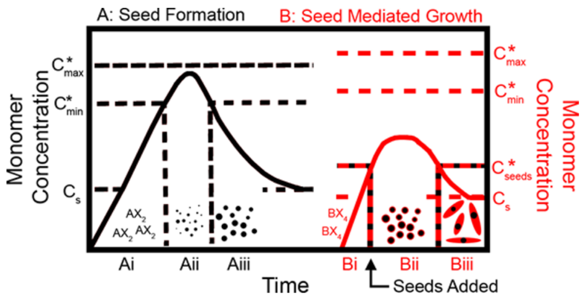
Figure I.16 : a) Modèle de LaMer pour la formation de nanoparticules utilisées comme germes. Avec C_s : niveau de solubilité, C_{min} : concentration minimum de monomère pour démarrer la nucléation, C_{max} : concentration maximum de monomère, A_i : étape de pré-nucléation, A_{ii} : étape de nucléation, A_{iii} : étape de croissance du germe ; b) extension du modèle de LaMer à la croissance par les germes. Avec C_{seeds} : concentration minimum de monomère pour démarrer la nucléation sur le germe, B_i : étape de pré-nucléation, B_{ii} : étape de nucléation sur le germe, B_{iii} : étape de croissance. Reproduit de la référence [263].
