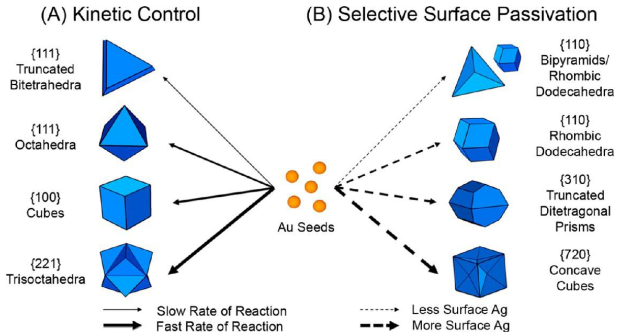
Figure I.18 : Schéma représentant le type de géométrie qu'il est possible d'obtenir selon le contrôle cinétique ou la passivation sélective de surface. Reproduit de la référence [266].
