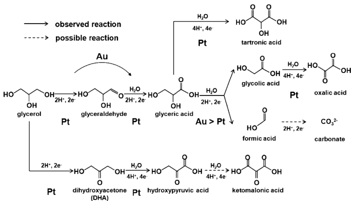
Figure I.14 : Mécanisme d'oxydation du glycérol sur Au et Pt en milieu alcalin. Reproduit de la référence [238].
