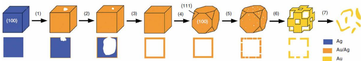
Figure I.19 : Illustration résumant comment évoluent des nanocubes d'argent lorsque la quantité de HAuCl_4 augmente. Les principales étapes : 1) initiation de la réaction de remplacement aux sites de plus haute énergie, 2) remplacement de Ag par HAuCl_4 pour former une structure partiellement creuse, 3) formation de « nanobox » avec une coquille Au–Ag, 4) initiation du dés-alliage et de la reconstruction des coins et 5–6) dés-alliage et formation d'une nanocage d'or comportant des pores. Reproduit de la référence [282].
