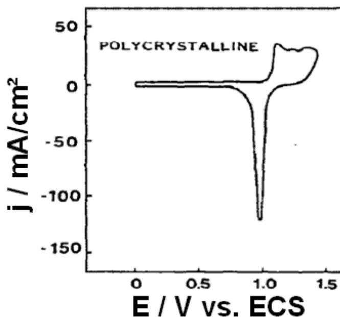
Figure I.6 : Voltammogramme cyclique de l'or polycristallin en milieu 1 mol.L -1 HClO 4 , enregistré à 20 mV.s -1 . Adapté à partir de la référence [55].
