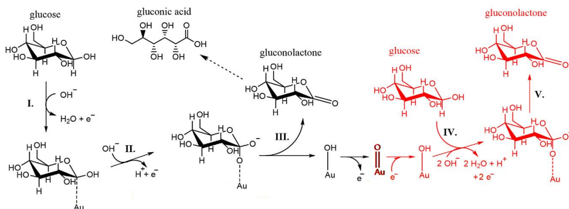
Figure I.13 : Mécanisme d'oxydation électrochimique du glucose en milieu alcalin sur une électrode d'or. Adapté de la référence [194].
