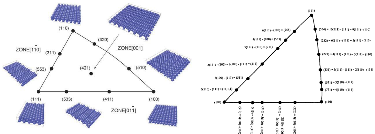
Figure I.4 : a) Triangle stéréographique avec la représentation schématique de l'empilement atomique de différentes surfaces ; b) Triangle stéréographique avec les notations TLK des hauts indices. Reproduit des figures [38] et [39].
