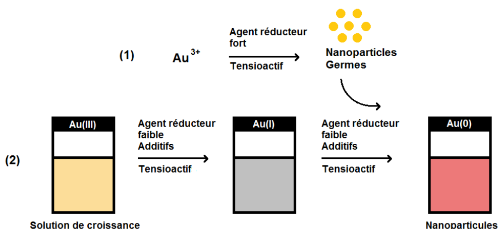
Figure I.17 : Schéma de la synthèse par la méthode de croissance par les germes.
