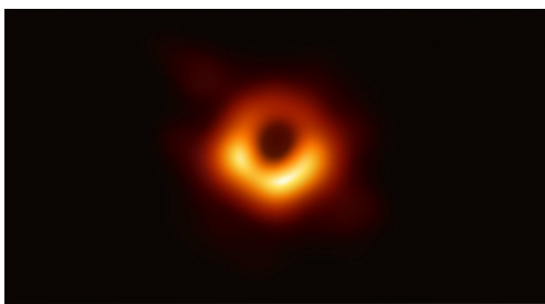
Image 29: le trou noir supermassif du centre de la galaxie M87, observé par le réseau EHT (Event Horizon Telescope), 2019.
